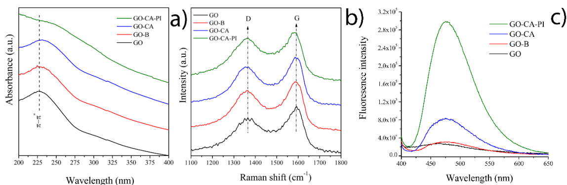
Figure 3.1 Caractérisation des échantillons GO, GO-B, GO-CA et GO-CA-PI par : a) spectroscopie UV, b) spectroscopie Raman et c) spectrométrie de fluorescence ( \lambda_{\text{ex}} = 390 \text{ nm} ).
