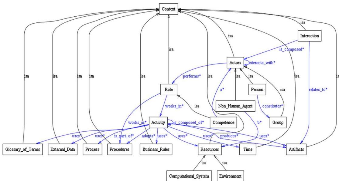
Figure 12: Modèle des données contextuelles proposé par Da Cunha Mattos et al. [138]
