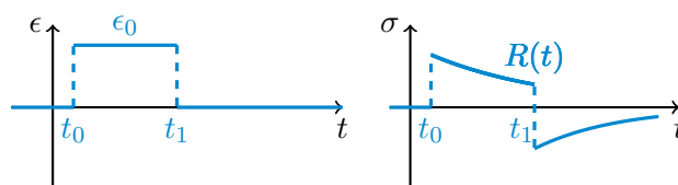
FIGURE 2.2 – Essai de relaxation avec recouvrement.
