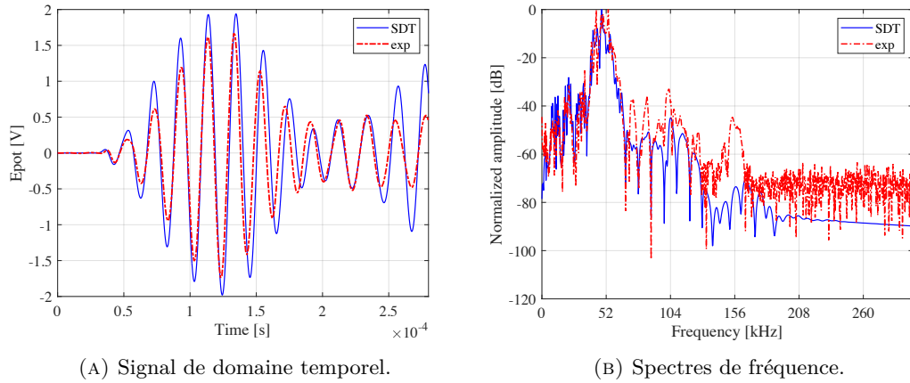
FIGURE A.16: Comparaison de la sortie électrique dans les domaines temporel et fréquentiel entre les résultats de la simulation et de l'expérience pour la plaque non endommagée. Les signaux de fréquence sont normalisés à la valeur maximale de chaque spectre respectivement.
