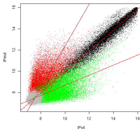
FIG. 5.15: Graphe obtenu avec le modèle sous contraintes de colinéarité avec une variance résiduelle différente et avec six composants par groupe ( 1666-\sigma_1^2\sigma_2^2 ), après classification par la règle du MAP. Le groupe bruit est en gris, le groupe identique est en noir, le groupe appauvri est en vert et le groupe enrichi est en rouge.
