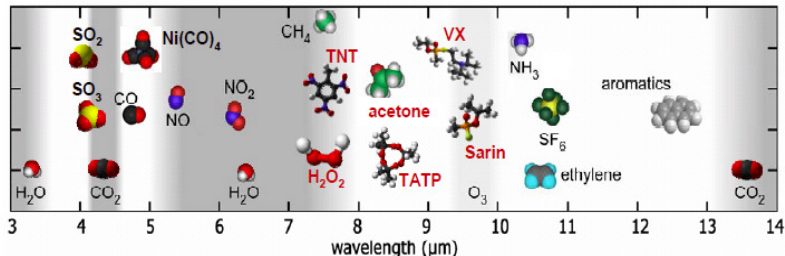
Figure 7.2: Longueur d'onde d'absorption de quelques molécules d'intérêt.
