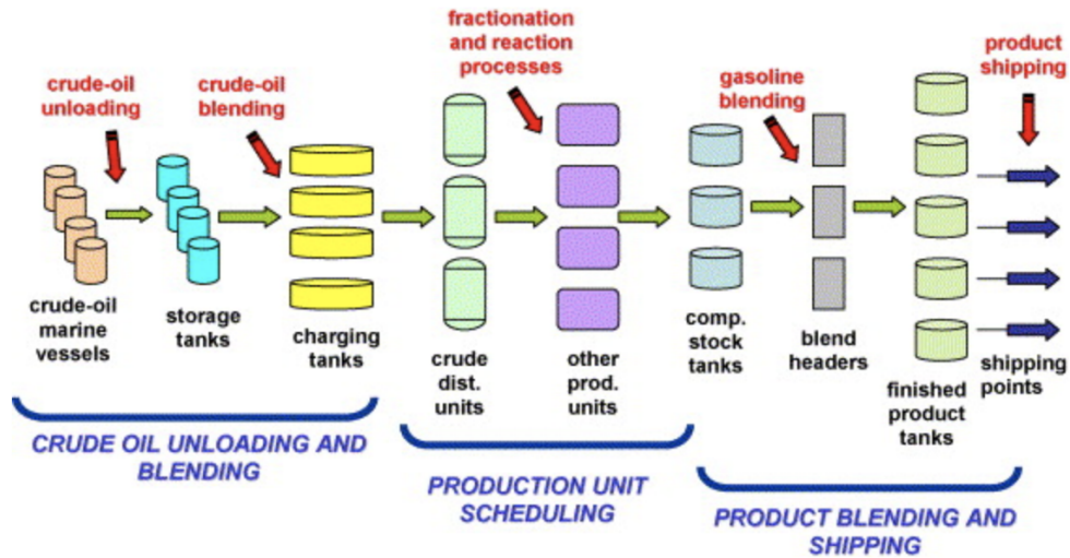
Figure 2.5: Représentation schématique des différentes étapes de raffinage
