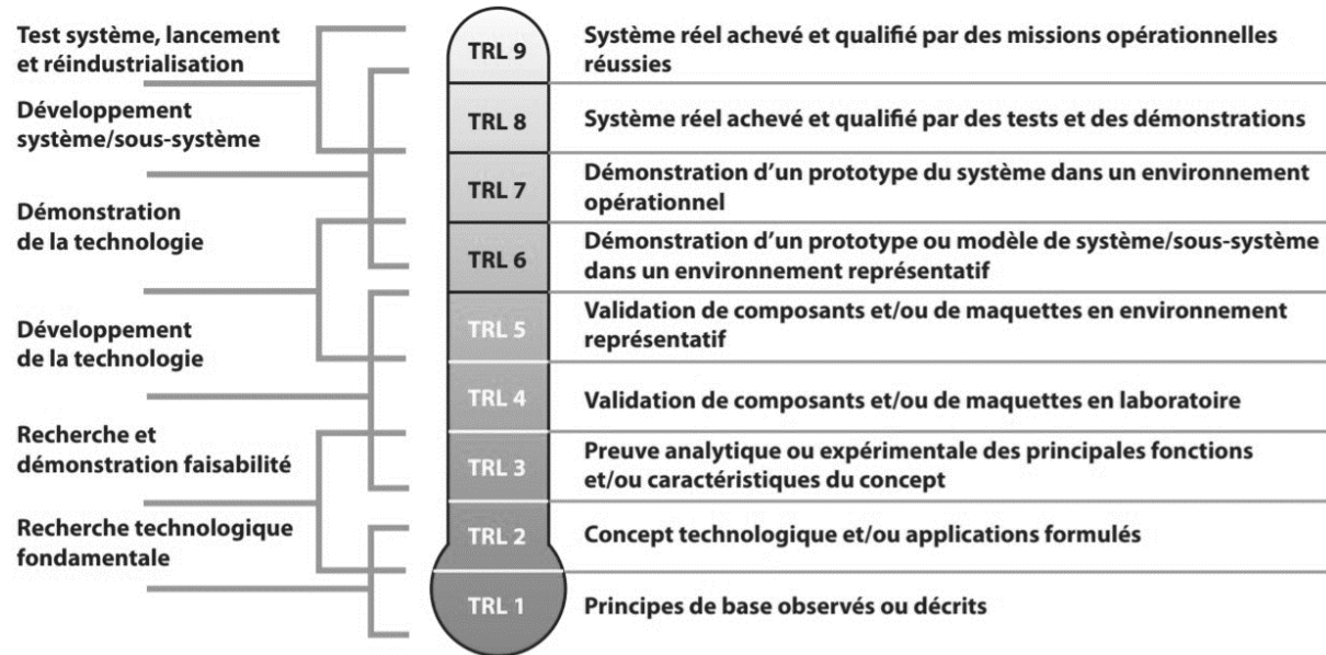
Figure 5 : Échelle TRL (DGA, 2009, p. 299)
