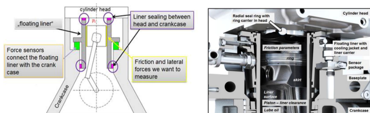
Figure 1-67 : Représentation schématique et réel d'un essai « cylindre flottant » permettant de mesurer les frottements du piston sur le cylindre [Vaitkunaite et al., 2022]
