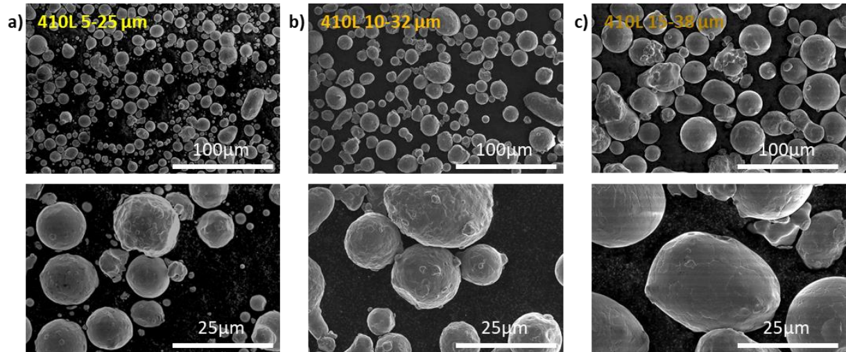
Figure 3-3 : Observations MEB en électrons secondaires des poudres d'acier 410L. Sur chaque ligne, de haut en bas, les grossissements \times 500 et \times 2000 . Sur chaque colonne une granulométrie : a) 5-25 \mu\text{m} , b) 10-32 \mu\text{m} , et c) 15-38 \mu\text{m} .
