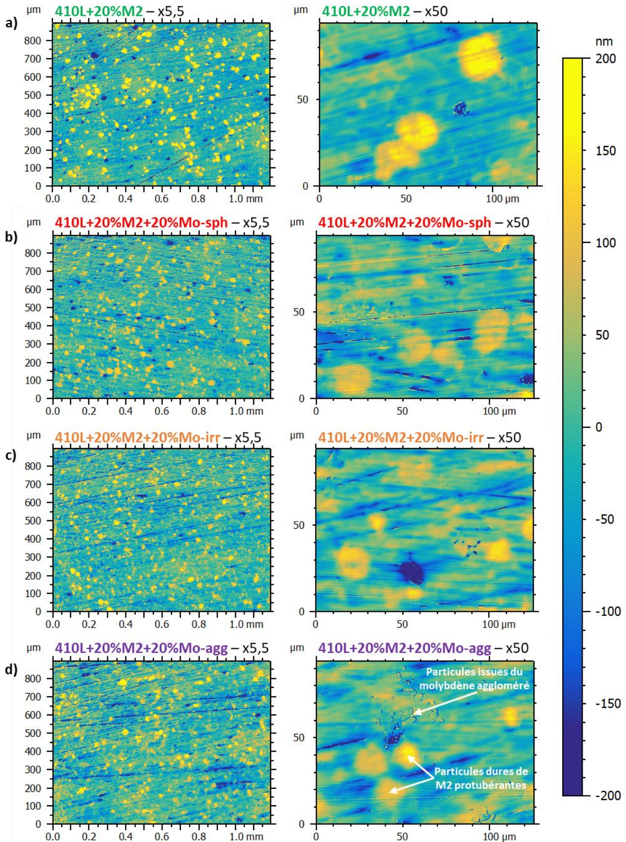
Figure 7-6 : Analyses topographiques faites par WLI avec, à gauche, le grossissement x5,5 et, à droite, le grossissement x50 des revêtements avec et sans les différentes poudres de molybdène : a) 410L+20%M2, b) 410L+20%M2+20%Mo-sph, c) 410L+20%M2+20%Mo-irr, d) 410L+20%M2+20%Mo-agg.
