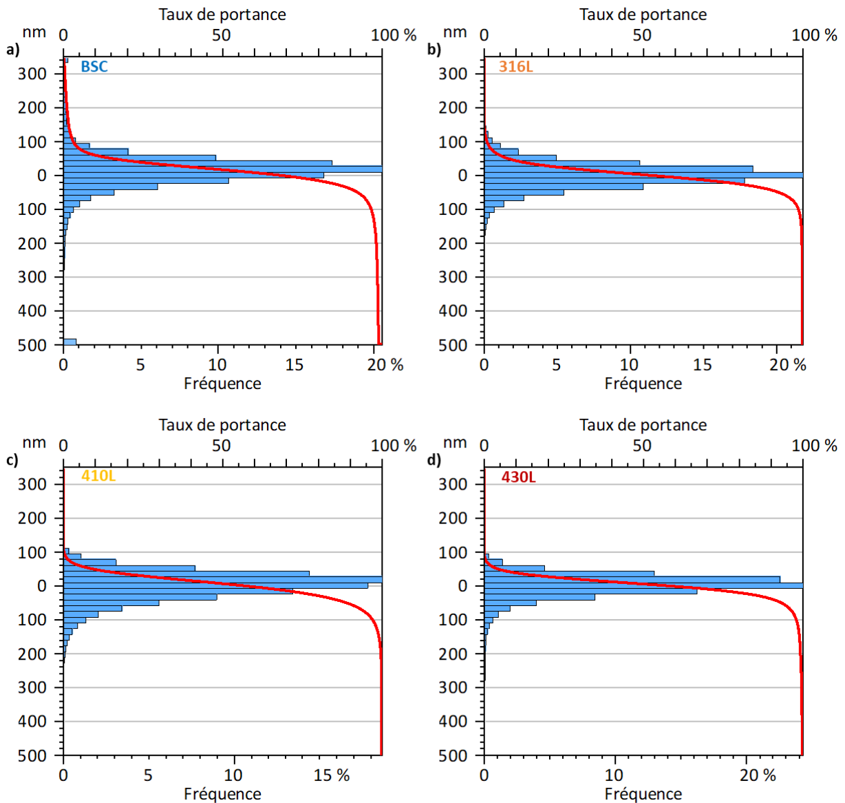
Figure 4-2 : Histogrammes des distributions de hauteurs issues du cliché WLI au grossissement \times 5,5 , et courbe d'Abbott, des revêtements en acier mono-composant : a) BSC, b) 316L, c) 410L et d) 430L.
