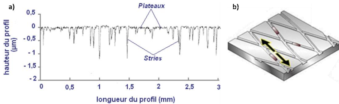
Figure 1-35 : Rodage plateau d'un matériau en fonte à graphite lamellaire : a) exemple de profil de rugosité [Sabri, 2010], et b) représentation schématique de sa topographie et lubrification [Özdeniz, 2016]
