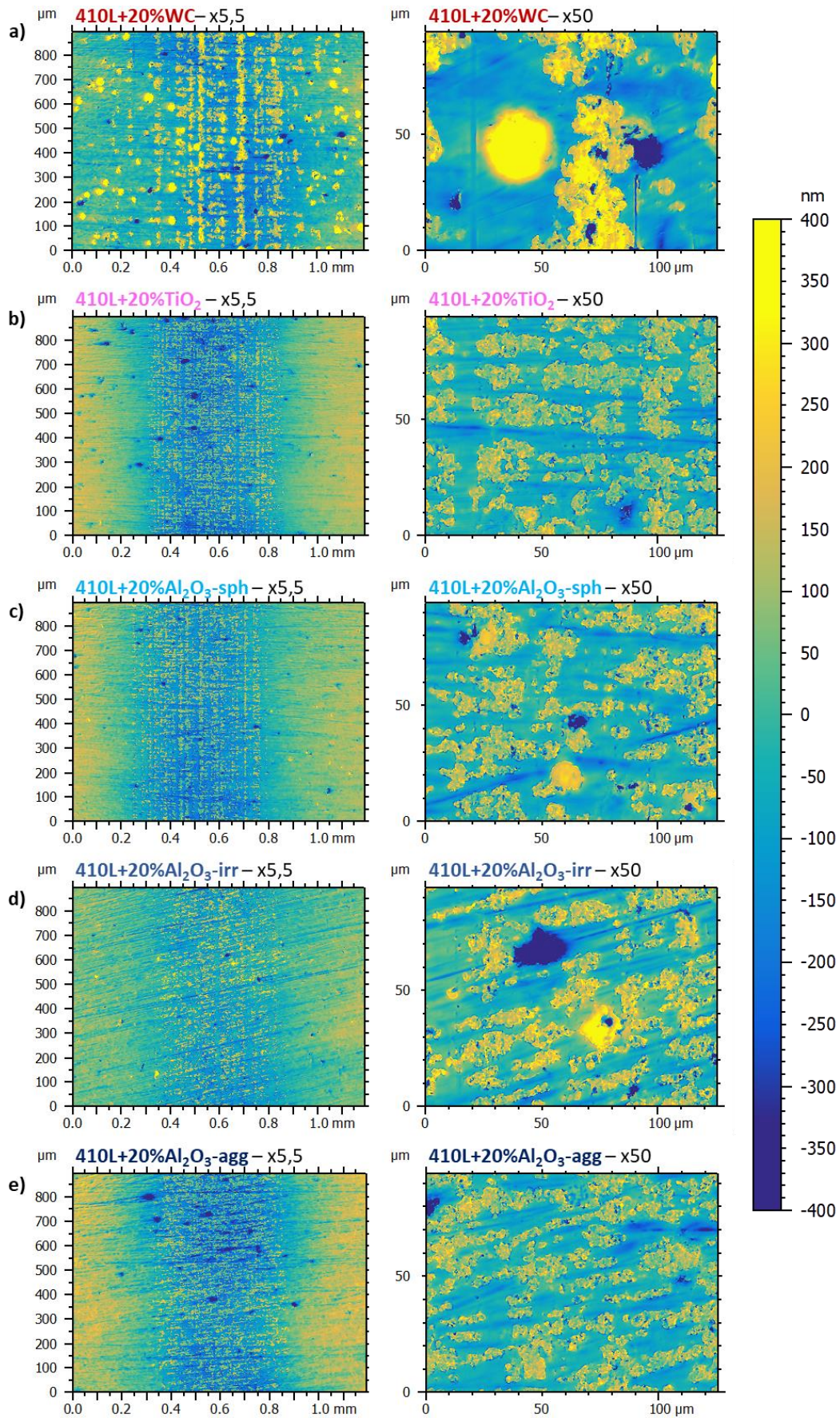
Figure 7-15 : Analyse topographique par WLI au centre de la trace d'usure, aux grossissements \times 5,5 et \times 50 , des revêtements avec renforts céramiques, après l'essai à 100 °C : a) 410L+20%WC, b) 410L+20%TiO 2 , c) 410L+20%Al 2 O 3 -sph, d) 410L+20%Al 2 O 3 -irr, et e) 410L+20%Al 2 O 3 -agg.
