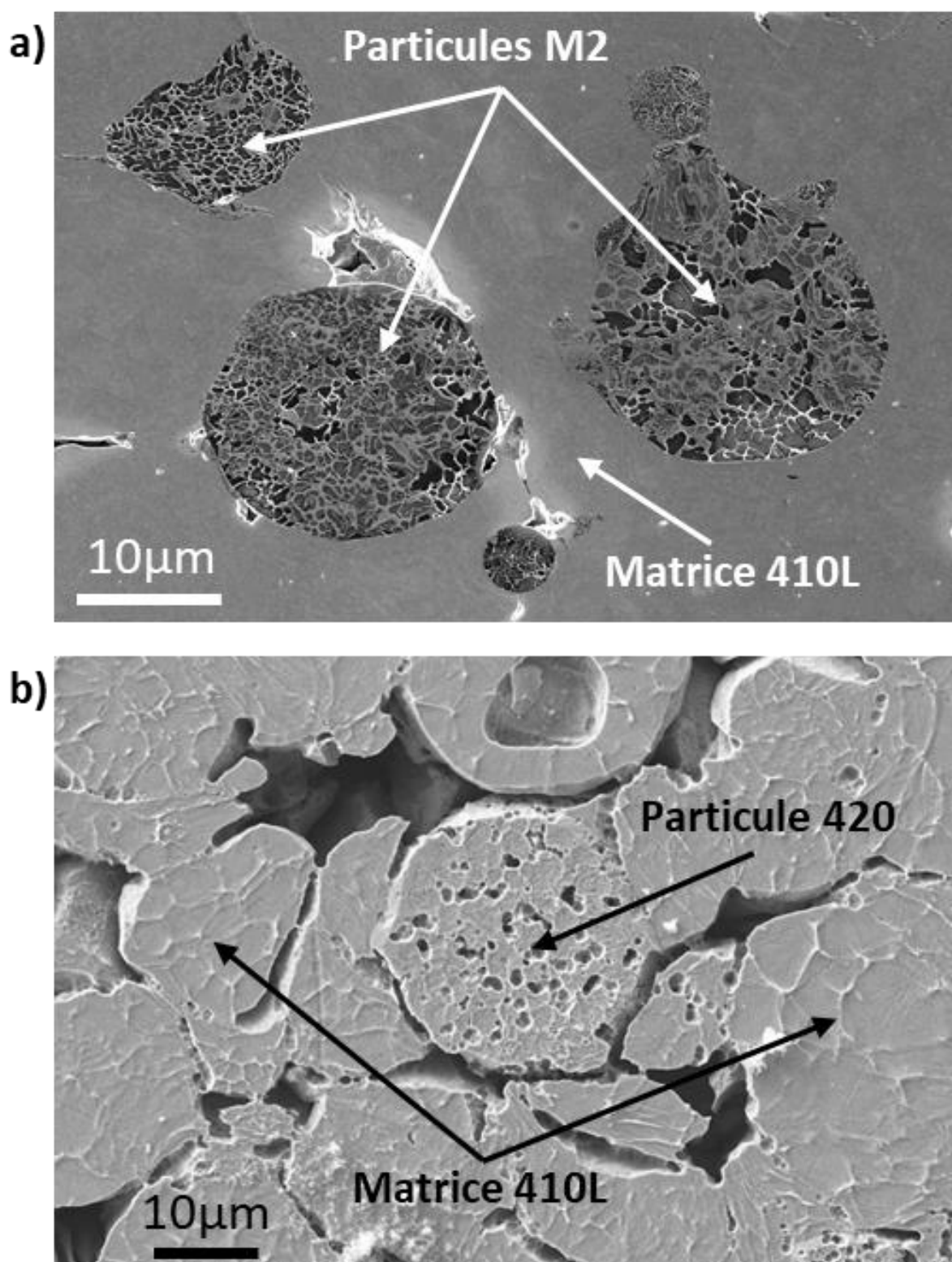
Figure 3-21 : Observations MEB en électrons secondaires de revêtements composites, permettant l'étude de la microstructure des renforts : a) Particules d'acier M2 de granulométrie 10-32 \mu\text{m} dans une matrice 410L dont la structure est révélée par une attaque OPS. b) Particules d'acier 420 de granulométrie 10-32 \mu\text{m} dans une matrice 410L dont les structures sont révélées par une attaque à l'acide oxalique.
