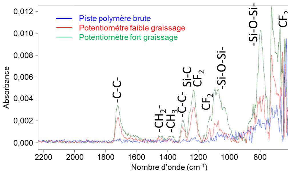
Fig. 4.21 : Spectres d'absorption IR de pistes polymères ; brute en bleu, recouverte de tribofilm peu homogène en rouge (cas du faible graissage) et recouverte de tribofilm relativement homogène en vert (cas du fort graissage). De par la correction de la ligne de base, ces analyses sont utilisées de manière qualitative et non quantitative.
