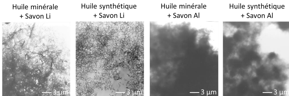
Fig. 1.46 : Microstructures des graisses étudiées par Couronné [139].
