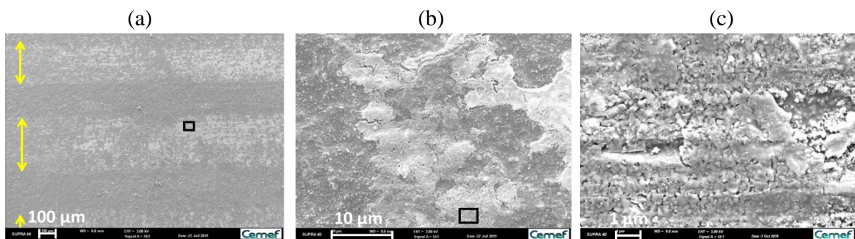
Fig. 4.32 : Image MEB-SE de la surface de la piste polymère graissée avec la graisse C-3 (faible graissage) après lavage avec le solvant Novec 71DA. Il est possible d'observer la formation d'un tribofilm. La largeur des contacts est indiquée par des flèches jaunes ; Zooms de (a) à (c) correspondants aux encadrés noirs.
