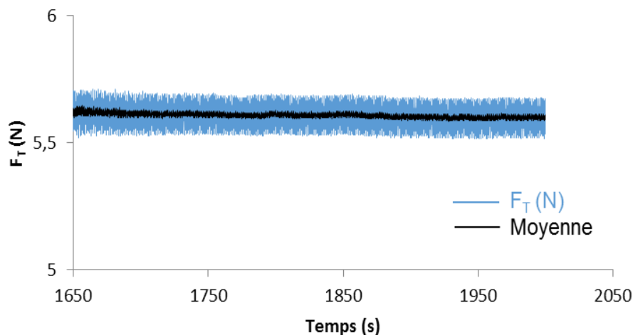
Fig. 2.20 : Évolution de F_T en fonction du temps, obtenue après des tests sur tribomètre pion-disque avec v = 21 mm/s et F_N = 4,3 N.
