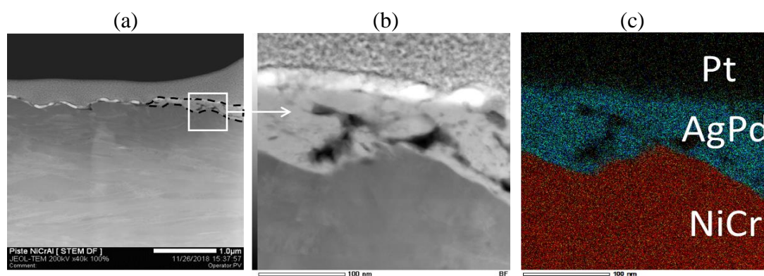
Fig. 3.44 : Analyses en contraste chimique de la piste NiCr dans la zone de contact, issue d'un capteur avec traitement de tribofinition et ayant montré une faible dérive de R_T ; (a) Image MET-DF montrant un dépôt d'une épaisseur pouvant aller jusqu'à 100 nm (entourée en noir) ; (b) Images MET-BF d'une zone zoomée de (a) ; (c) Image en contraste chimique de la même zone ; noir = Pt, bleu = AgPd, rouge = NiCr.
