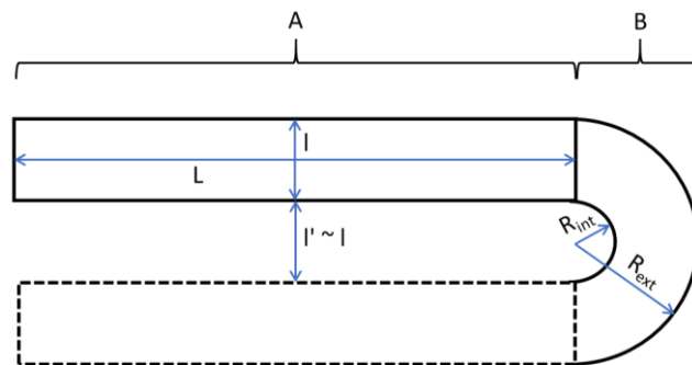
Fig. II.1 : Schéma d'une unité répétitive du serpentins de la piste NiCr dans les rhéostats ; avec L la longueur, l la largeur, l' la largeur entre deux serpentins, R_{int} le rayon interne de la courbure et R_{ext} le rayon externe de la courbure. A est la partie sans courbure, et B est la partie courbée.
