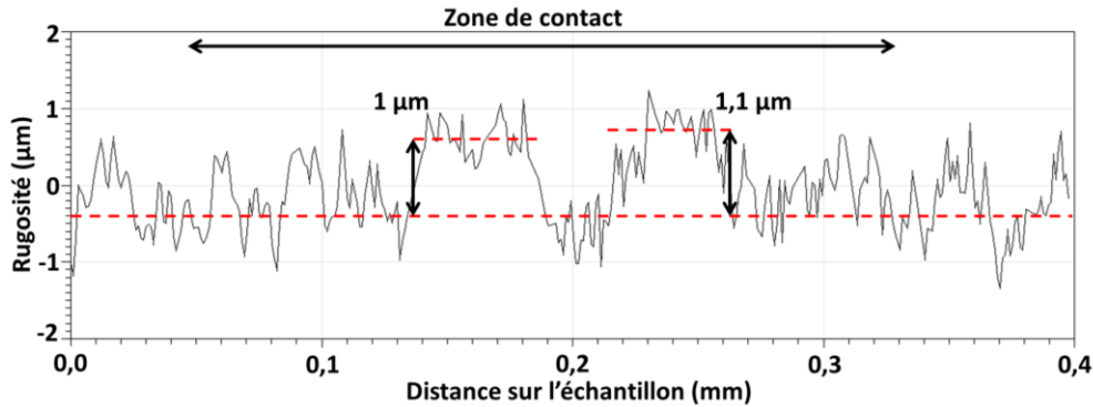
Fig. 4.33 : Mesure en rugosimétrie du tribofilm formé avec la graisse C-2 (faible graissage). Celui-ci est hétérogène et laisse paraître deux amas d'épaisseurs importantes ( 1\ \mu\text{m} et 1,1\ \mu\text{m} ).
