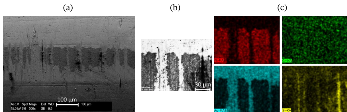
Fig. 3.31 : Analyse du curseur AuCu pour un capteur testé dans les conditions FF (faible pression, faible graissage, en bas à gauche sur la figure Fig. 3.30), dont la piste a été fortement utilisée ; (a) Image MEB-SE du curseur avec un dépôt au niveau de la zone du contact ; (b) Image MEB-BSE d'une zone du contact ; (c) Analyse EDX de la zone (b) avec rouge = Ni, vert = Cr, cyan = Au et jaune = Si.
