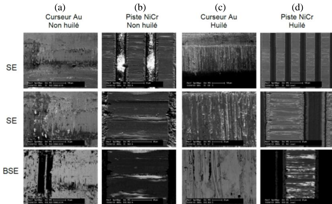
Fig. I.4 : Images MEB du système NiCr – AuCuPt ; (a) & (b) Dans le cas sec ; (c) & (d) Dans le cas lubrifié à l'huile A-1.
