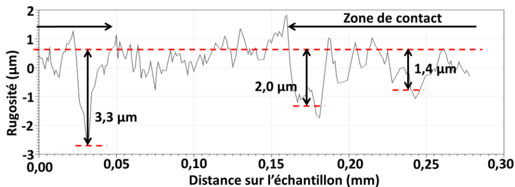
Fig. 4.28 : Mesure en rugosimétrie de deux zones de contact (notées avec des flèches) sur la piste graissée avec la graisse B (fort graissage). De fortes usures apparaissent ( 1,4 \mu\text{m} à 3,3 \mu\text{m} de profondeur), mais sous forme de stries, localisées à quelques endroits de la zone de contact.
