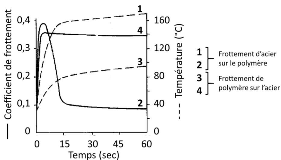
Fig. 1.21 : Évolution des coefficients de frottement en fonction de la température de contact (contact rotatif sous une charge de 30 kg et une vitesse de 0,45 m/s), d'après les travaux de Vinogradov [79] ; dans le cas de l'acier frottant sur le polymère (1&2) ; dans le cas du polymère frottant sur l'acier (3&4).
