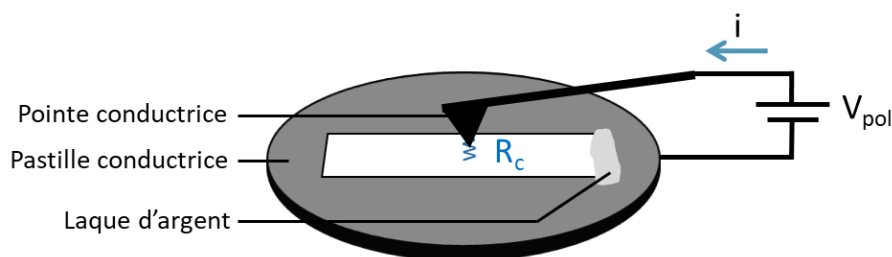
Fig. 2.24 : Schéma du contact dans la mesure au Résiscope ® , avec la pointe conductrice de l'AFM et le schéma électrique permis par le contact électrique entre l'échantillon et la pastille conductrice.
