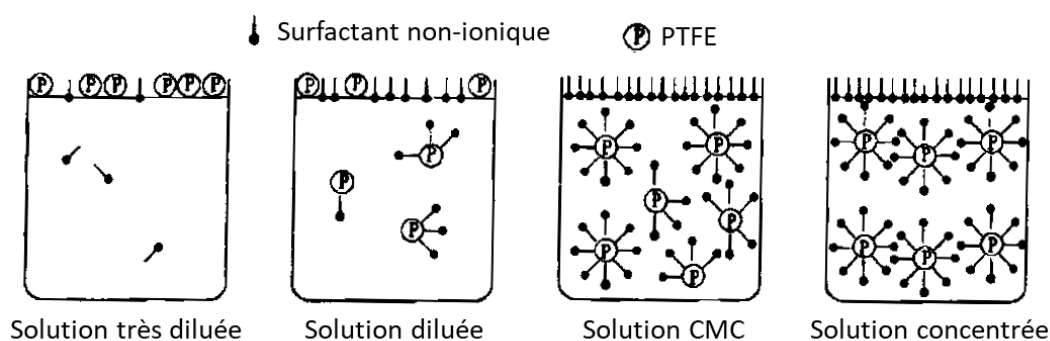
Fig. 1.43 : Mécanisme de miscibilité du PTFE dans l'huile en présence d'une concentration variable en dispersant non ionique, proposé par Matsuda et al. [155].
