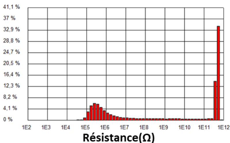
Fig. 2.14 : Histogramme des résistances mesurées sur la zone 5 μm × 5 μm associée à la figure Fig. 2.13(b). Les valeurs sont présentées en % de résistances comprises entre 10 2 et 10 12 Ω.
