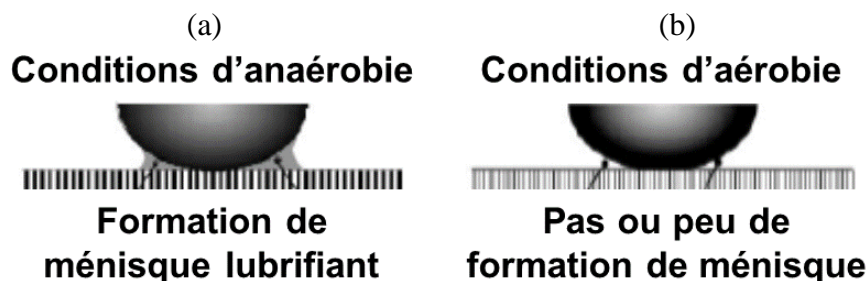
Fig. I.1 : Schémas des contacts dans le cas d'un lubrifiant de type huile ; (a) Dans les conditions d'anaérobie ; (b) Dans les conditions d'aérobie, selon Glossbrenner [233].
