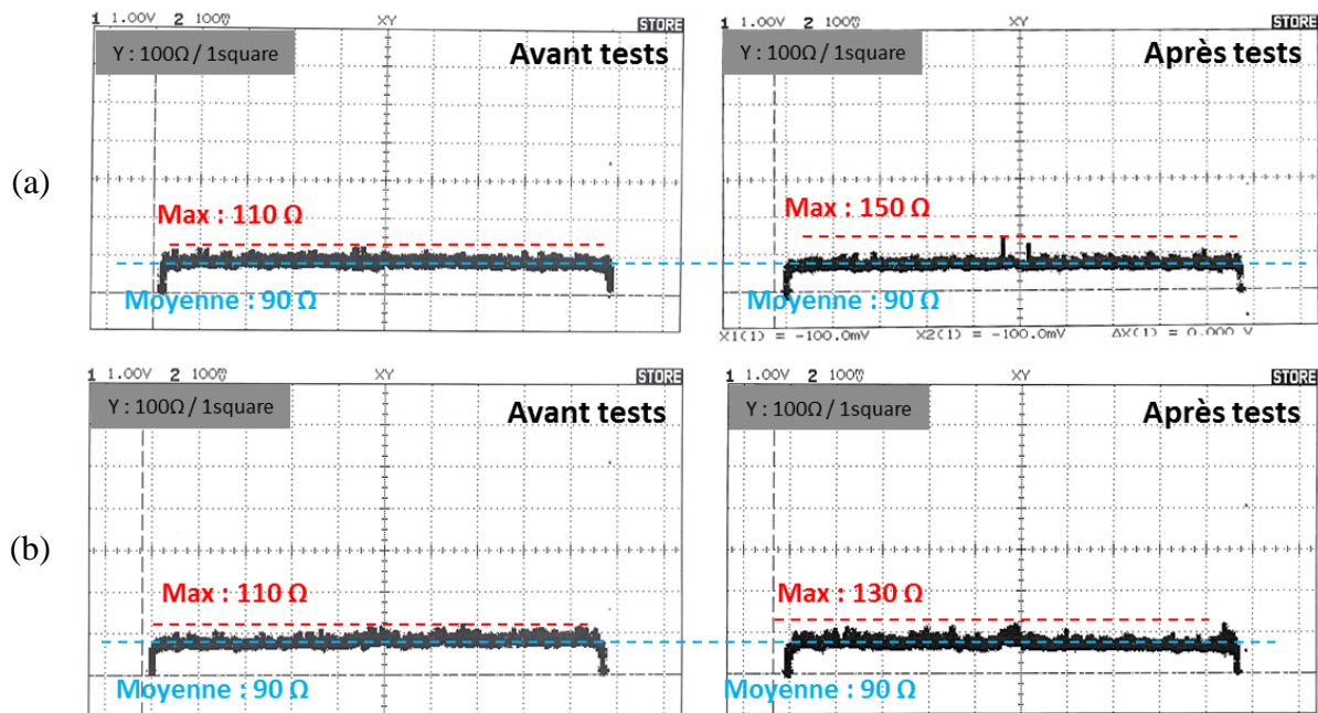
Fig. 4.19 : Mesure de R_c , dans le cas d'un contact lubrifié à la graisse A-2 ; (a) Avant et après essai d'endurance pour un graissage normal (environ 0,5 \text{ g/m}^2 ) ; (b) Avant et après essai d'endurance pour un graissage fort (environ 9 \text{ g/m}^2 ).
