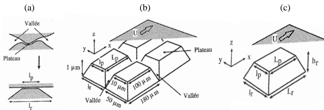
Fig. 1.30 : Surfaces dans l'étude de Letalleur [126] ; (a) Schéma de simplification d'une surface réelle en surface vallées-plateaux ; (b) Surface étudiée par Letalleur ; (c) Définitions des longueurs L_p , L_r , l_p et l_r .
