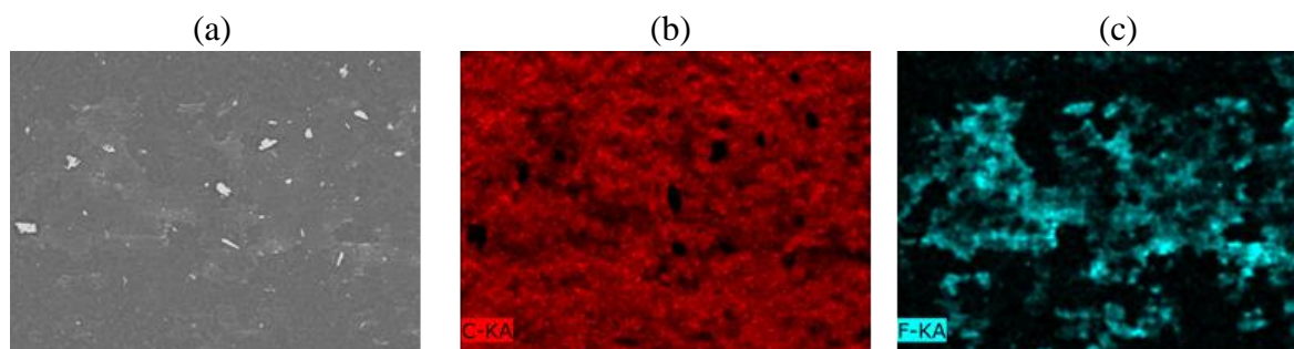
Fig. 4.35 : Image MEB-BSE et analyse EDX correspondante du tribofilm de la piste polymère, après essai d'endurance, avec rouge = C et cyan = F ; pour un graissage C-3. Les particules en gris très clair sur l'image (a) sont riches en éléments métalliques.
