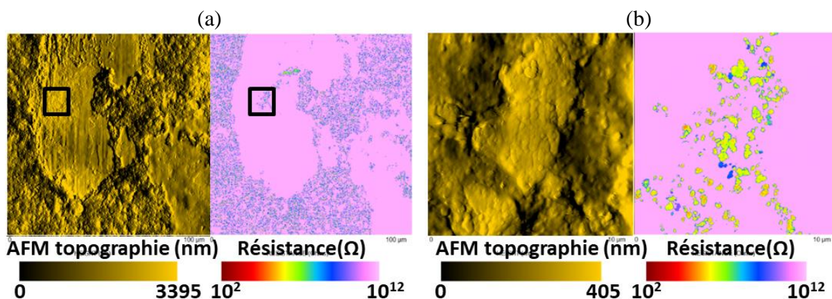
Fig. 4.12 : Images AFM-Résiscope ® (topographie-valeurs de résistances) de pistes polymères chargées carbone dans des zones recouvertes de troisième corps ; (a) Couple d'images d'une zone de 100\ \mu\text{m} \times 100\ \mu\text{m} ; (b) Couple d'images d'une zone de 10\ \mu\text{m} \times 10\ \mu\text{m} (grossissement de (a) dans un amas du troisième corps, correspondant à l'encadré noir).
