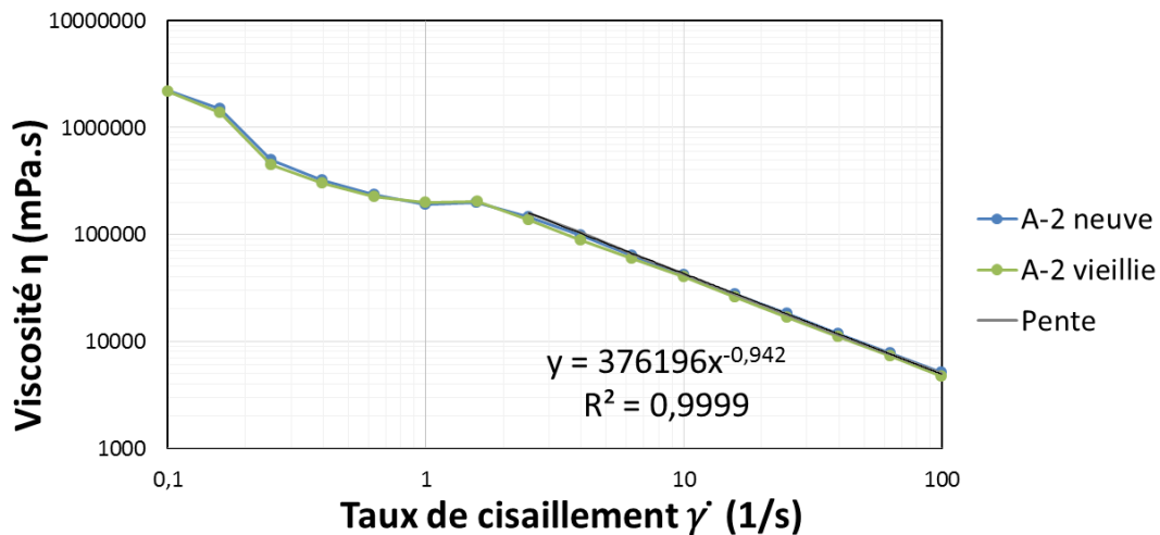
Fig. 2.16 : Exemple de courbe de viscosité en fonction du cisaillement appliqué \dot{\gamma} , pour la graisse silicone chlorée + PTFE (A-2), la pente étant ici égale à -0,942.
