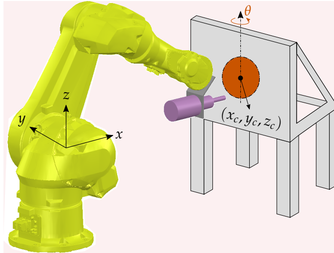
FIGURE A.22: Schéma de la cellule de travail pour le processus d'ébavurage
