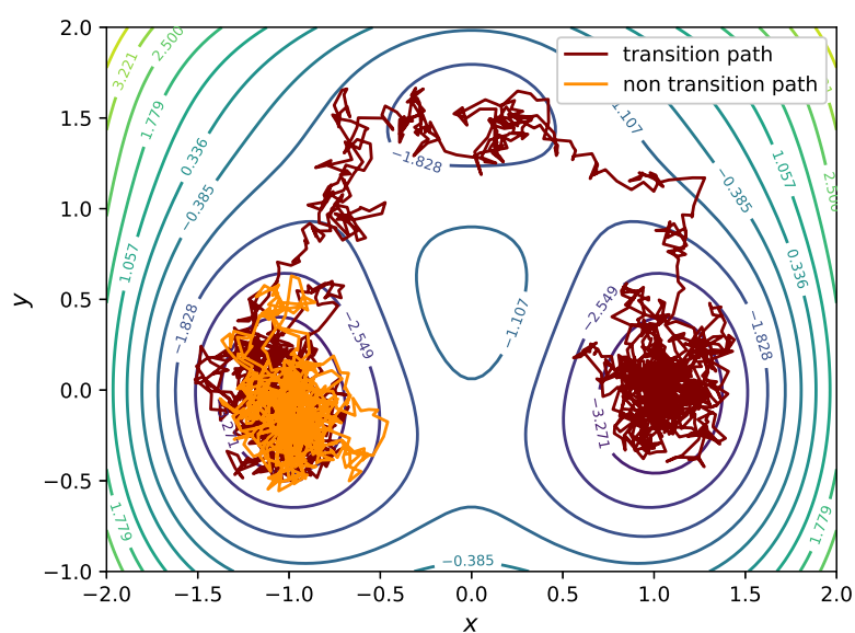
Figure 5.1 – Trajectoire de transition et trajectoire de non-transition dans le potentiel bidimensionnel donné par (4.3).
