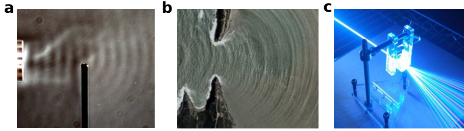
FIG. 1.1: Exemple de diffraction d'ondes. (a) Ondes sonores diffractées par un obstacle et visualisées par stroboscopie [11]. (b) Vagues diffractées à l'entrée d'un port par une digue jouant le rôle de fente. Source : GoogleEarth (c) Diffraction de la lumière par un réseau périodique. Source : Physics Open-Lab.org .
