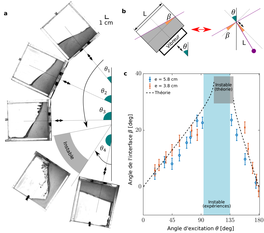
FIG. 6.1: Angle d'équilibre pour un bac de longueur L = 9 cm (a) Photographies d'une interface vibrée dans différentes directions (b) Notations et schéma d'une interface liquide et du pendule équivalent associé (c) Mesure de l'angle \beta entre la normale à l'excitation et l'interface pour différents angles d'excitation \theta . Le pendule associé a pour pulsation \omega_0^2 = \alpha_0 g |\cos \beta| / L avec \alpha_0 = 2.3 .
