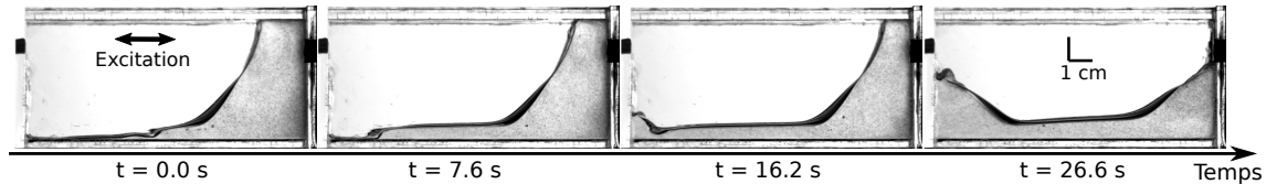
FIG. 6.8: Lorsque le forçage V_{exc} est maintenu constant juste en dessous de la vitesse limite V_{lim} , on observe la fuite de liquide par une langue de quelques millimètres dont la progression est lente. Lorsque le liquide atteint l'autre extrémité du bac, une seconde accumulation de liquide se forme jusqu'à ce que le liquide soit dans un nouvel état symétrique stable ( t = 26.6 s).
