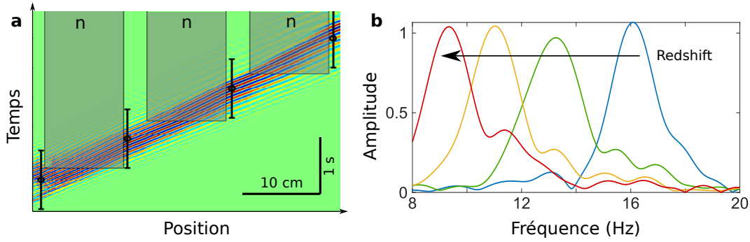
FIG. 3.8: (a) Diagramme spatio-temporel d'une cascade descendante en fréquence. La tension de chaque électrode passe de 0 à V_0 lors du passage du paquet d'onde et sort ensuite de sous l'électrode par une interface spatiale. (b) Spectre fréquentiel du paquet d'onde après chaque transformation élémentaire
