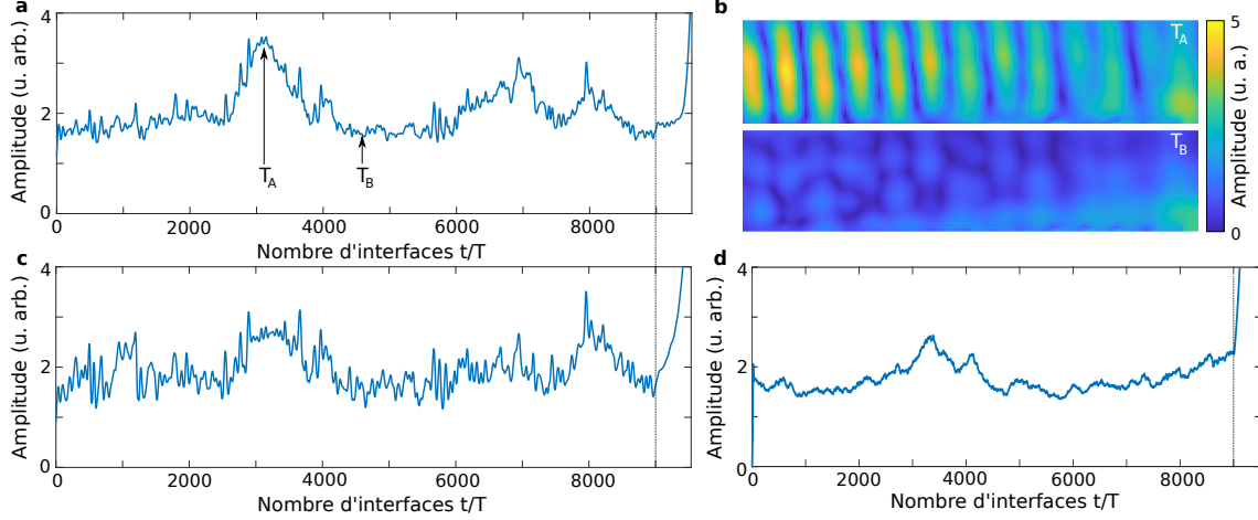
FIG. 4.4: (a) Amplitude des ondes en fonction du temps pour un taux de croissance nul et un désordre \sigma \approx 0.09 . L'amplitude est approximativement constante mais présente des phénomènes d'intermittence. (b) Lorsque la même séquence de pics est envoyée, les mêmes phénomènes d'intermittence sont observés. (c) Simulation de l'amplitude des ondes pour la même séquence de pics. Les événements de localisation similaire sont visible. (d) Valeur absolue de l'amplitude du champ d'onde mesuré durant un pic d'intermittence (en haut) et hors d'un pic (en bas).
