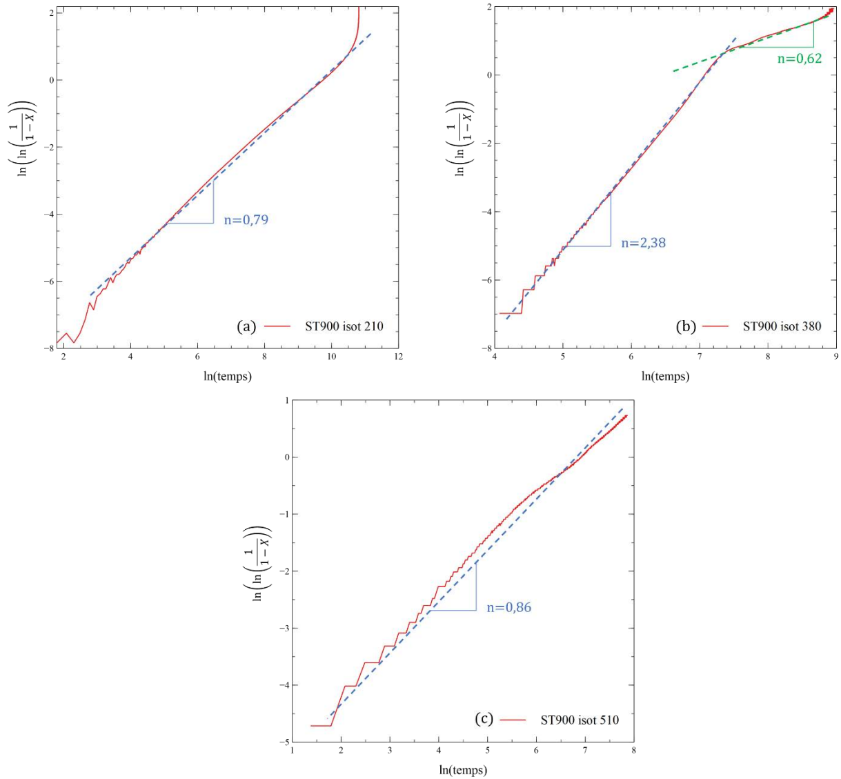
figure 5-16 : diagrammes de JMAK pour des isothermes à (a) 210°C, (b) 380°C, (c) 450°C et (d) 510°C, après mise en solution à 900°C
