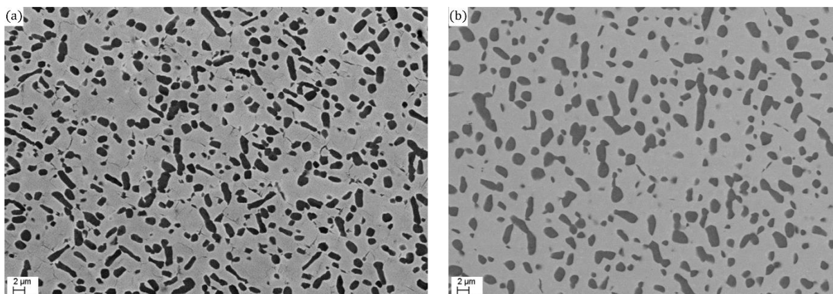
figure 3-24 : Micrographies MEB (a) d'un état brut de forge K=3,8 et (b) d'un état K=3,8 ayant subi un traitement de mise en solution à 800°C pendant 2h
