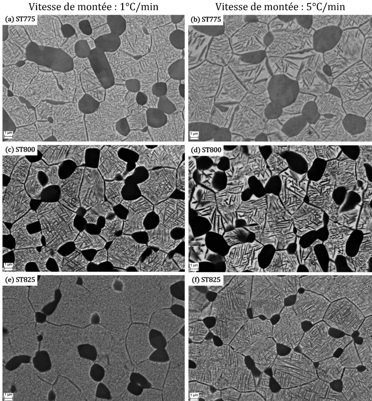
figure 4-18 : Microstructures d'échantillons issus de la barre forgée K=2,7 ayant subi un traitement de mise en solution à (a, b) 775°C, (c et d) 800°C et (e et f) 825°C puis un traitement de revenu à 600°C pendant 8h avec une vitesse de montée de (a, c et e) 1°C/min, (b, d et f) 5°C/min
