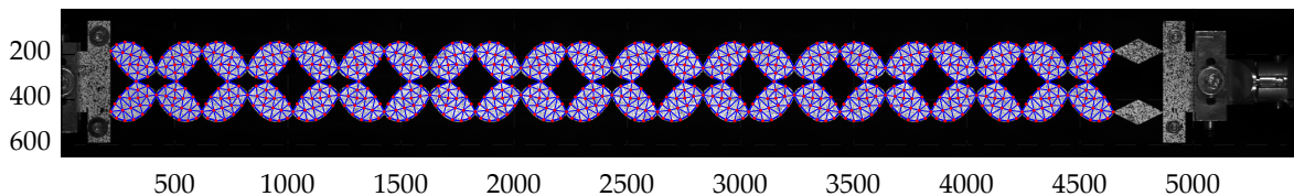
FIGURE IV.34 – ROI \Omega (blanc transparent) et maillage utilisés pour la mesure du déplacement par CIN globale. Représentation sur la configuration initiale, au début de l'essai S-C.
