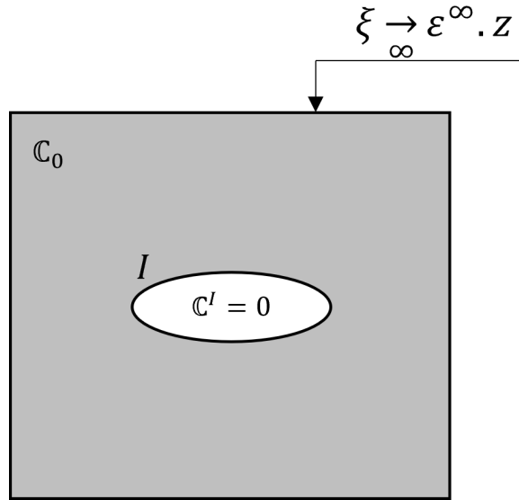
FIGURE A-4 – Problème inclusionnaire d'Eshelby
