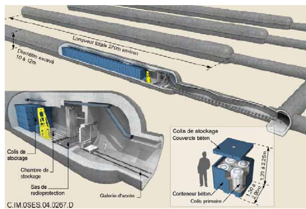
FIGURE 1-3 – Illustration d’une Alvéole de stockage
