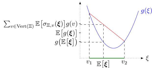
Figure 1.2: Une illustration des inégalités de Jensen et d'Edmundson-Madansky, voir aussi la proposition 6.7
