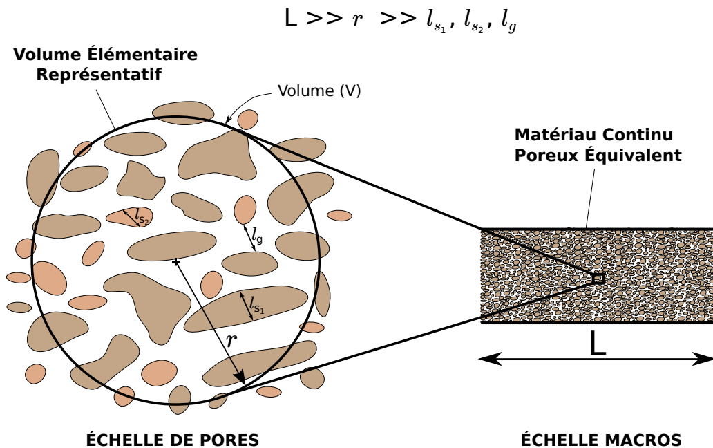
FIGURE 1.2 – Concept générique du processus de mise à l'échelle. Le processus repose sur les hypothèses de séparation d'échelle ( L \gg r \gg l_{s_1}, l_{s_2}, l_g ) et sur l'existence d'un REV où les variations à petite échelle sont atténuées.
