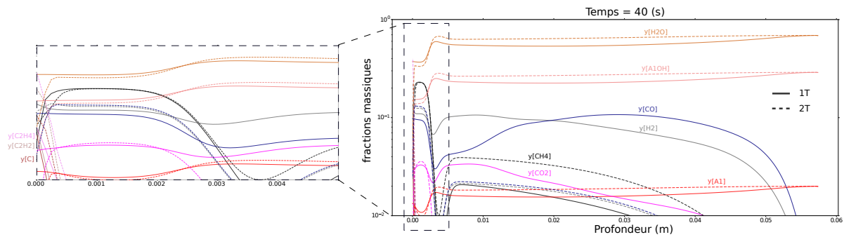
FIGURE 1.8 – Cas Stardust. Distribution des espèces dans le matériau au temps t = 40 s. A gauche: un zoom sur les fractions massiques près de la surface avec l'environnement externe.
