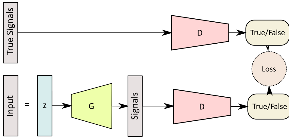
FIGURE 3.3 – Schéma du GAN classique
