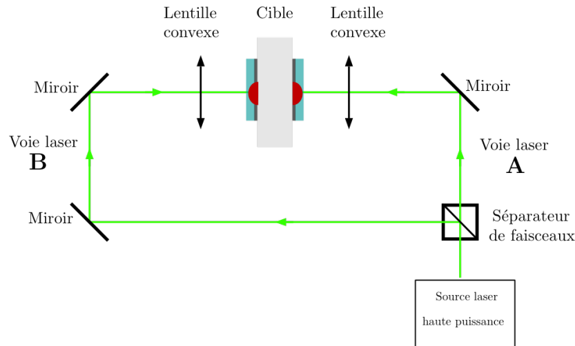
FIGURE 1.15 – Schéma de principe du choc laser symétrique
