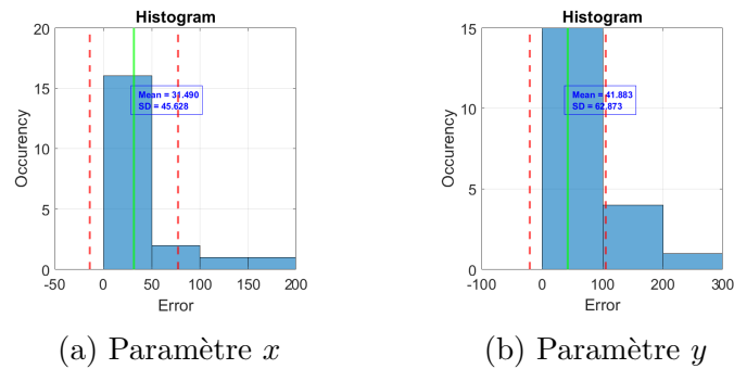
FIGURE C.2 – Histogrammes des erreurs de la résolution inverse sur S2 avec RBF et SVD
