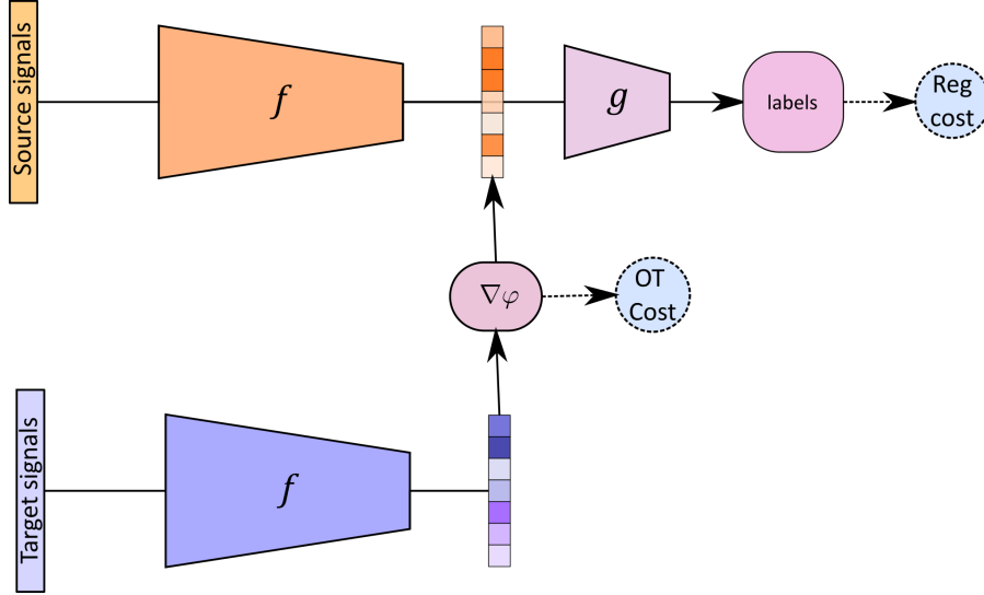
FIGURE 5.5 – Apprentissage de transfert profond basé sur le transport de caractéristiques avec la dualité de Monge-Kantorovich
