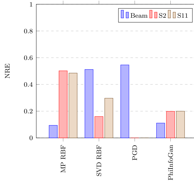
FIGURE 3.18 – Erreur moyenne (NRE) de prédictions des métamodèles sur les trois cas d'étude (Poutre, S2 et S11)
