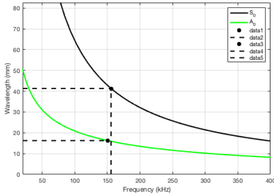
(a) Longueur d'onde en fonction de la fréquence
