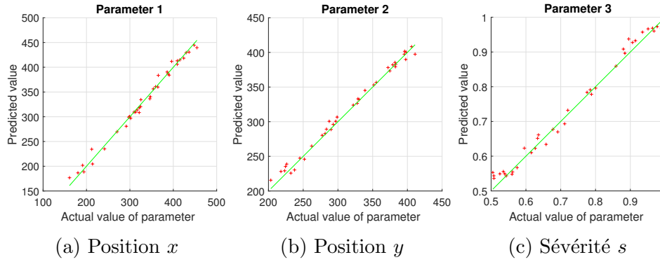
FIGURE 4.15 – Évaluation du CNN temporel sur le cas 1
