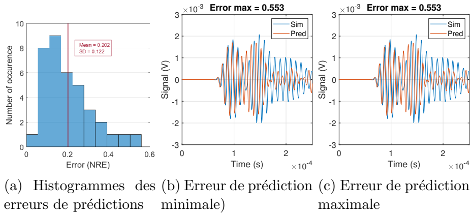
FIGURE B.6 – Évaluation du RBF avec SVD sur la structure S11
