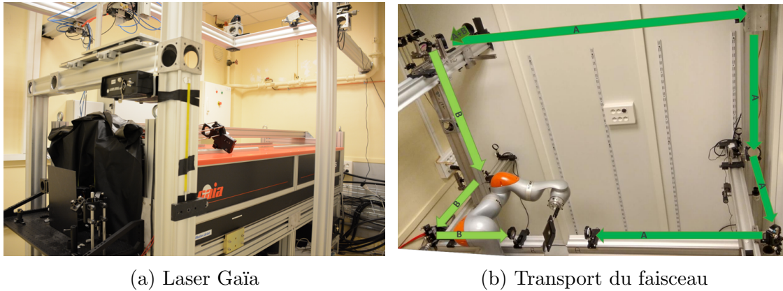
FIGURE 1.14 – La plateforme Héphaïstos du PIMM
