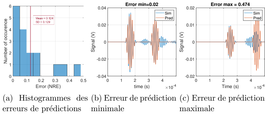
FIGURE B.1 – Évaluation du RBF avec MP sur la structure poutre
