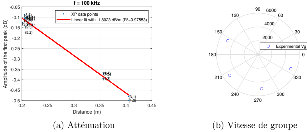
FIGURE 2.3 – Caractérisation expérimentale du premier paquet d'ondes dans la structure X11 à 100kHz
