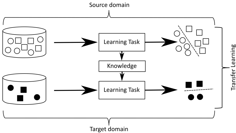
FIGURE 5.1 – Exemple simple d’apprentissage par transfert : ici la tâche source consiste à distinguer des carrés creux des cercles creux. L’apprentissage peut être transféré pour distinguer les cercles pleins des carrées pleins.
