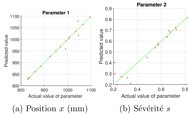
FIGURE 4.3 – Évaluation de la résolution inverse sur la Poutre avec RBF + MP
