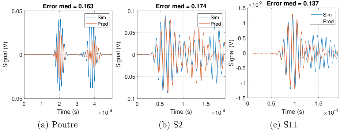
FIGURE 3.17 – Erreur médiane de l'évaluation de l'InfoGAN
