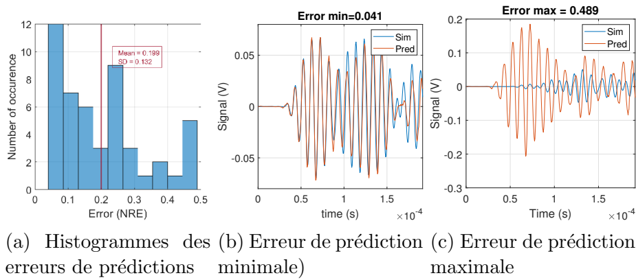
FIGURE B.7 – Évaluation du S-InfoGAN sur la structure S2
