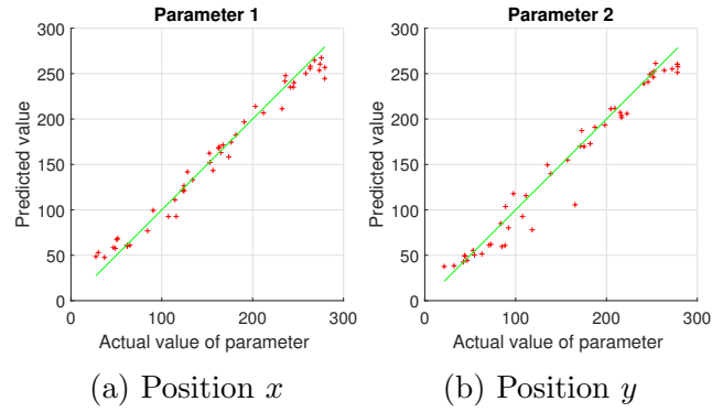
FIGURE 4.14 – Évaluation de la résolution inverse sur S2 avec CNN temporel. Des figures équivalentes sont obtenues avec le CNN avec TVDI.
