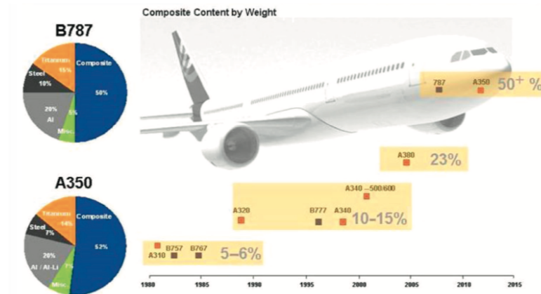
FIGURE 1.1 – Évolution du pourcentage en masse des matériaux composites dans les avions [1]
