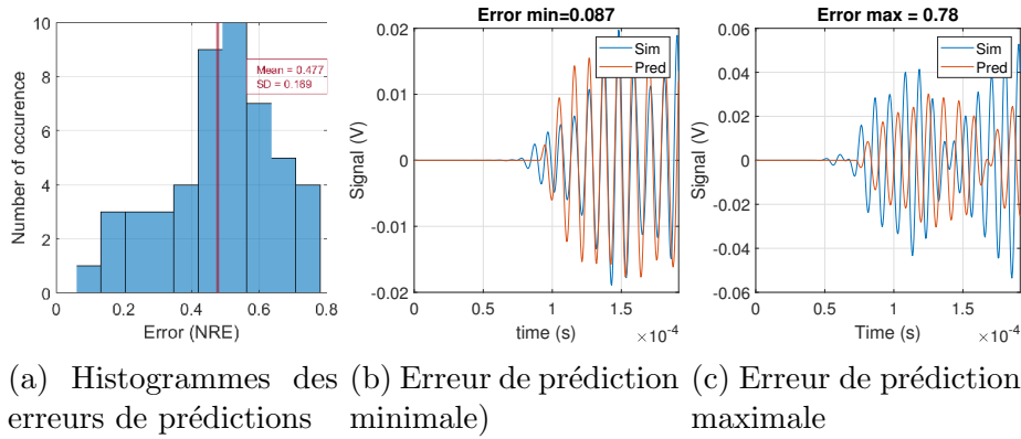
FIGURE B.3 – Évaluation du RBF avec MP sur la structure S2
