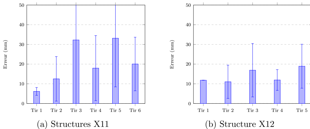
FIGURE 4.22 – Erreur de localisation sur les structures expérimentales du CNN temporel
