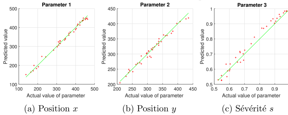
FIGURE 4.16 – Évaluation du CNN TVDI sur le cas 1
