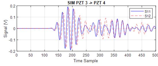
FIGURE 4.7 – Comparaison des signaux à l'état sain de la structure S11 et S12
