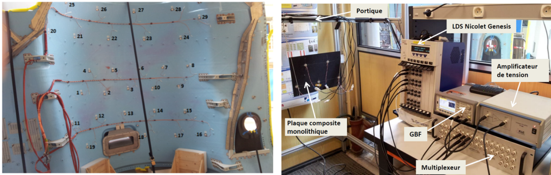
(a) La nacelle équipée d'un réseau de PZT (b) Plaque en cours d'inspection au laboratoire Procédé et Ingénierie en Mécanique et Matériaux (PIMM) [45]
