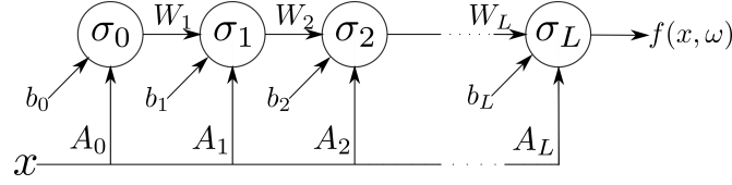
FIGURE 5.8 – Schéma d'un ICNN
