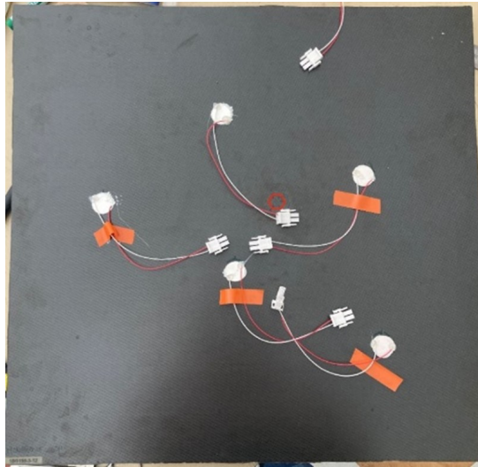
(c) Structure X11 équipée de PZTs
