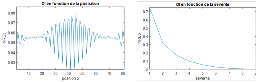
FIGURE 2.12 – Exemple caractéristique d'évolution d'un DI dans la poutre en fonction de la position et de la sévérité
