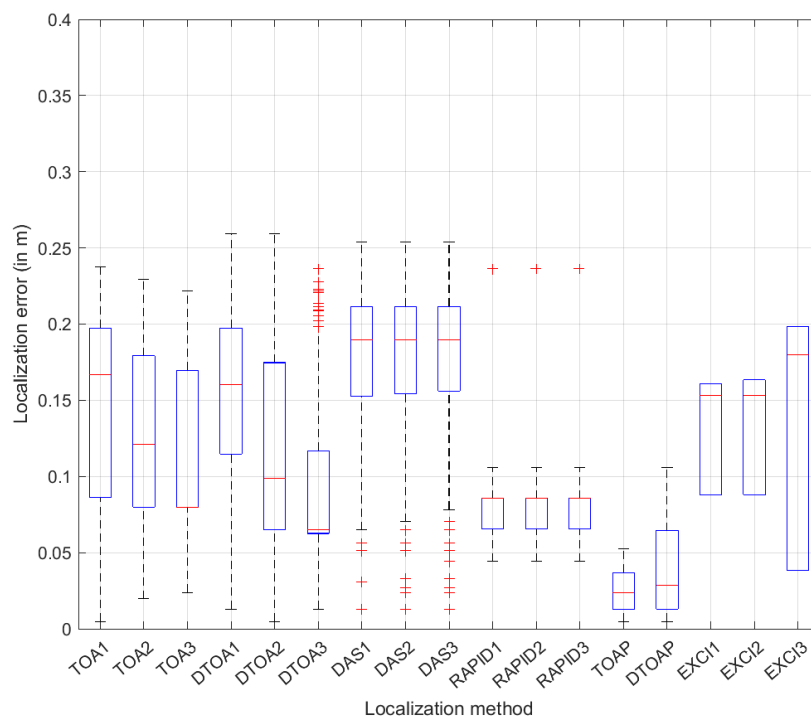
FIGURE 2.8 – Évaluations des méthodes de localisation sur les structures X11 et X12
