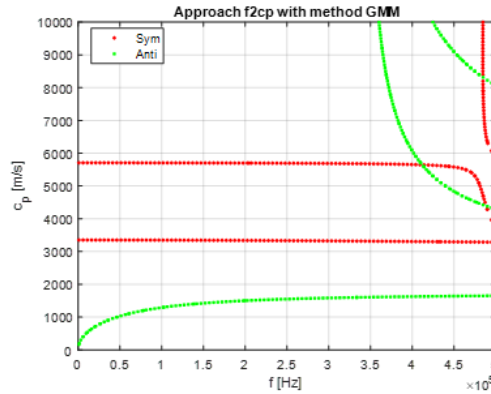
FIGURE 1.9 – Exemple d’une courbe de dispersion des ondes de Lamb dans un matériau composite aéronautique
