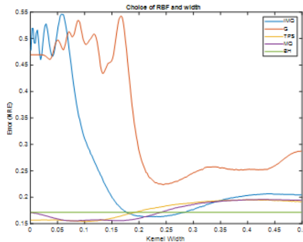
FIGURE 3.13 – Erreur en fonction de la largeur \varepsilon pour différentes fonctions RBF pour la poutre avec MP
