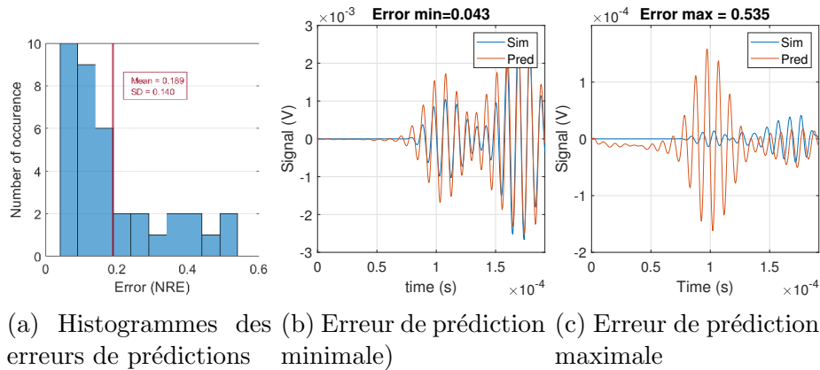
FIGURE B.8 – Évaluation du S-InfoGAN sur la structure S11
