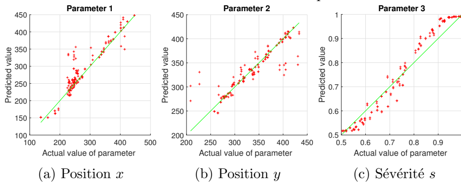
FIGURE 4.20 – Évaluation du CNN TVDI sur le cas 3
