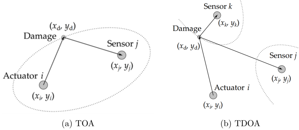
FIGURE 1.13 – Méthodes de localisation par le calcul des temps de vol [59]
