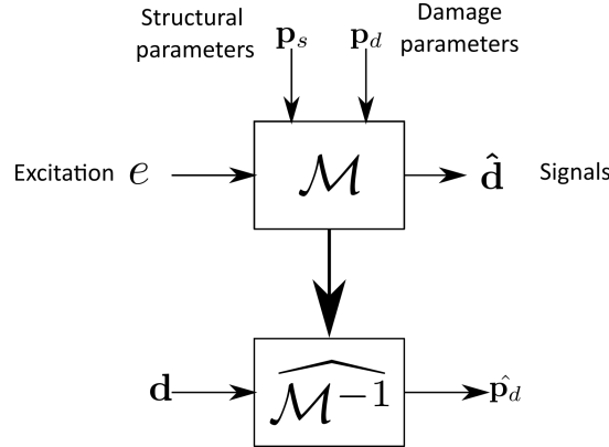
FIGURE 4.6 – Résolution inverse par un métamodèle dédié
