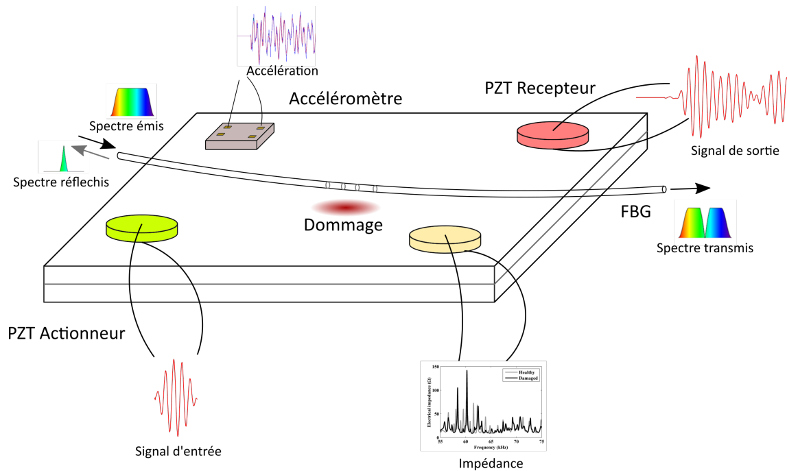
FIGURE 1.7 – Structure intelligente équipée d'un ensemble de transducteurs pour réaliser des mesures
