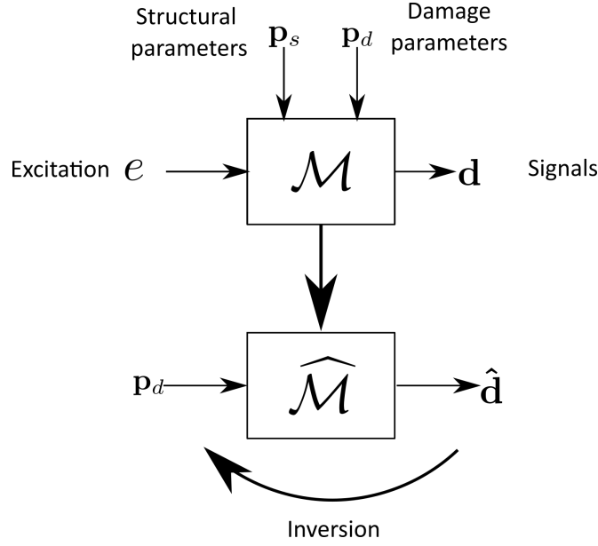
FIGURE 4.1 – La résolution inverse vise à trouver les paramètres du dommages \mathbf{p}_d à l'aide des prédictions rapides \hat{\mathbf{d}} du métamodèle \hat{\mathcal{M}}
