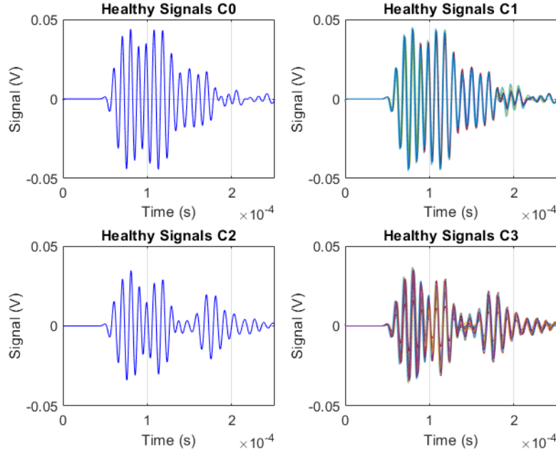
FIGURE 5.3 – Signaux sains utilisés pour le calcul des SIs (uniquement le signal du chemin PZT1 vers PZT3 est affiché). Pour les structures C_1 et C_3 , il y a plusieurs signaux sains, un pour chaque coupon.
