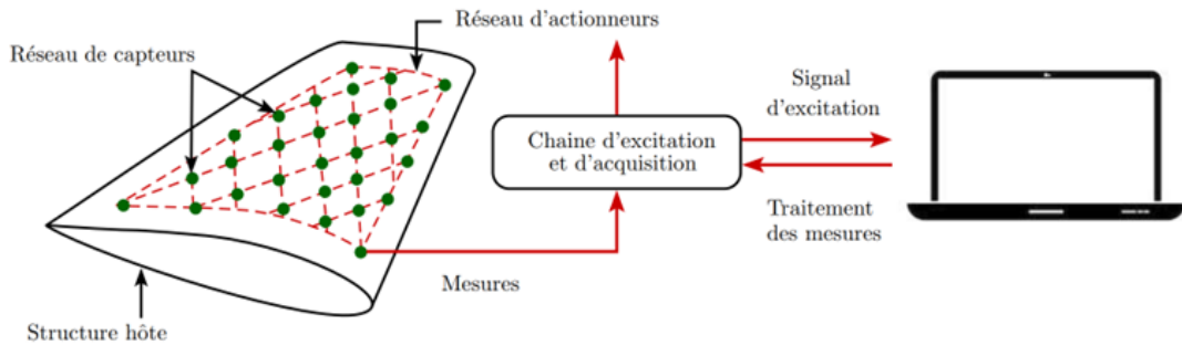
FIGURE 1.10 – Structure intelligente équipée d’un réseau de PZTs [8]
