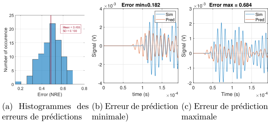
FIGURE B.5 – Évaluation du RBF avec MP sur la structure S11
