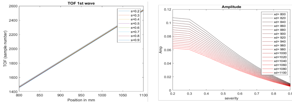
FIGURE 2.11 – Évolution de l'amplitude et du temps de vol du premier paquet dans la poutre
