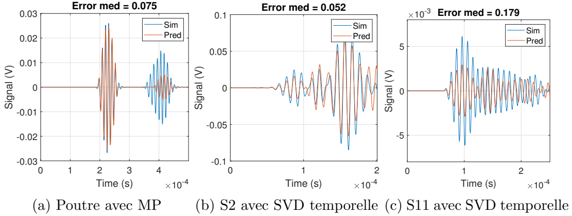
FIGURE 3.14 – Erreur médiane de l'évaluation de la RBF
