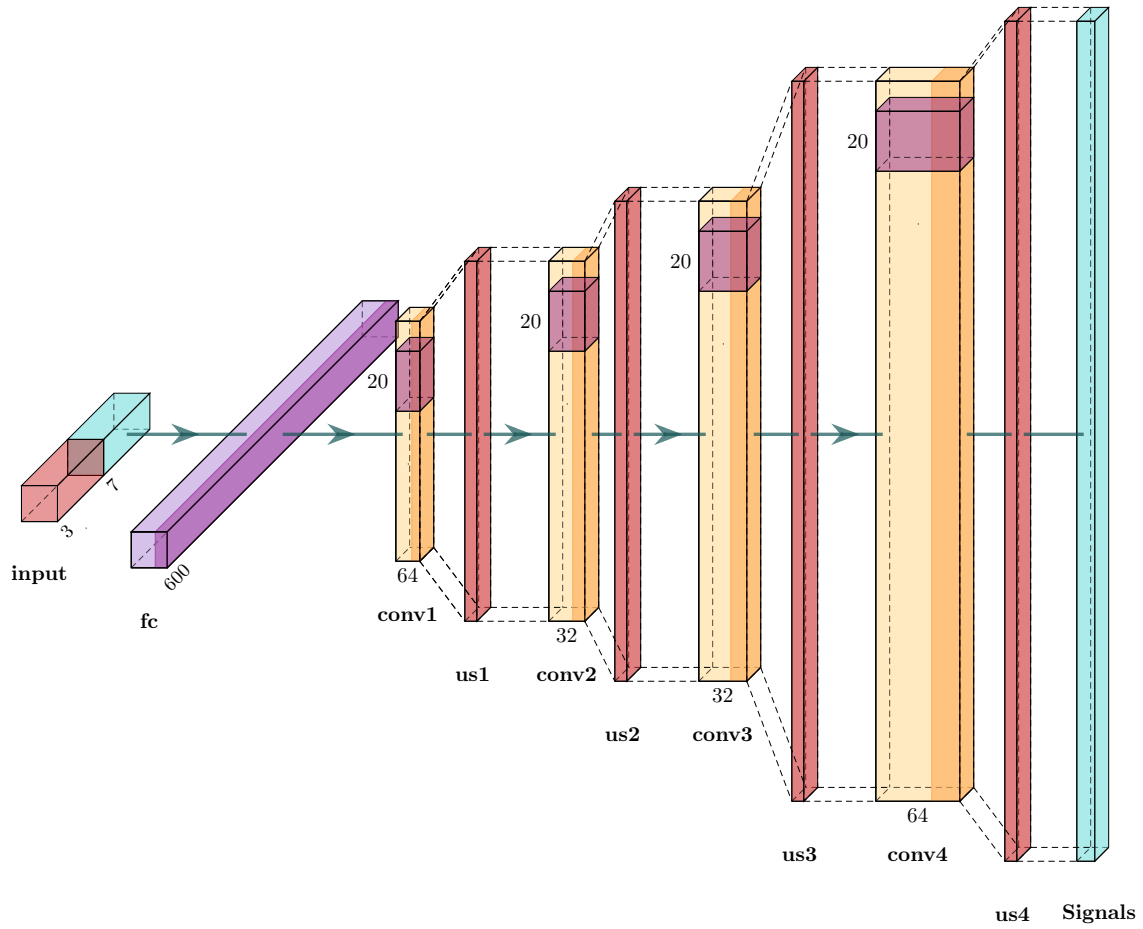
(a) Générateur de signaux
