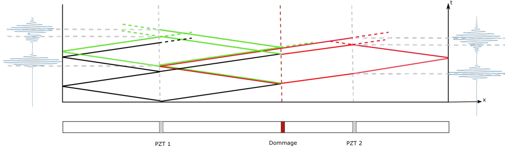
FIGURE 2.10 – Diagramme XT de propagation du premier mode dans la poutre
