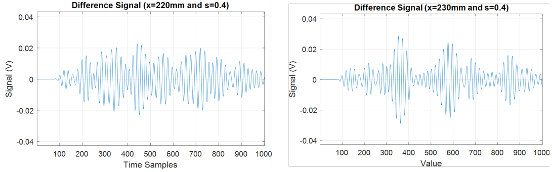
FIGURE 2.14 – Signal de différence de la plaque S2 où le dommage est déplacé de 10mm.
