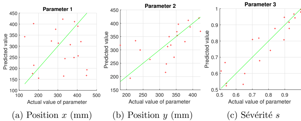
FIGURE 4.5 – Évaluation de la résolution inverse sur S11 avec la RBF et SVD
