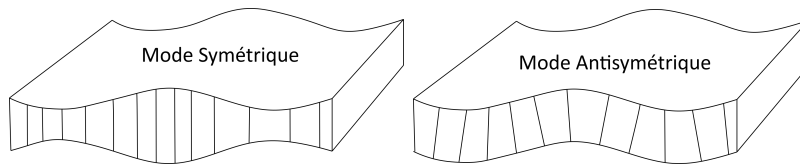
FIGURE 1.8 – Mode symétrique et antisymétrique dans une plaque
