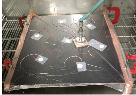
(b) Collage des PZTs sous vide dans une étuve
