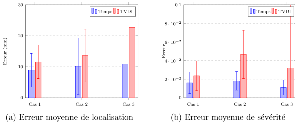
FIGURE 4.21 – Comparaison prédictions du CNN sur les différents cas de S11
