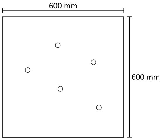
(a) Proposition de placement des PZTs sur la structure X11
