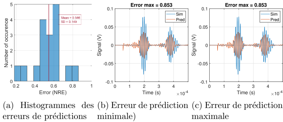
FIGURE B.2 – Évaluation du RBF avec SVD sur la structure poutre
