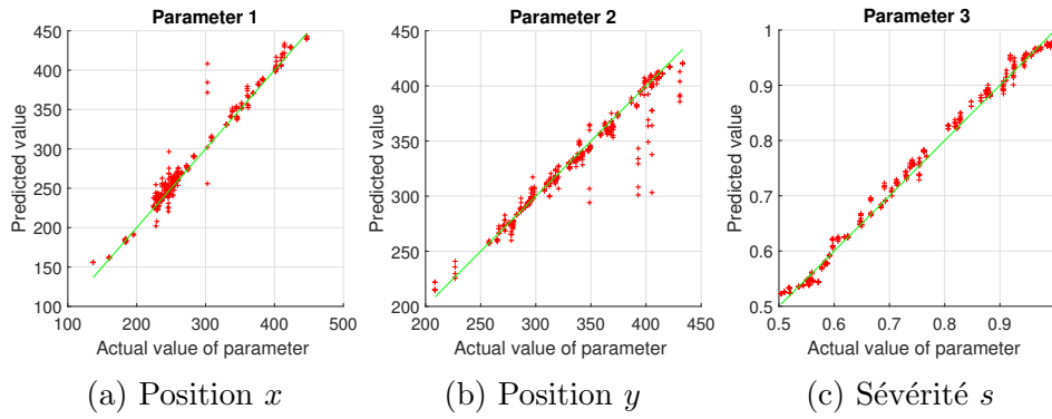
FIGURE 4.19 – Évaluation du CNN temporel sur le cas 3
