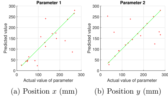
FIGURE 4.4 – Évaluation de la résolution inverse sur S2 avec RBF et SVD
