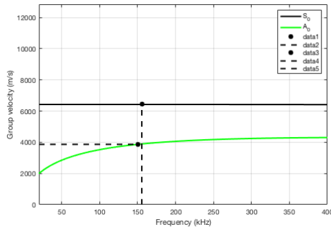
(c) Vitesse de groupe en fonction de la fréquence
