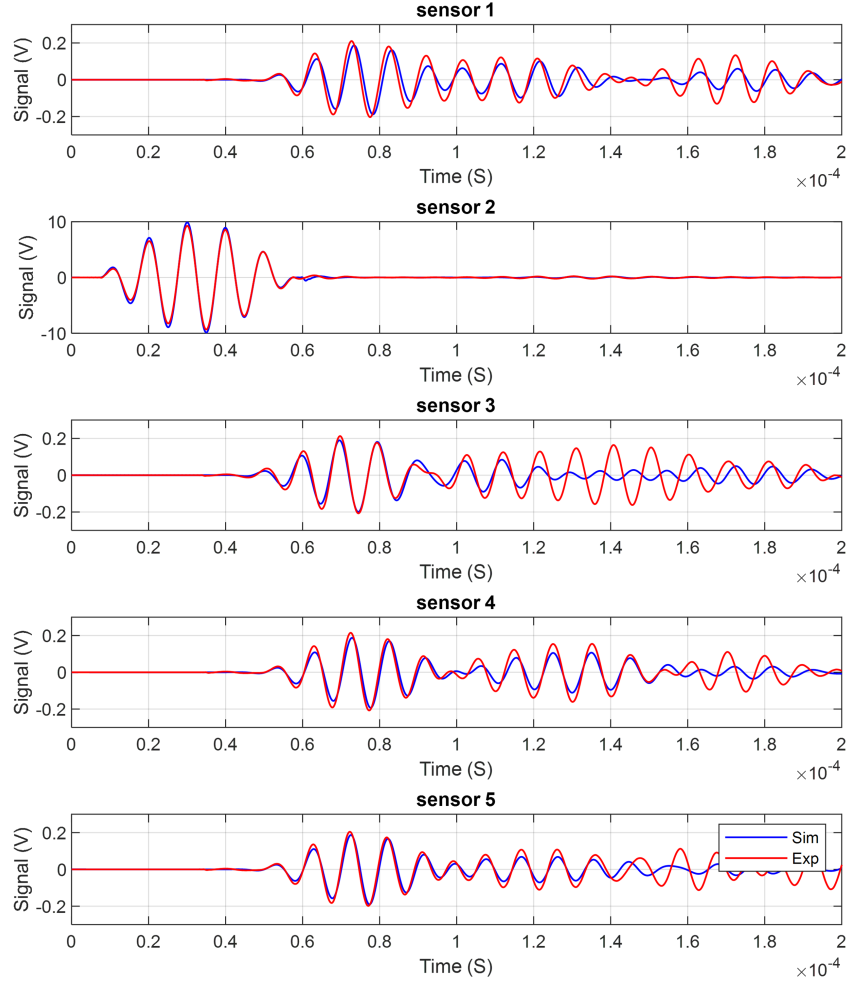
FIGURE 2.9 – Comparaison des signaux numériques et expérimentaux avec le PZT2 en actionneur à 100kHz
