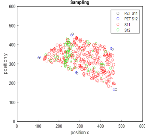
FIGURE 4.8 – Échantillonnage et placement des capteurs pour les structures S11 et S12
