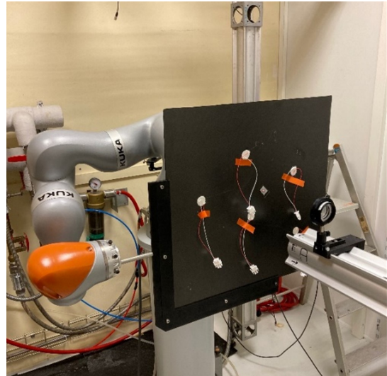
(d) Structure X11 en cours d'endommagement dans la plateforme Héphaïstos
