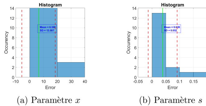
FIGURE C.1 – Histogrammes des erreurs de la résolution inverse sur la Poutre avec RBF et MP
