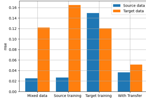
FIGURE 5.13 – Erreur quadratique moyenne du transfert C_0 \rightarrow C_3
