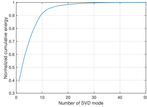
FIGURE 3.10 – Énergie cumulée de la SVD appliquée aux signaux temporels de la poutre
