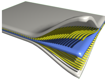
FIGURE 1.2 – Matériau composites avec la matrice et les renforts
