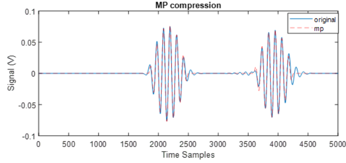
FIGURE 3.12 – Exemple d’une observation de la poutre compressée par MP avec deux paquets.
