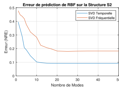
(c) Évolution de l'erreur de prédictions de la RBF sur les données de validation pour le domaine temporel et fréquentiel sur la structure S2
