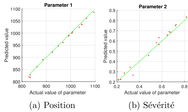
FIGURE 4.13 – Évaluation de la résolution inverse sur la poutre avec CNN temporel
