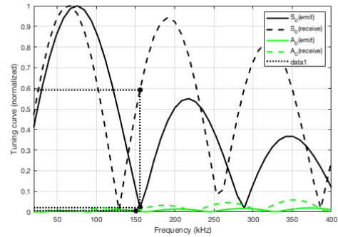
(d) Tuning Curves
