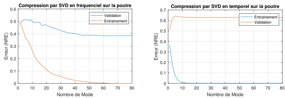
(a) SVD dans le domaine fréquentiel sur la poutre (b) SVD dans le domaine temporel sur la poutre
