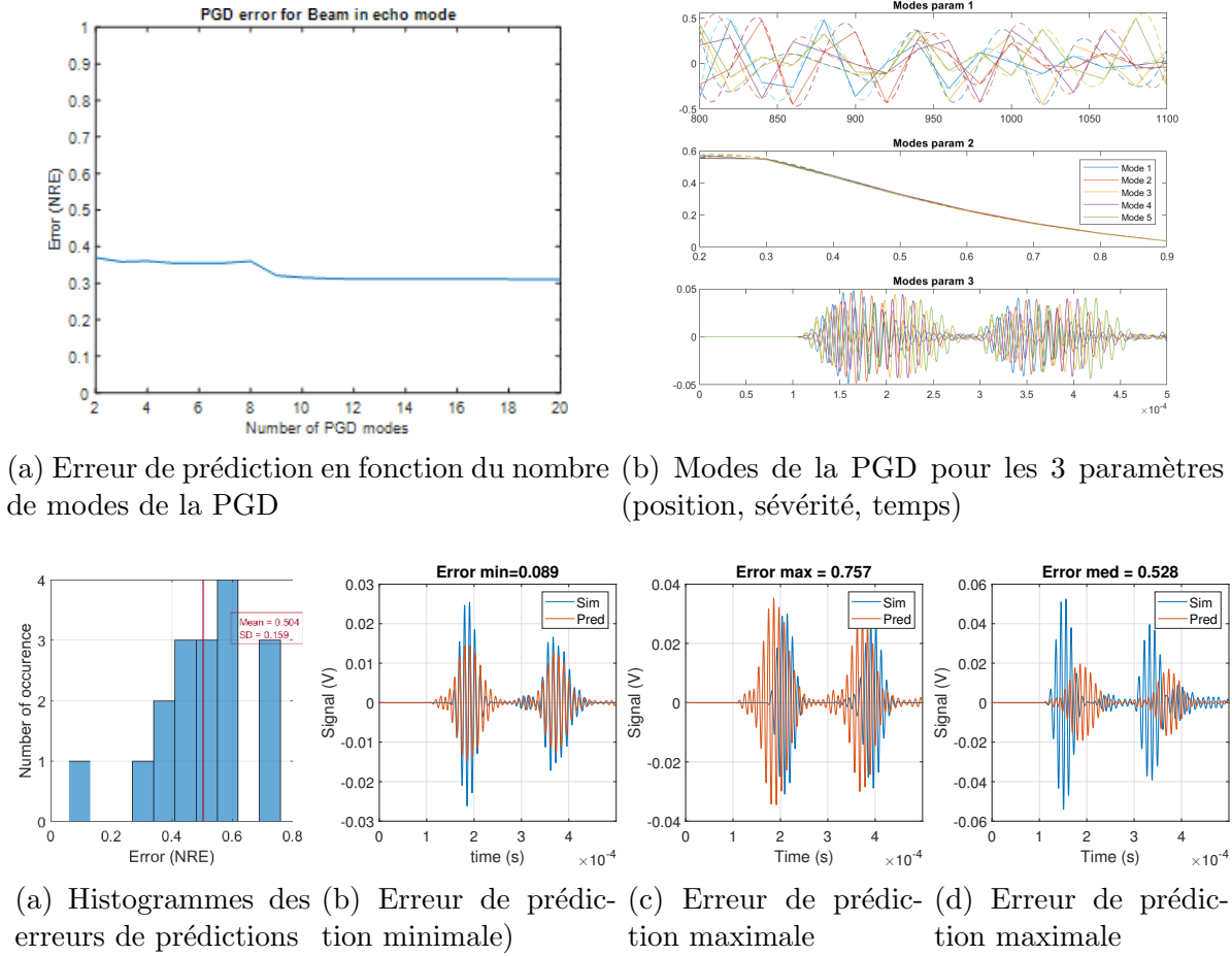
FIGURE 3.16 – Évaluation de la PGD sur la structure poutre
