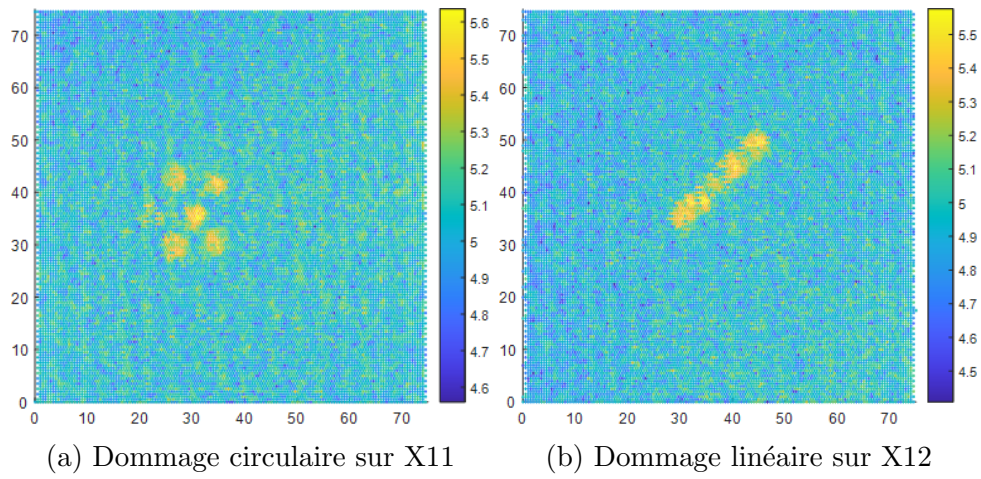
FIGURE 2.7 – C-SCAN des endommagements réalisés
