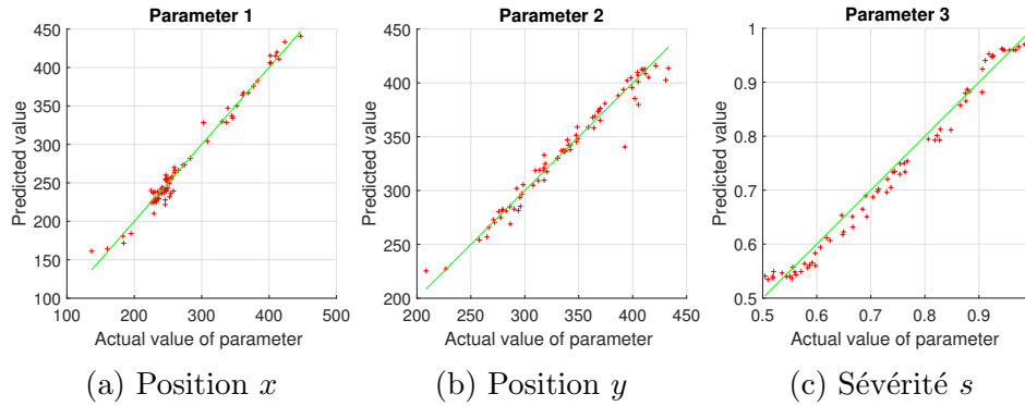
FIGURE 4.17 – Évaluation du CNN temporel sur le cas 2
