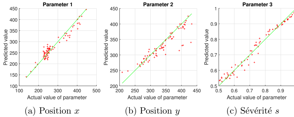
FIGURE 4.18 – Évaluation du CNN avec TVDI sur le cas 2
