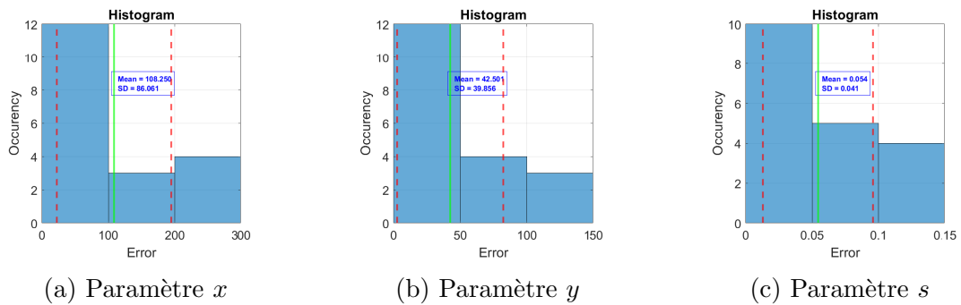
FIGURE C.3 – Histogrammes des erreurs de la résolution inverse sur S11 avec la RBF et SVD
