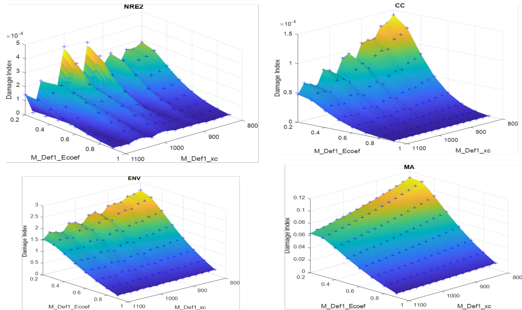
FIGURE 2.13 – DIs en fonction de la sévérité et de la position pour la poutre en réflexion (PZT 1 → PZT 1)
