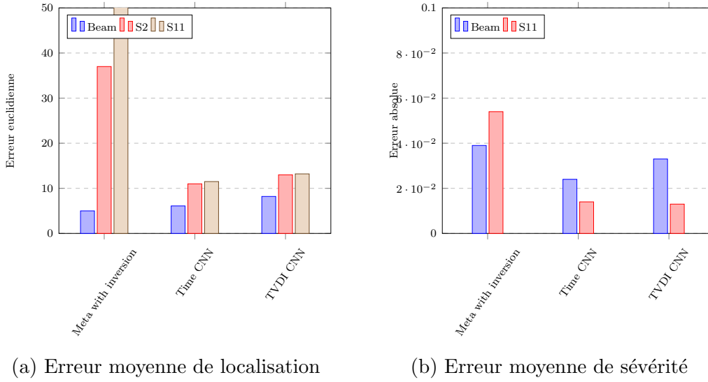
FIGURE 4.23 – Comparaison des méthodes de résolution inverse
