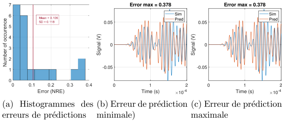
FIGURE B.4 – Évaluation du RBF avec SVD sur la structure S2
