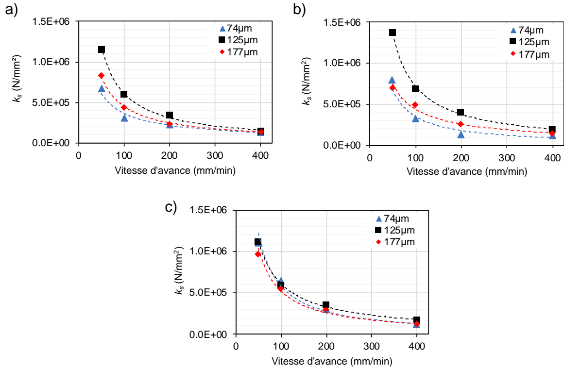
Figure 5.11 : Évolution de l'effort spécifique de coupe en fonction de la vitesse d'avance calculé d'après le modèle de Fekaier pour différents diamètres de particules abrasives. a) Q_a = 100 g/min ; b) Q_a = 150 g/min et c) Q_a = 200 g/min
