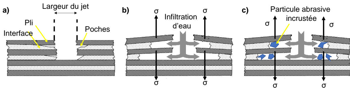
Figure 1.29 : Description du mécanisme de délaminage et d'incrustation des particules abrasives dans un matériau composite [154]: a) création de poches de délaminage par l'impact du jet, b) fragilisation des interfaces par le jet, c) incrustation des particules abrasives dans les poches de délaminage
