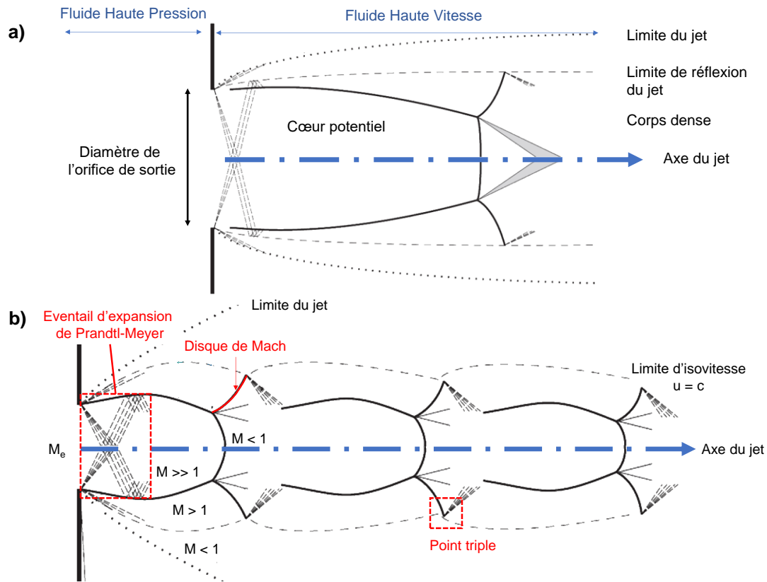
Figure 1.17 : Description schématique d'un jet sous-détendu : a) en sortie de buse; b) jet entier [113]
