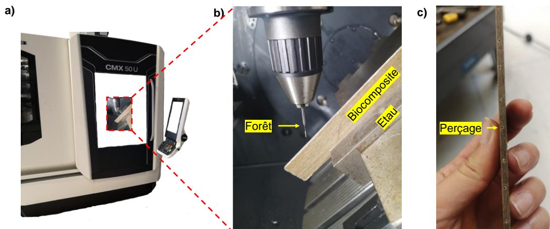
Figure 2.17 : Perçage des bandes d'agrocomposites à l'aide d'une machine à commandes numériques : Photographie de : a) la machine à commande numérique modèle CMX 50U ; b) banc de perçage monté sur la CMX ; c) Profil du biocomposite percé pour l'insertion des thermocouples lors des essais de découpe du Chapitre 5
