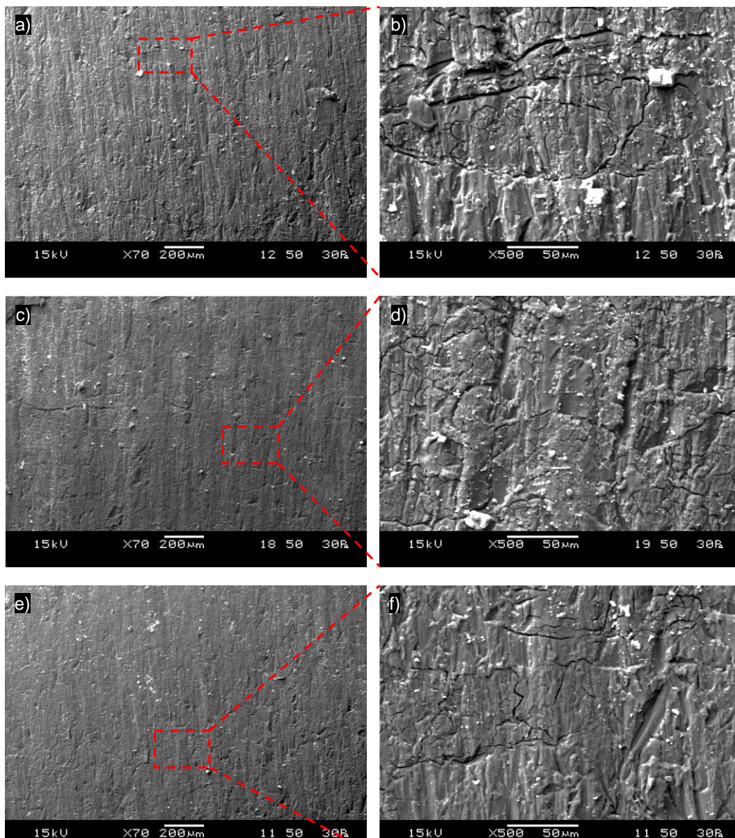
Figure 5.7 : Observations MEB réalisées au niveau de la zone médiane du profil usiné avec V_a = 50 mm/min et D_a = 74 μm en utilisant différentes de débit massique des particules à deux grossissements : a) et b) Q_a = 100 g/min, c) et d) Q_a = 150
