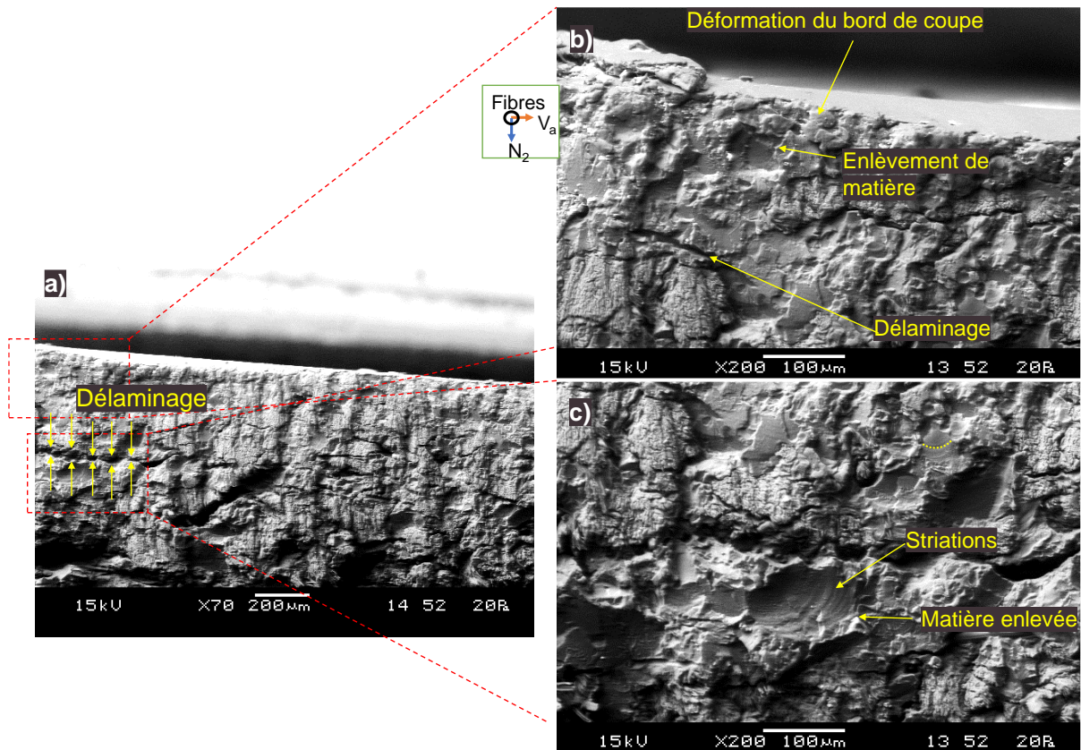
Figure 3.11 : Observation microscopique au M.E.B. de l'endommagement surfacique au J.A.C. pour P_{N_2} = 200 MPa et V_a = 50 mm/min a) à un grossissement x70 ; en agrandissant b) la zone d'endommagement initiale ; c) une zone de délaminage
