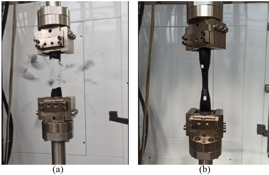
FIGURE 4 – a) Essai de traction-torsion pour le diabolo à HR0 ; b) Essai de traction-torsion pour le diabolo à HR50.
