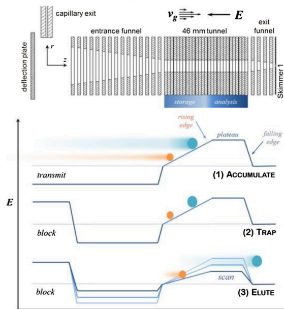
Figure 13 : Fonctionnement du TIMS. Haut : Les ions entrent dans un tunnel, poussés par un flux de gaz constant ( V_g ), et sont ralentis par un champ électrique E dont l'intensité augmente avec la distance parcourue. Bas : Dans un premier temps, dans l'état accumulation (accumulate), les ions entrent dans le tunnel et se stabilisent en fonction de leur mobilité. Dans un second temps, l'entrée d'autres ions est empêchée en imposant un fort champ électrique en entrée (état trap). Dans un troisième temps, l'intensité du champ électrique est progressivement diminuée, libérant les ions successivement suivant leur mobilité (état elute).
