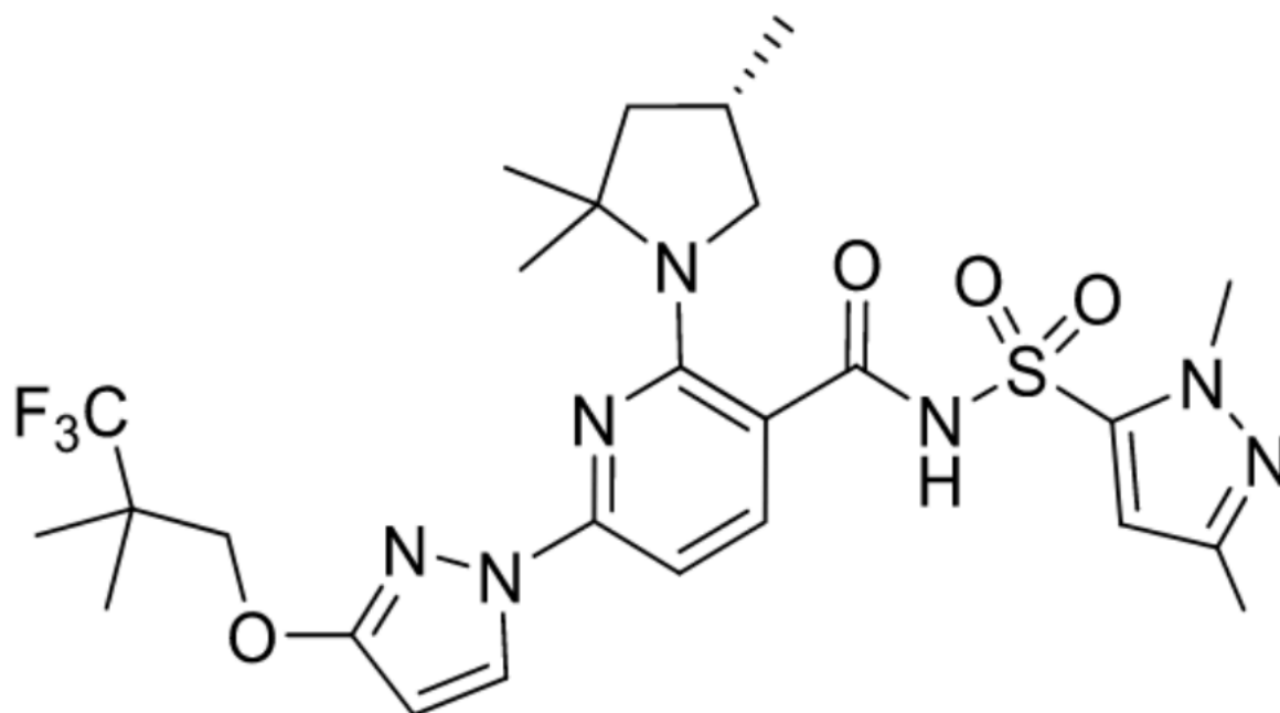
Figure 12 : Formule chimique du VX-445 (Elexacaftor) (Bardin 2021)
