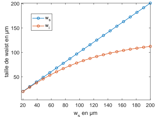
(b) Tailles de waist w_i et w_s en fonction de w_s
