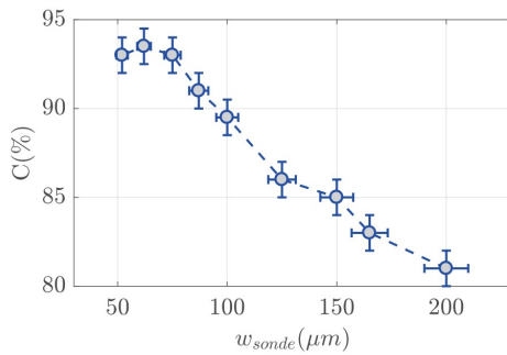
(a) Contraste entre l'idler et la sonde pour plusieurs w_s ; Provenance ; thèse de Martin Bouillard [Bou17]
