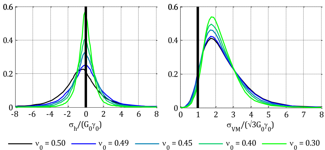
Figure 83 : Distribution des contraintes hydrostatique \sigma_h et équivalente \sigma_{VM} dans la matrice pour différentes compressibilités \nu_0
