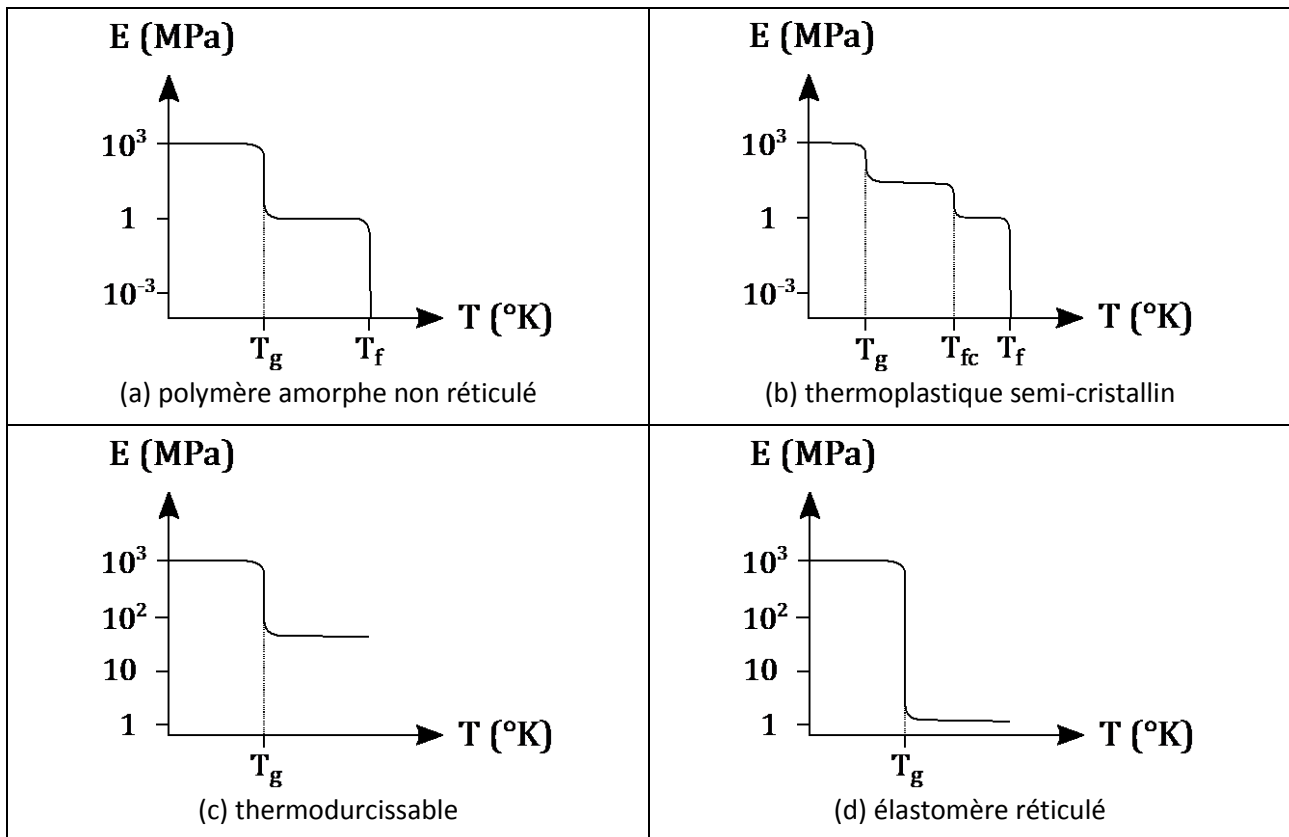
Figure 3 : Illustration de l'évolution de la rigidité des polymères selon leur catégorie
