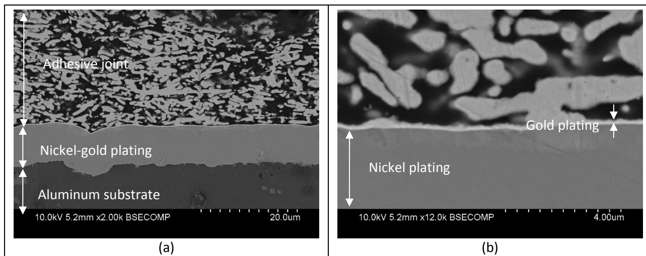
Figure 34 : Illustration du plaquage nickel-or sur les substrats des assemblage collés (l'image (b) est un zoom de l'image (a) montrant la finesse du dépôt d'or)
