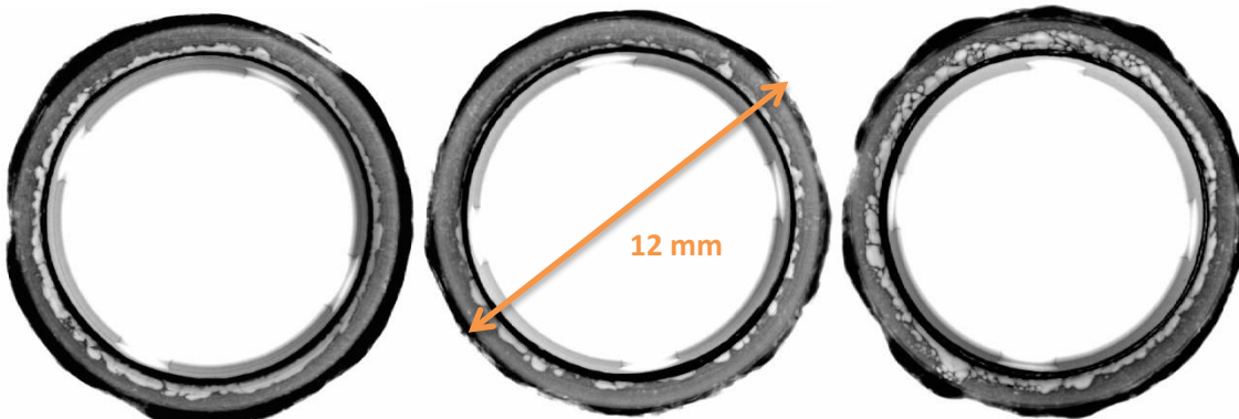
Figure 41 : Vues aux rayons X de 3 joints polyimide annulaires : les cavités sont regroupées au niveau du diamètre interne
