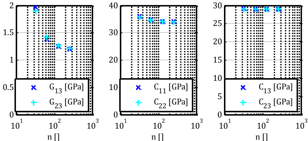
Figure 74: Evolution des coefficients du tenseur d'élasticité homogénéisé avec la discrétisation du VER
