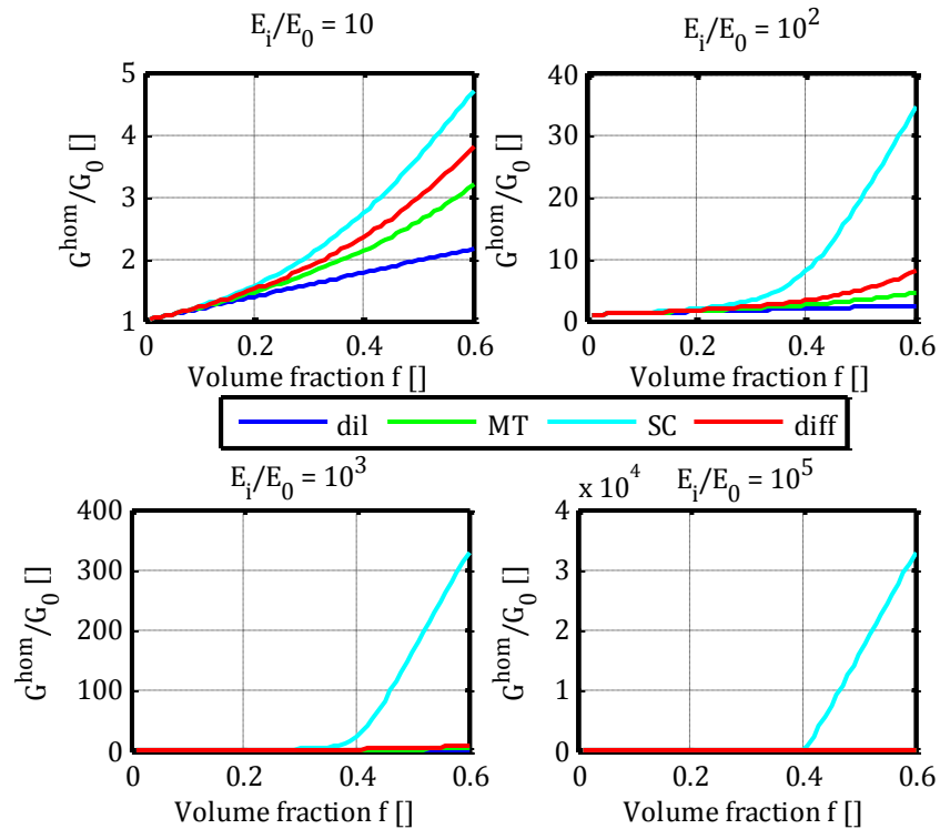
Figure 71 : Evolution du module de cisaillement homogénéisé normalisé G^{hom}/G_0 avec la fraction volumique de particules f pour les schémas dilué, Mori-Tanaka (MT), auto-cohérent (SC) et différentiel en fonction du contraste de rigidité matrice/particule E_i/E_0
