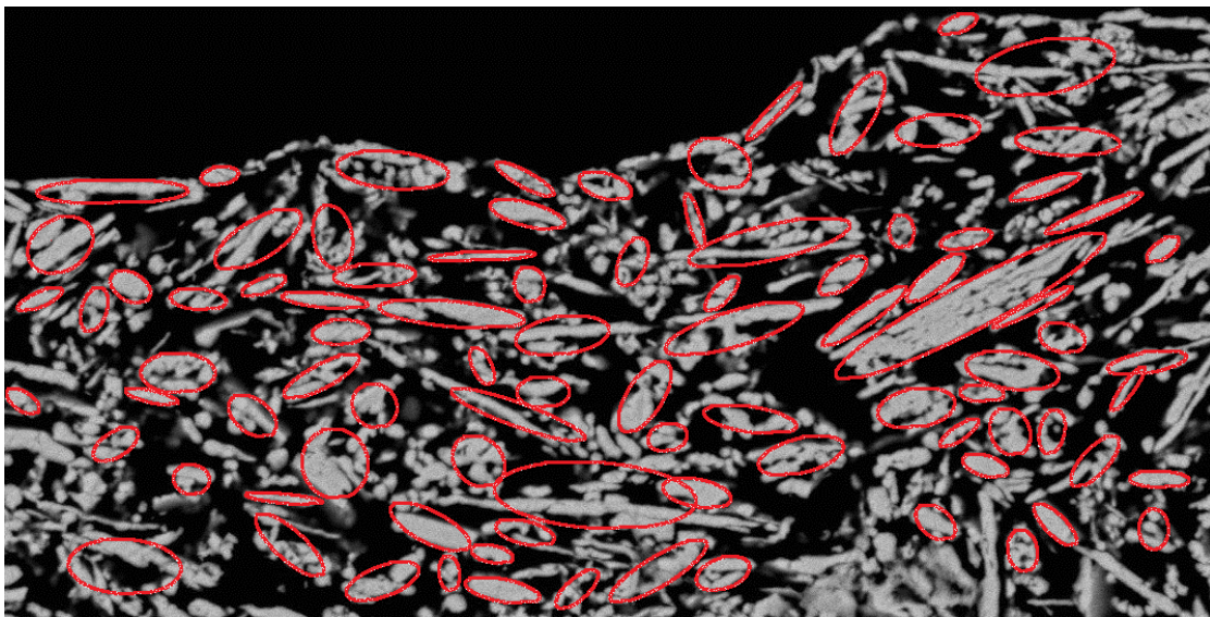
Figure 67 : Identification des particules dans le joint polyimide avec le logiciel Fiji
