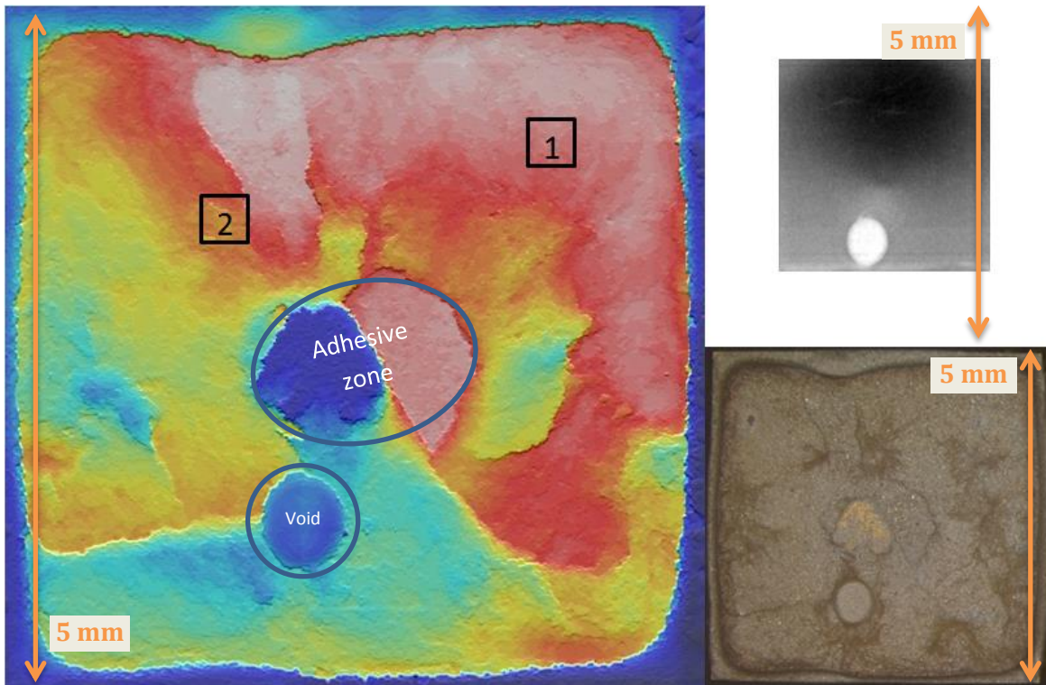
Figure 97 : Observation au profilomètre du faciès de rupture cohésif du joint silicone (le cliché optique est rappelé en bas à droite, le cliché rayons X en haut à droite). Une zone locale au milieu est identifiée comme adhésive, une autre en-dessous provient d'une cavité initialement présente dans le joint
