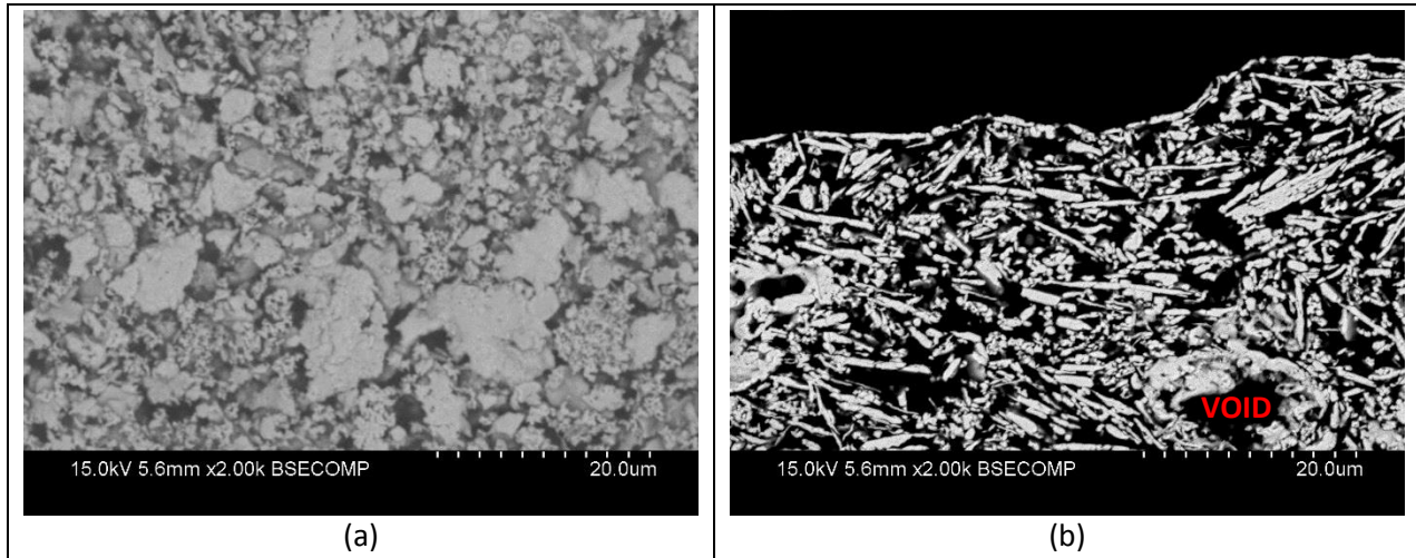
Figure 7 : Vue de dessus (a) et en coupe (b) d'un joint polyimide
