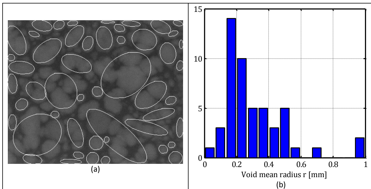
Figure 36 : (a) identification des cavités du joint polyimide par le logiciel Fiji ; (b) histogramme du rayon moyen des cavités
