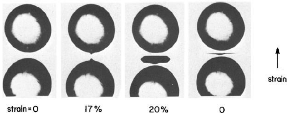
Figure 93 : cavitation entre deux particules alignées dans la direction de traction [92]
