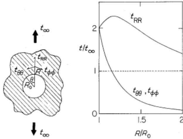
Figure 92 : Contraintes au voisinage d'une inclusion rigide de rayon R_0 en fonction de la distance R au centre de la particule dans la direction du chargement appliqué [101]
