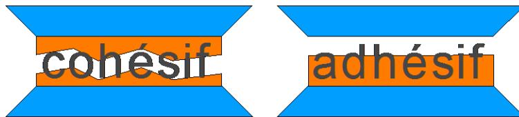
Figure 90 : Schématisation d'une rupture cohésive et d'une rupture adhésive
