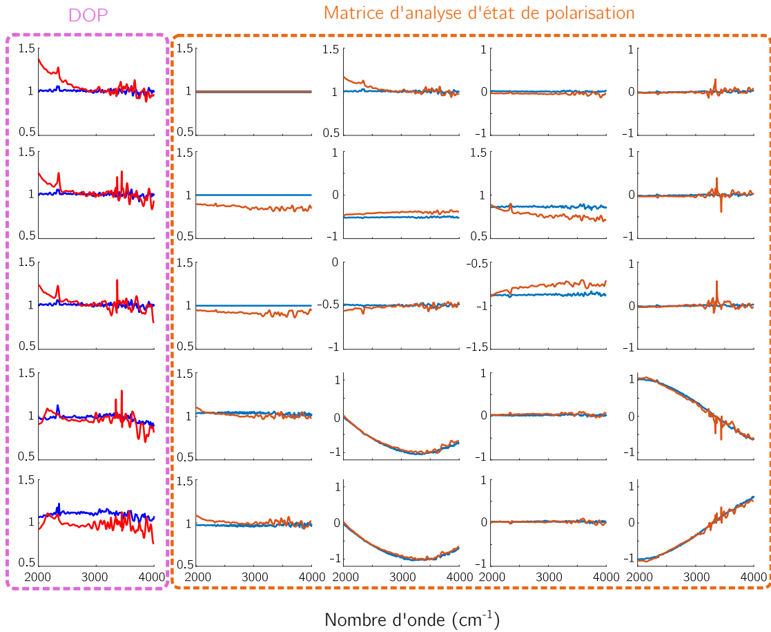
Figure 4.16 – (Encadré orange) Évolution spectrale des composantes de la matrice d'analyse d'état de polarisation \mathbf{W} pour un PSA en configuration bipyramide triangulaire. En bleu : reproduction des valeurs présentées en Fig.4.11. En orange : valeurs obtenues avec la méthode présentée en Eq.(4.32). (Encadré rose) Degré de polarisation (DOP) de chaque état correspondant du PSA figurant sur la même ligne. En bleu foncé : reproduction du DOP présenté en Fig.4.11. En rouge : DOP pour les états obtenus expérimentalement avec l'Eq.(4.32) (valeurs en orange sur la même ligne). L'ensemble des courbes sont tracées en fonction du nombre d'onde allant de 2000 à 4000 \text{cm}^{-1} .
