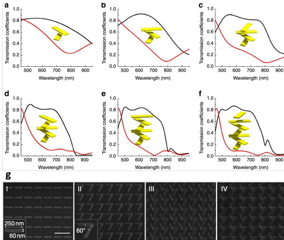
Figure 1.13 – a) Transmission d'une onde plane polarisée circulaire gauche (rouge) et droite (noir) à travers différents nombres de couches superposées composées de nanobâtonnets, proposé par [Zhao et al., 2012]. Chaque couche est une métasurface 2D de période 300 nm dans les deux directions dans le plan et composée de résonateurs en or de 55 nm d'épaisseur, de 250 nm de longueur et de 60 nm de largeur. Les couches sont séparées de 120 nm d'espaceur en \text{SiO}_2 et sont tournées relativement aux couches voisines de 60^\circ . a-f) Transmission à travers la structure lorsque le nombre de couches augmente de 2 à 7. g) Image MEB de 4 couches superposées. La barre d'échelle symbolise 500 nm.
