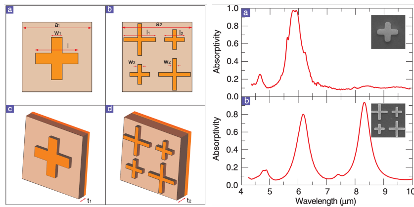
Figure 1.5 – a) Schéma de la cellule élémentaire d'une métasurface proposée par [Liu et al., 2011] optimisée pour une absorption sélective dans le MIR. b) Schéma de la cellule élémentaire d'une métasurface optimisée pour une absorption à sélective pour deux longueurs d'onde dans le MIR. c-d) Vue en perspective des cellules élémentaires précédentes. Un miroir métallique est déposé en-dessous de la métasurface, la séparation s'effectuant avec un espaceur.
