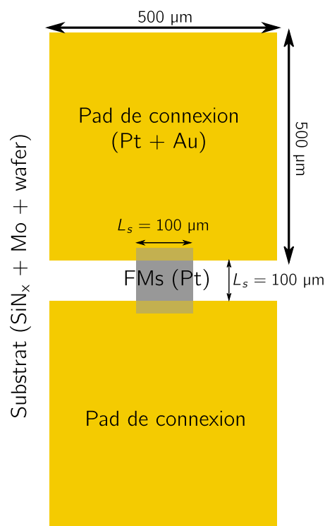
Figure 2.5 – Schéma d'une source avec ses pads de connexion. Les fils métalliques (FMs) sont verticaux dans cette orientation.
