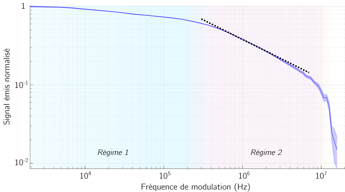
Figure 5.9 – Mesure expérimentale de la réponse en fréquence de la source représentée en Fig.5.2 en régime de modulation harmonique. On représente l'amplitude normalisée du signal modulé émis. Les barres d'erreur sont à 1\sigma . La courbe en pointillés noirs souligne la décroissance en f_{th}^{-1/2} .
