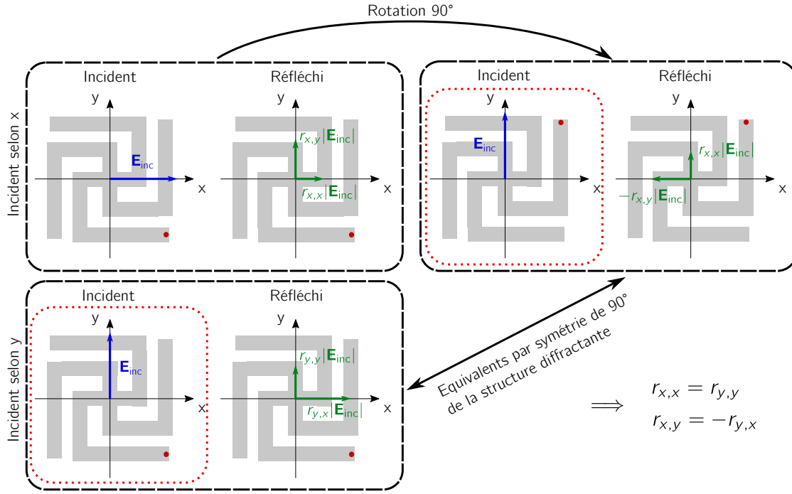
Figure 5.1 – Schéma justifiant l'absence de dichroïsme circulaire pour un réseau dont le motif élémentaire (motif grisé) présente une symétrie de rotation dans le plan de 90° autour de l'axe z. Ceci suppose que l'onde incidente arrive en incidence normale, que la transmission à travers le système est nul et qu'il n'y a réflexion que dans l'ordre 0. Le point rouge est purement symbolique et vise à faciliter la représentation visuelle de la rotation.
