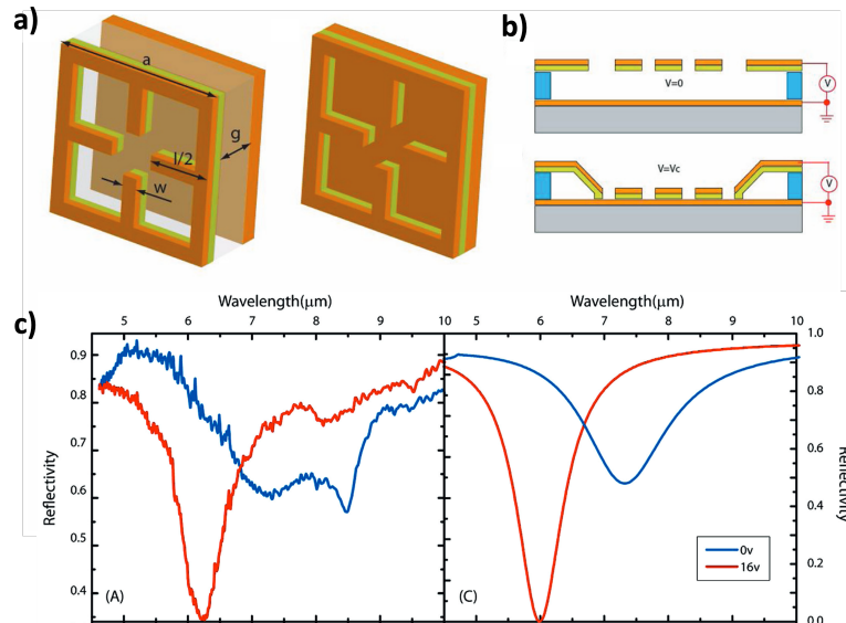
Figure 1.8 – a) Schéma d'une cellule élémentaire de la métasurface électromécanique proposée par [Liu and Padilla, 2013] en position de non-contact (à gauche) ou contact (à droite) avec le plan métallique inférieur. Les dimensions sont de a = 3.5 \mu\text{m} , l = 2.6 \mu\text{m} , w = 0.4 \mu\text{m} , g = 1.2 \mu\text{m} . Le plan métallique inférieur est considéré comme un miroir parfait à la longueur d'onde de travail, l'émetteur suspendu est constitué de 100 nm de métal déposé sur 280 nm de diélectrique. b) Schéma montrant le contrôle du contact de la source avec le plan métallique inférieur lorsqu'une tension est appliquée entre le métal émetteur et le miroir parfait sous-jacent. c) Spectre de réflectivité mesuré (gauche) et simulé (droite) pour la configuration contact (rouge) et non-contact (bleu).
