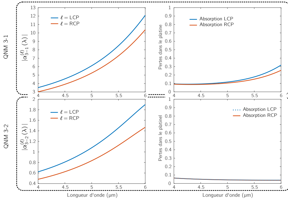
Figure C.2 – Colonne de gauche : Norme des coefficients d'excitation \alpha_X^{(\ell)}(\lambda) , X=3-1,3-2 étant le numéro du QNM identifié en Fig.5.16 et (\ell) la polarisation correspondante. Colonne de droite : Simulation du spectre d'absorption pour un unique QNM considéré. Ces QNMs sont une contribution minoritaire vers 5 \mu .
