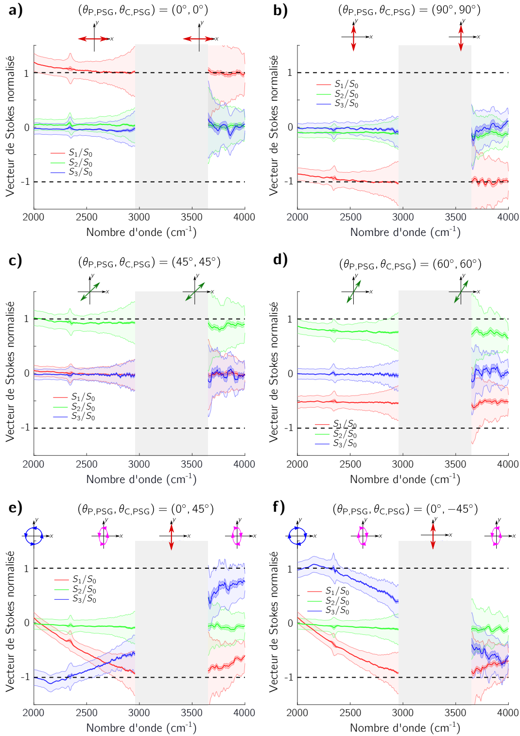
Figure 4.18 – Mesure du vecteur de Stokes normalisé pour plusieurs états de polarisation connus en entrée du PSA bipyramidal triangulaire présenté. Les états en entrée sont générés par un générateur d'état de polarisation constitué d'un polariseur linéaire suivi d'une lame à retard en \text{MgF}_2 quart d'onde à 2000 \text{cm}^{-1} . Leurs orientations respectives par rapport à une référence commune sont notées au-dessus de chacun des panneaux et les états de polarisation générés y sont également schématisés. a-d) : états de polarisation linéaires en entrée. e-f) : états de polarisation elliptiques devenant circulaires à 2000 \text{cm}^{-1} . La zone entre 3000-3650 \text{cm}^{-1} est en-dehors de la plage de fonctionnement du PSA. La ligne centrale fine représente la valeur estimée par pseudo-inversion pour le vecteur de Stokes. Les zones colorées plus foncées autour des lignes centrales représentent les barres d'erreur à 1\sigma estimées par la matrice de covariance (Eq.(4.26)). Les zones colorées plus claires et plus larges représentent les barres d'erreur estimées par l'Eq.(4.21) pour \|\Delta\mathbf{W}\|/\|\mathbf{W}\| = 0.03 .
