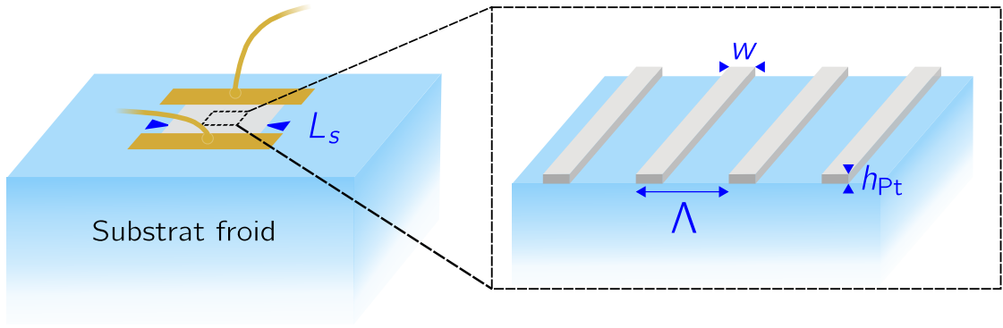
Figure 3.1 – Famille de source incandescente à modulation de température pour laquelle nous cherchons à optimiser le rendement.
