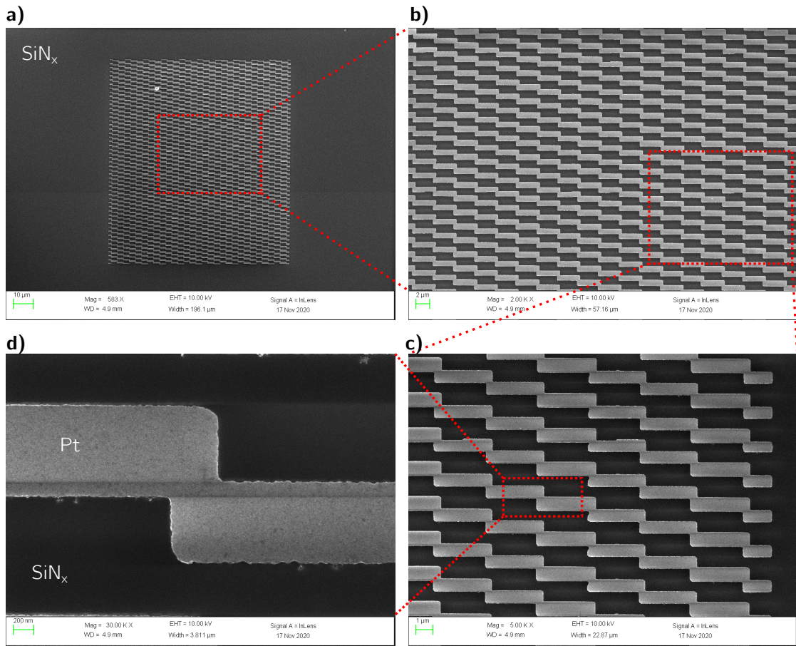
Figure 5.5 – Images de la source au microscope à balayage électronique à différents grossissements (croissants dans l'ordre alphabétique). Les échelles de longueur sont symbolisées par le trait vert en bas à gauche de chaque image MEB a) 10 \mu\text{m} , b) 2 \mu\text{m} , c) 1 \mu\text{m} , d) 200 nm).
