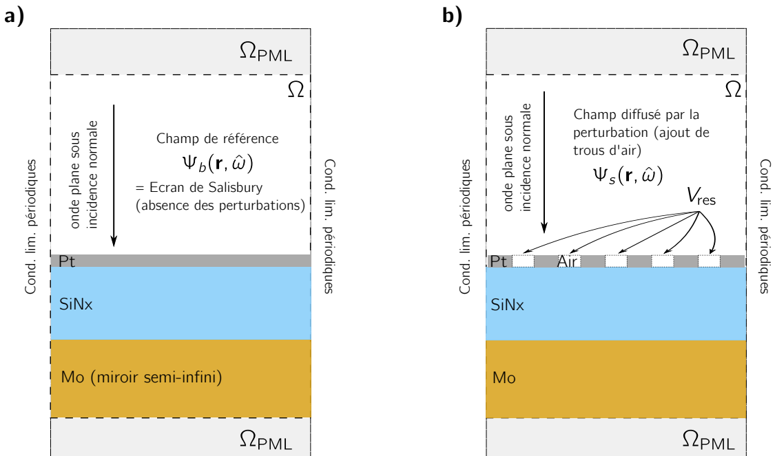
Figure 5.15 – Calcul du champ de référence \Psi_b = [\mathbf{E}_b, \mathbf{H}_b] . La situation de référence est un simple écran de Salisbury excité par une onde plane sous incidence normale. b) Ajout des perturbations par rapport à la situation de référence. On s'intéresse aux champs diffusés du fait de l'ajout de ces perturbations \Psi_s = [\mathbf{E}_s, \mathbf{H}_s] .
