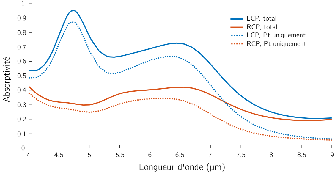
Figure 5.3 – Simulation du spectre d'absorption de la source dans son ensemble, éclairée par une onde plane de polarisation circulaire gauche (bleu, trait plein) et droite (orange, trait plein) sous incidence normale. On trace en traits pointillés dans une couleur identique l'absorption ayant lieu uniquement dans la métasurface en platine.
