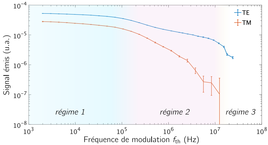
Figure 2.10 – Réponse en fréquence de la source en fonction de la fréquence de modulation thermique f_{th} = \omega_{th}/(2\pi) = 2f_{elec} . Bien que les valeurs en ordonnées soient représentées en unités arbitraires, les acquisitions représentant les puissances émises polarisées linéairement TE et TM à un même facteur de proportionalité près, sont faites dans les mêmes conditions expérimentales et les valeurs tracées peuvent donc être comparées relativement l'une à l'autre. Les barres d'erreur représentent l'écart type des valeurs expérimentales obtenues pour chaque fréquence de modulation.
