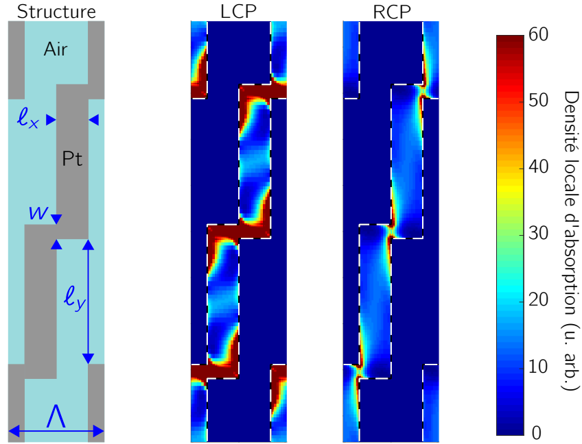
Figure 5.14 – Gauche : schéma de la couche dans laquelle l'absorption locale est calculée (au milieu de la couche de platine). Droite : densité locale d'absorption \frac{\pi}{\lambda_0} \epsilon_0 c \operatorname{Im} [\epsilon(\mathbf{r}, \lambda_0)] |\mathbf{E}^{(\ell)}(\mathbf{r}, \lambda_0)|^2 dans structure schématisée à gauche lorsque le réseau est éclairé avec une onde plane polarisée circulaire gauche (LCP) et droite (RCP). L'échelle de couleurs est la même pour les deux cartes et la valeur est en unité arbitraire.
