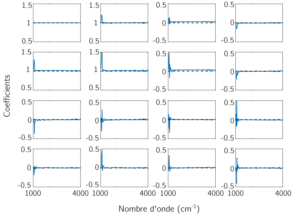
Figure 4.9 – Évolution spectrale des coefficients de la matrice de Mueller du polariseur utilisé dans le PSA construit. Les mesures sont faites en utilisant un polarimètre de Mueller. L'ensemble des courbes sont tracées entre 1000 et 4000 \text{cm}^{-1} . Les lignes tiretées en noir représentent les valeurs théoriques attendues pour un polariseur parfait.
