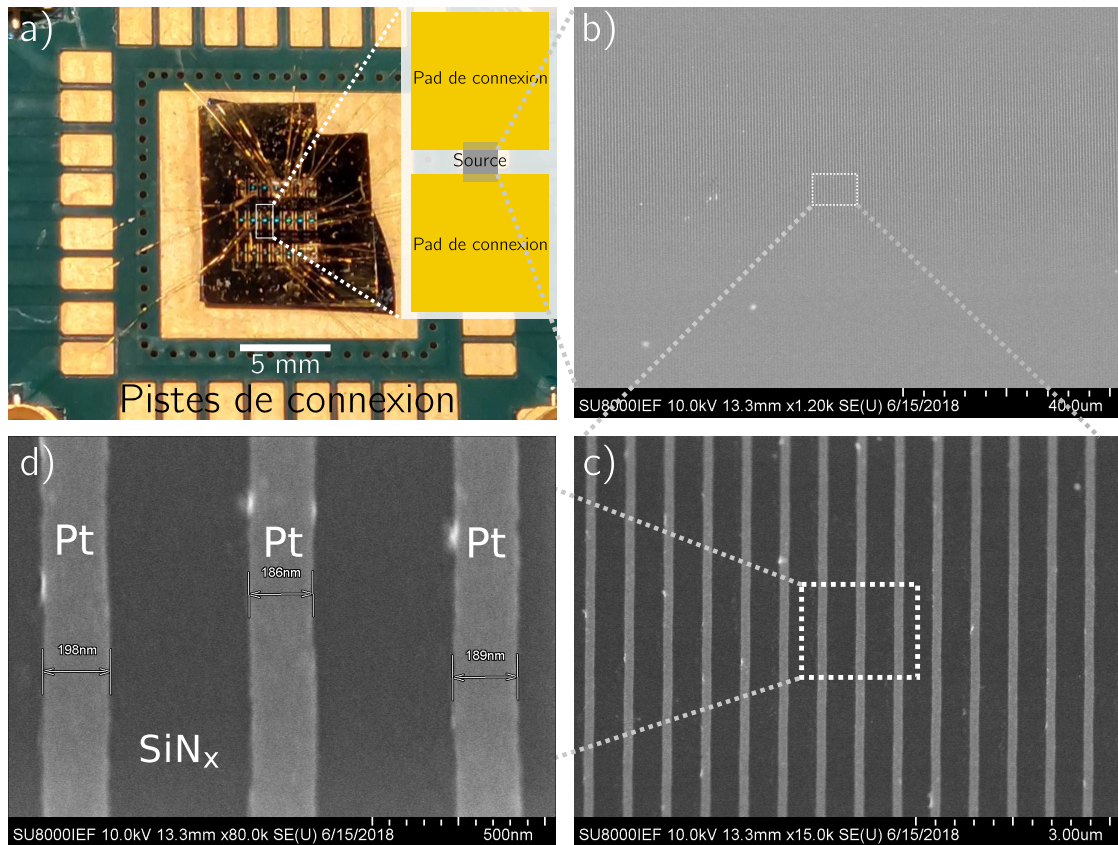
Figure 2.6 – a) Photographie du wafer contenant une dizaine de sources. Les fils métalliques qu'on aperçoit, connectant l'échantillon aux pistes de connexion, sont en or et ont été posés par wire bonding. b,c,d) Images MEB des fils métalliques à différents grossissements.
