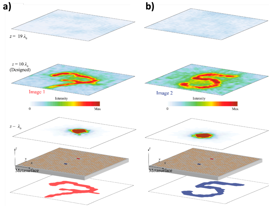
Figure 1.6 – a-b) Schémas d'une métasurface incandescente proposée par [Zhou et al., 2021] constituée de résonateurs (métalliques ou en SiC) carrés produisant des hologrammes variables. La longueur d'onde de travail est de \lambda_0 = 10 \mu\text{m} et la métasurface fait 10\lambda_0 \times 10\lambda_0 . Les résonateurs sont espacés de 0.4\lambda_0 . Lorsqu'on ne chauffe sélectivement que le résonateur en rouge ( a) ), la métasurface projette le chiffre 7 dans un plan situé 10\lambda_0 au-dessus de la métasurface. Lorsque l'émetteur bleu uniquement est chauffé, c'est le chiffre 5 qui est cette fois projeté dans le même plan.
