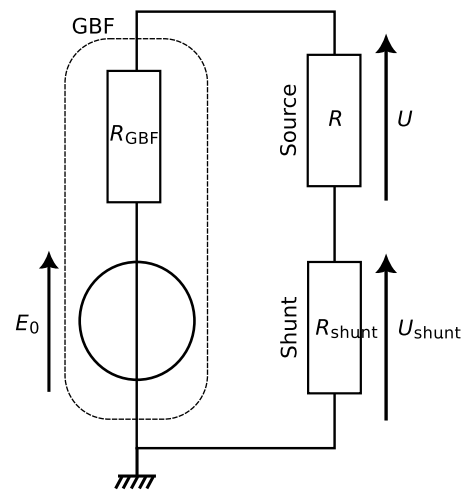
Figure 2.14 – Dispositif de mesure de résistance électrique de notre source.
