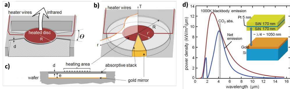
Figure 1.4 – a) Schéma d'une membrane suspendue typiquement utilisée pour la détection infrarouge. b) Schéma de la source incandescente proposée par [Brucoli et al., 2014] à base de membrane suspendue par deux bras de chauffage au-dessus d'un miroir d'or. c) Schéma en coupe de la source incandescente proposée. d) Structure optimisée pour émettre à 4.26 \mu\text{m} . La courbe rouge représente le spectre d'émission d'un corps noir à 1000 K et la courbe bleue le spectre émis par la structure schématisée à droite lorsque le platine est chauffé à 1000 K.
