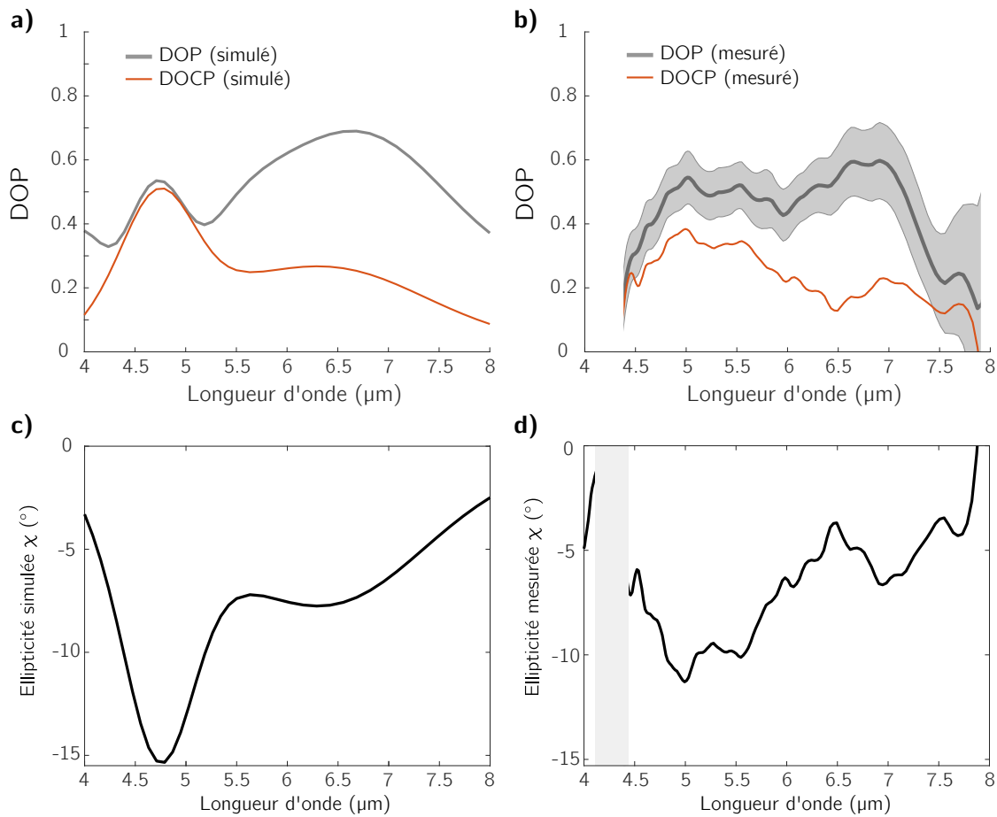
Figure 5.13 – Degré de polarisation (DOP, gris) et degré de polarisation circulaire (DOCP, orange) du rayonnement émis a) simulé b) déduit de la mesure expérimentale des paramètres de Stokes. Les barres d'erreur sont à 1\sigma . La gamme spectrale entre 4 et 4.4 \mu\text{m} n'est pas représentée à cause de l'absorption du \text{CO}_2 . c) Ellipticité simulée et d) ellipticité mesurée.
