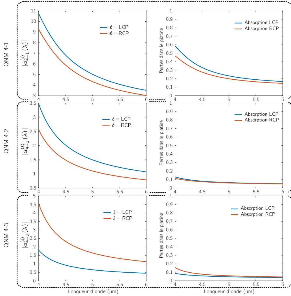
Figure C.3 – Colonne de gauche : Norme des coefficients d'excitation \alpha_X^{(\ell)}(\lambda) , X=4-1, 4-2, 4-3 étant le numéro du QNM identifié en Fig. 5.16 et (\ell) la polarisation correspondante. Colonne de droite : Simulation du spectre d'absorption pour un unique QNM considéré. Ces QNMs sont une contribution minoritaire vers 5 \mu .
