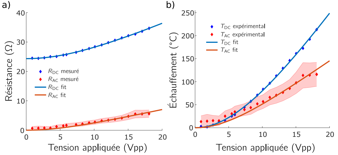
Figure 2.15 – Mesure a) de la résistance et b) de l'échauffement des FMs pour différentes tensions appliquées. La tension appliquée aux bornes de la source est une sinusoïde pure oscillant à 10 kHz. Les points représentent les mesures expérimentales et la zone en couleur représente les barres d'erreur à 1\sigma . Les courbes en traits pleins sont les ajustements effectués selon les Eqs.(2.32), (2.36), (2.30) et (2.37).
