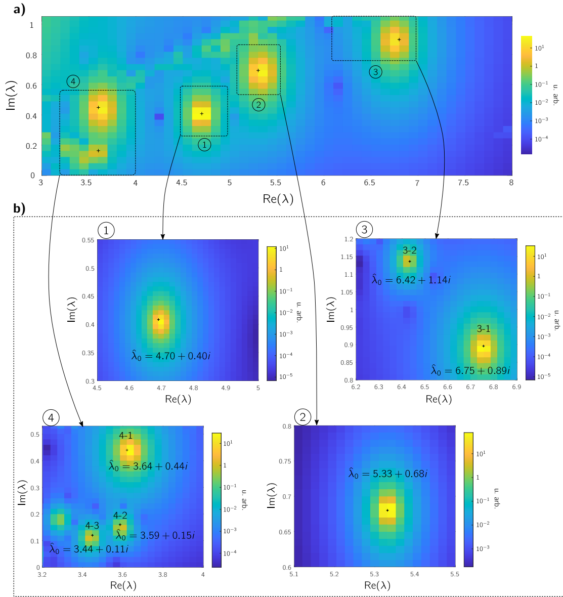
Figure 5.16 – Recherche des pôles du déterminant de la matrice de scattering, les longueurs d'onde sont exprimées en \mu\text{m} . a) On trace en couleur le \log_{10} de l'intégrale de Cauchy estimée grossièrement sur le contour des rectangles élémentaires définis par le maillage dans le plan complexe. Ce calcul permet d'obtenir une valeur approximative des pôles au maillage près (symbolisée par une croix noire), correspondant à une divergence du déterminant de la matrice de scattering. b) Affinage du maillage et recherche des zéros de l'inverse du déterminant de la matrice de scattering. Ces derniers sont numérotés ①,②,③-①,③-② et ④-①,④-②,④-③ et la valeur correspondante est notée en-dessous de chaque estimation.
