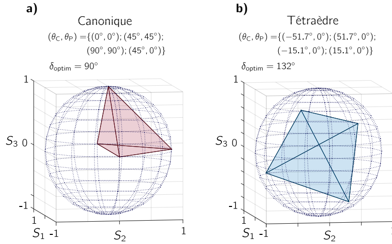
Figure 4.2 – Polyèdres à 4 sommets inscrits dans la sphère de Poincaré représentant les PSA à M = 4 états présentés en Sec.4.2.1 pour leur retard optimal respectif : a) ensemble canonique à 4 états, b) tétraèdre régulier (spherical 2-design pour M = 4 ).
