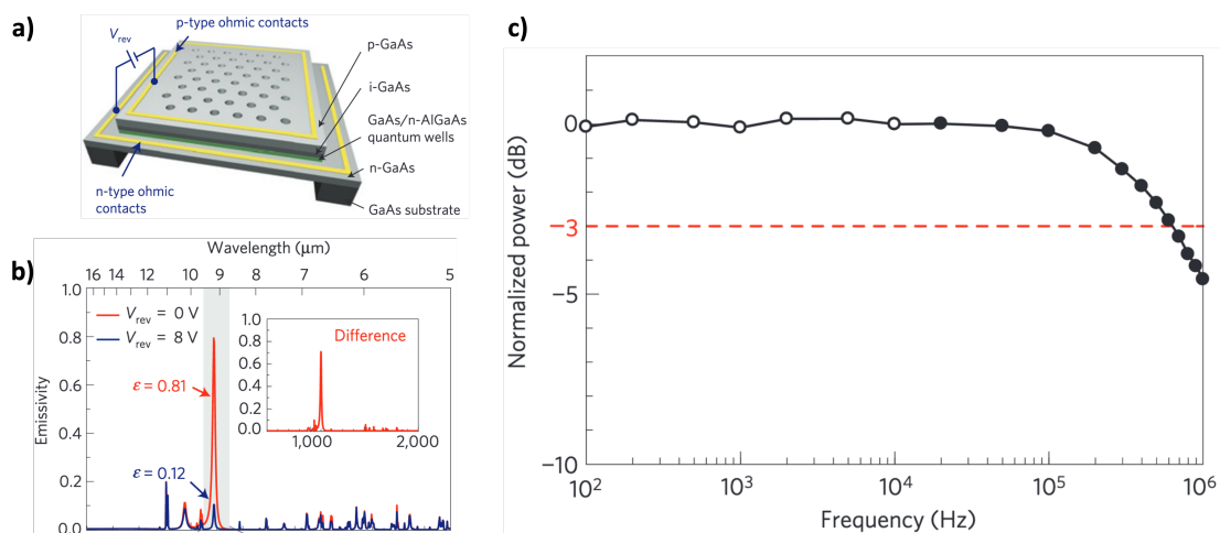
Figure 1.9 – a) Schéma du dispositif proposé par [Inoue et al., 2014]. b) Spectre d'émissivité calculé pour différentes tensions appliquées aux bornes de leur source. c) Réponse en fréquence de leur source incandescente. Le trait pointillé symbolise la coupure à 3 dB atteinte à 600 kHz.
