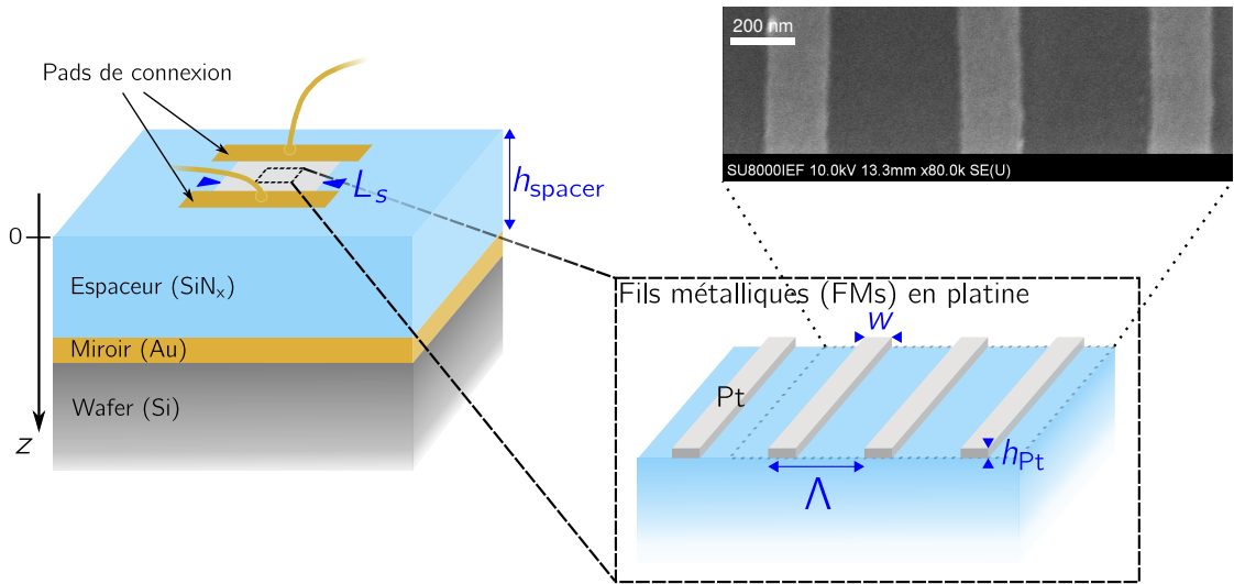
Figure 2.3 – Architecture finale de la source MIR à modulation rapide.
