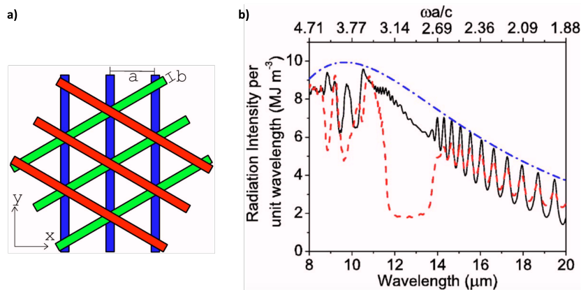
Figure 1.18 – a) Schéma du cristal photonique à bandgap sensible à l'hélicité de la polarisation proposé par [Lee and Chan, 2007]. Les couleurs symbolisent chacun des réseaux 1D orientés à 0^\circ , 60^\circ et 120^\circ . Ces réseaux sont constitués de fils en matériau diélectrique. b) Simulations du spectre émis par la source à 300 K en incidence normale, lorsqu'un miroir parfait est placé sous le cristal photonique. En pointillés bleus : le spectre de corps noir. En noir : la luminance polarisée circulaire gauche émise par la source. En bleu : la luminance polarisée circulaire droite émise par la source.
