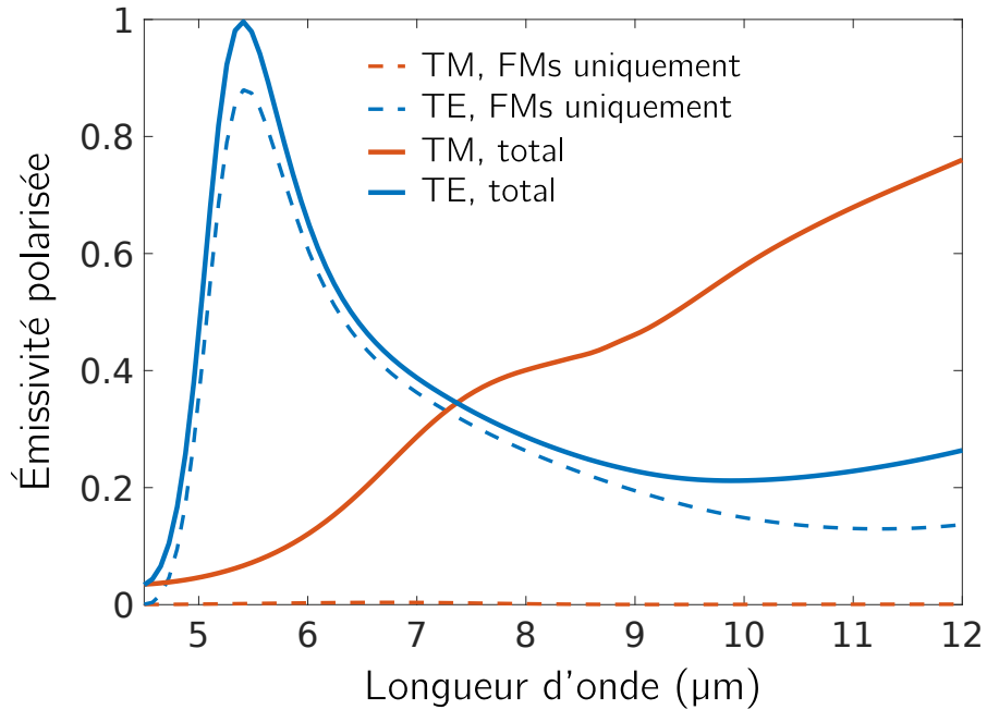
Figure 2.4 – Simulations de l'émissivité spectrale. En traits pleins l'absorption totale de la structure (FMs + substrat). En traits pointillés l'absorption due uniquement aux FMs. De cette simulation, on peut légitimement considérer que \eta^{(TM)}(\lambda) = 0 dans la zone spectrale d'intérêt.
