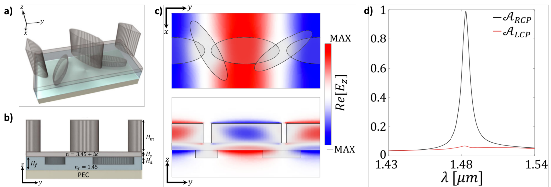
Figure 1.16 – a) Schéma en perspective du méta-atome constituant la métasurface incandescente proposée par [Overvig et al., 2021]. Le film en silicium est texturé en forme de pilier elliptique posé sur un substrat diélectrique. Le schéma montre l'exemple de deux couches de métamatériaux empilées. b) Schéma de la vue en coupe. c) Représentation de la partie réelle du champ électrique projeté sur la normale à la surface. On voit un mode BIC supporté par la structure. d) Spectre d'absorption de la structure lorsqu'elle est éclairée avec une onde plane polarisée circulaire gauche ou droite. La simulation montre un rayonnement thermique quasi parfaitement polarisé circulairement.
