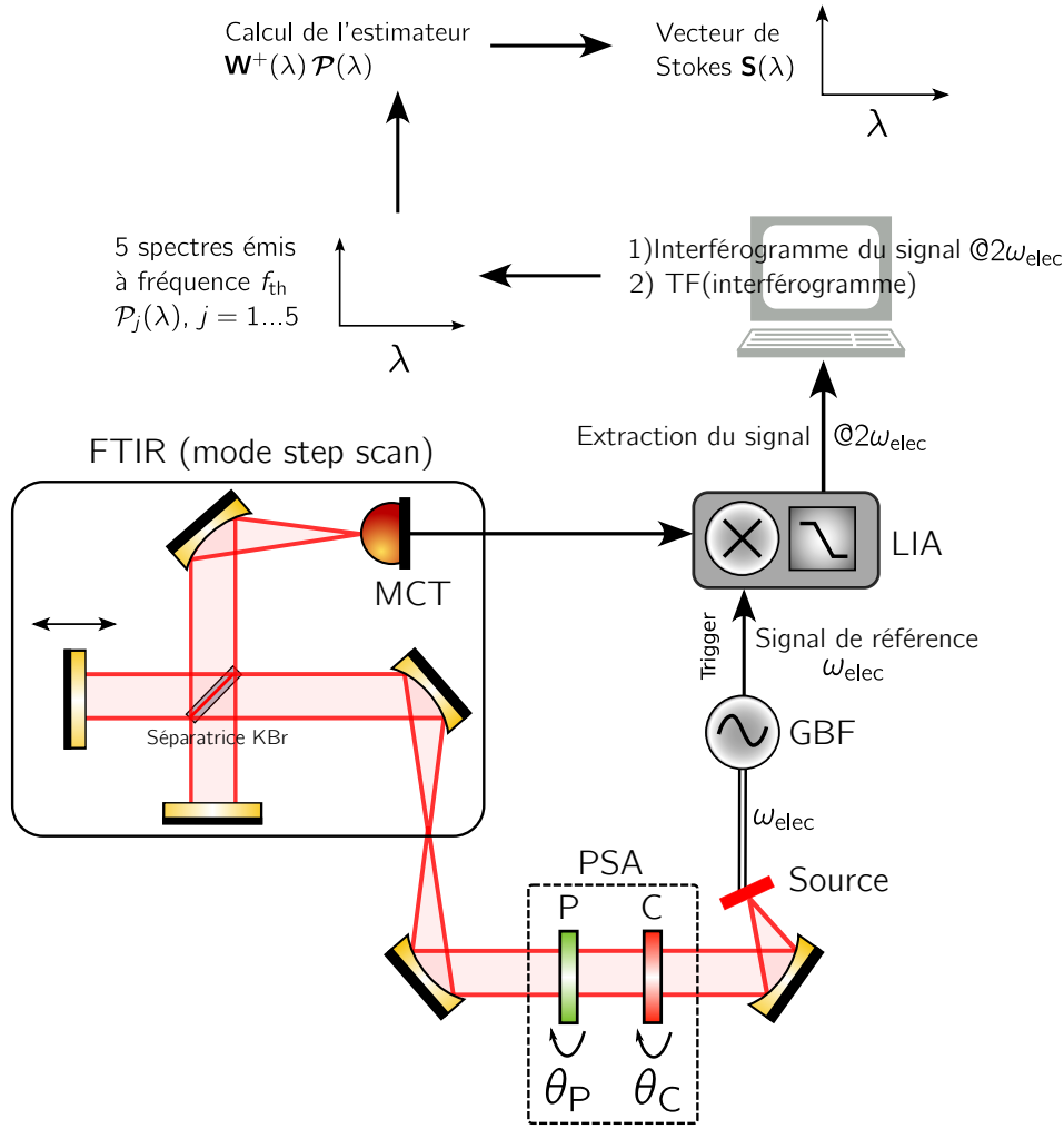
Figure 5.11 – Dispositif expérimental de mesure de l'état de polarisation du rayonnement émis par la source en régime de fonctionnement modulé.
