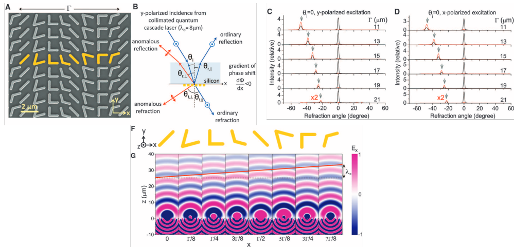
Figure 1.2 – a) Image MEB de la métasurface proposée par [Yu et al., 2011]. La cellule élémentaire de l'interface plasmonique est représentée en jaune et consiste en 8 antennes en forme de "V" en or avec une largeur de bras d'environ 220 nm et une épaisseur de 50 nm. La période en x vaut \Gamma = 11 \mu\text{m} et la période selon y est de 1.5 \mu\text{m} . La longueur d'onde de travail est à 8 \mu\text{m} . b) Schéma de l'expérience pour une excitation avec une onde plane avec un champ électrique selon y . c,d) Intensités mesurées en champ lointain dues à la réfraction sur la métasurface lorsqu'elle est éclairée avec une onde polarisée selon y et x respectivement. L'angle est pris par rapport à la normale à la surface. Les spectres sont montrés pour 6 échantillons différents se différenciant par la période en x . f) Schéma de la cellule élémentaire de la métasurface. Les antennes sont conçues pour avoir des amplitudes diffusées égales et une différence de phase constante de \pi/4 entre voisins. g) Simulations du champ électrique polarisé selon x et diffusé par chacune des antennes de la cellule élémentaire présentée en f) . Les antennes sont excitées avec une onde plane polarisée selon y et arrivant sous incidence normale à la surface de l'échantillon. La ligne oblique en pointillés rouges représente l'enveloppe des ondes sphériques diffusées par l'ensemble des antennes, projetée sur le plan x - z .
