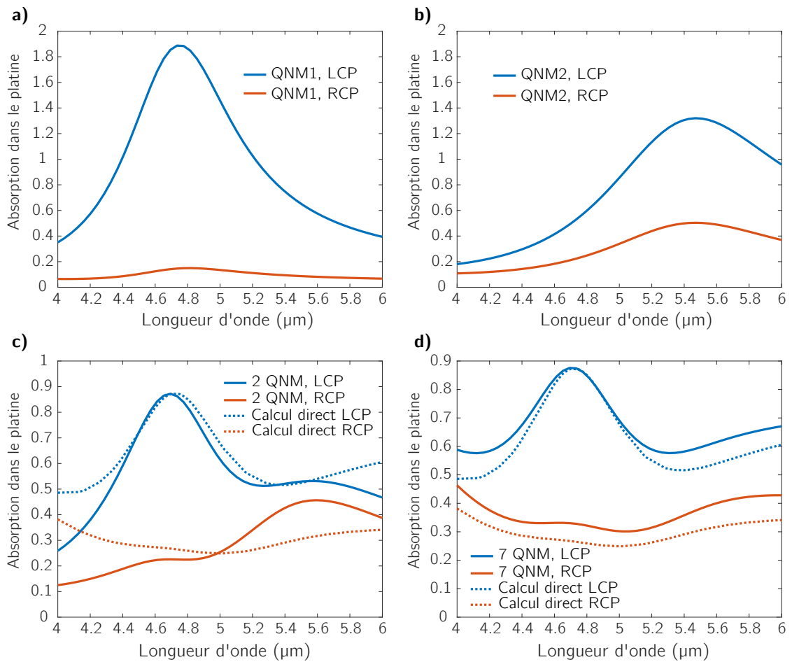
Figure 5.17 – Simulation du spectre d’absorption dans le platine lorsque l’échantillon est éclairé sous incidence normale avec une onde plane polarisée circulaire gauche (LCP) ou droite (RCP) en tronquant le champ à quelques QNMs. On garde en a) uniquement le QNM1, en b) uniquement le QNM2, en c) les QNM1 et QNM2 seulement et en d) les 7 QNMs identifiés en Fig.5.16. L’absorption peut dépasser 1 lorsqu’on ne considère pas l’interférence de suffisamment de QNMs de la structure.
