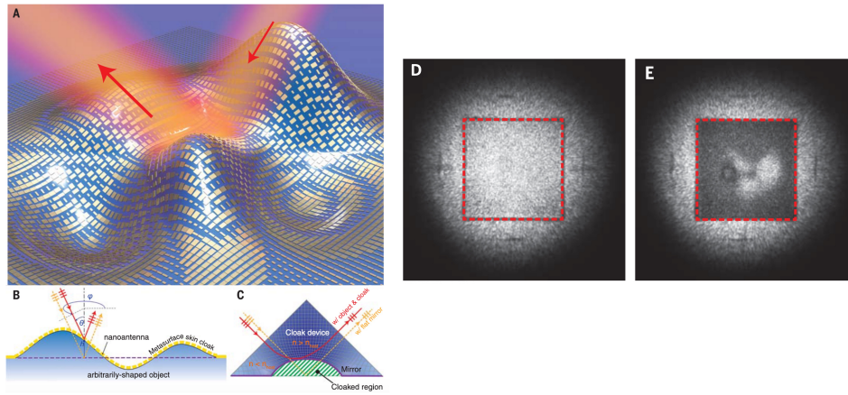
Figure 1.1 – a) Illustration d'une cape d'invisibilité à base d'une métasurface constituée de nanoantennes en or recouvrant un objet arbitraire que l'on souhaite cacher, repris de [Ni et al., 2015]. b) Vue en coupe de la métasurface. c) Schéma explicatif de l'effet de la métasurface sur la diffraction d'une onde incidente sur l'objet à cacher. d-e) Image en réflexion observée au microscope optique de l'objet à cacher, situé dans la zone entourée en rouge d) lorsque cet objet est recouvert par la métasurface e) en l'absence de métasurface.
