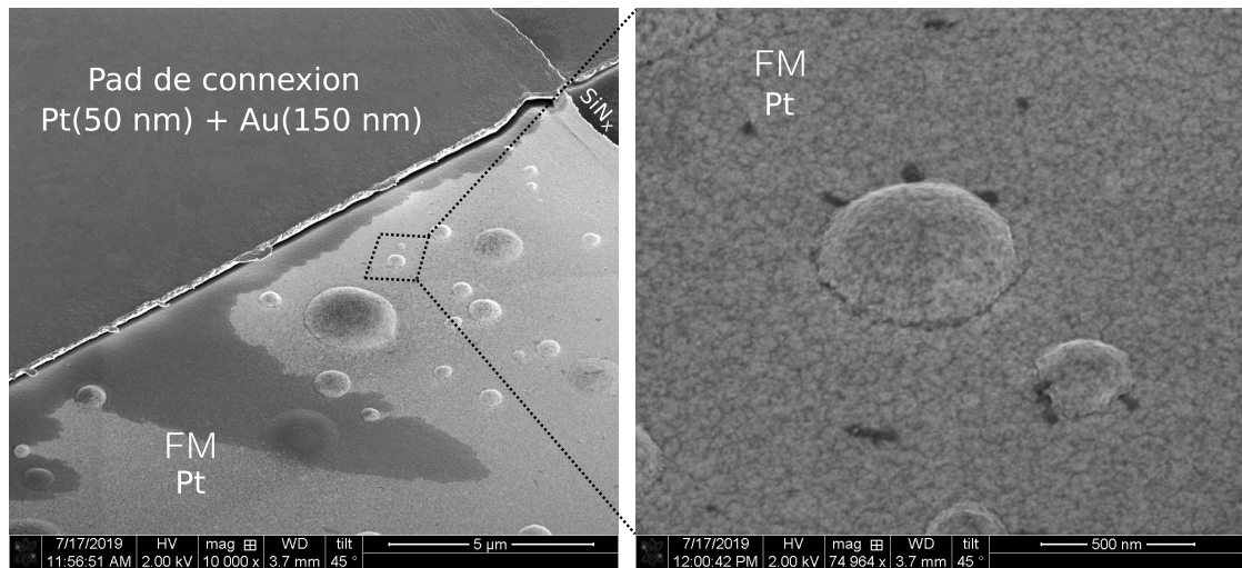
Figure 2.7 – Image MEB à fort grossissement d'un fil métallique après l'avoir mis sous tension pendant plusieurs heures. On peut voir le développement de bulles sous le platine, dues au dégazage du \text{SiN}_x lorsque ce dernier est chauffé.
