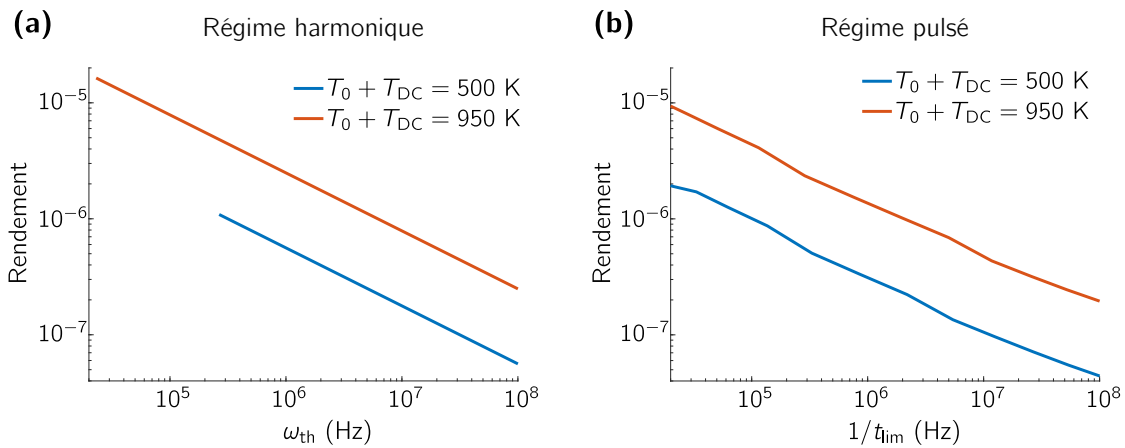
Figure 3.3 – Régime de fonctionnement linéaire. Rendement de la source incandescente à modulation de température en fonction de sa fréquence de modulation \omega_{th} (a) pour un régime harmonique décrit en Eq.(3.22) avec U_0 = 20V et T_0 + T_{DC} = 500, 950 K – la courbe à 500 K est tronquée pour de faibles fréquences pour garantir \Delta T < T_{DC} – et (b) pour un régime pulsé décrit en Eq.(3.21) tracé en fonction de 1/t_{lim} pour U_0 = 20 V et pour T_0 + T_{DC} = 500, 950K .
