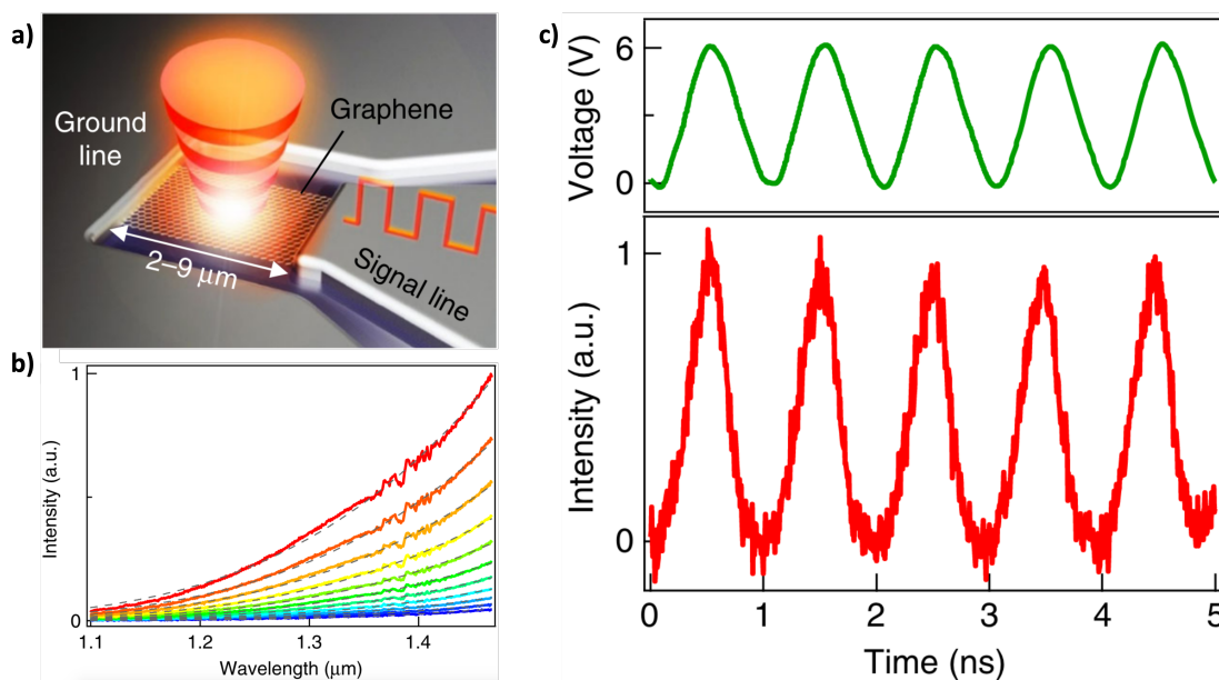
Figure 1.10 – a) Schéma de la source à incandescence proposée par [Miyoshi et al., 2018] à base de quelques feuillets voir monocouche de graphène. b) Luminance mesurée expérimentalement pour différentes températures (plus la température est élevée, plus la couleur est proche du rouge). Les températures atteintes dans les feuillets de graphène sont comprises entre 600°C et 750°C. Les courbes en pointillés sont les ajustements des mesures expérimentales par une loi de Planck. c) Modulation de la source par application d'une tension sinusoïdale (en vert) et mesure de la modulation de l'émission de l'échantillon (en rouge) démontrant une modulation à 1 GHz.
