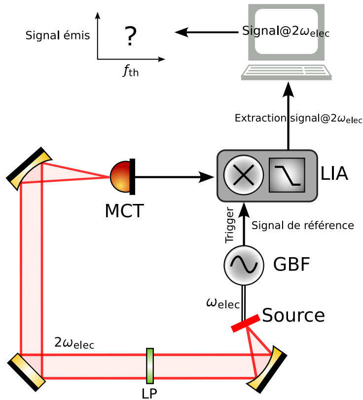
Figure 2.9 – Schéma du dispositif expérimental pour la caractérisation de la réponse en fréquence de la source. LP : polariseur linéaire dans le MIR.
