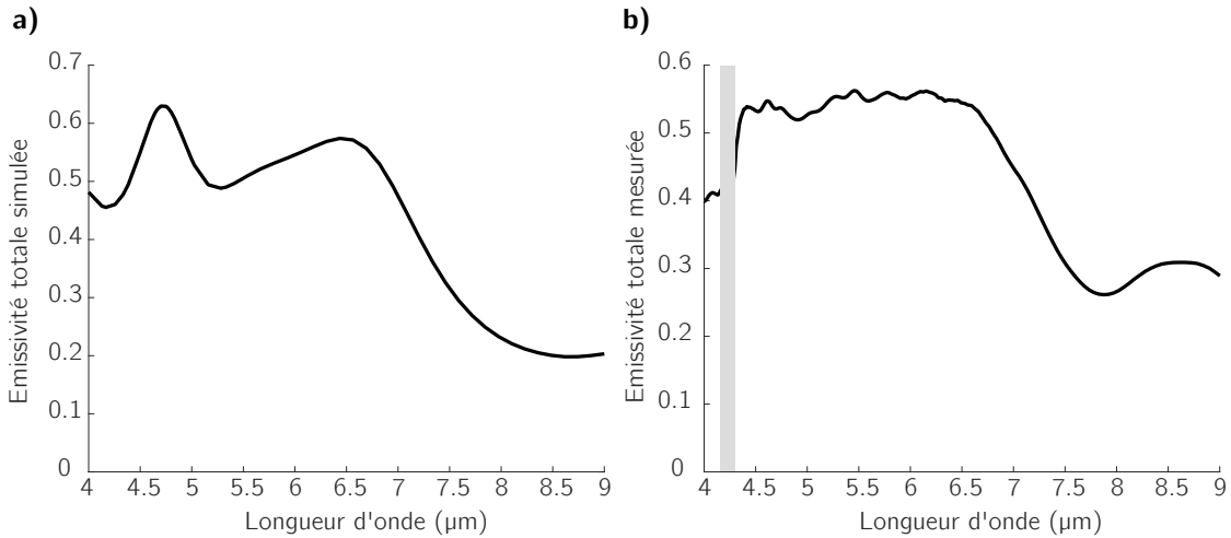
Figure 5.10 – Émissivité totale, moyenne des émissivités de polarisations croisées, a) simulée b) mesurée expérimentalement. En b) , les valeurs expérimentales ont été normalisées de façon à ce que l'émissivité à 4.7 μm prenne la même valeur que prédite par les simulations.
