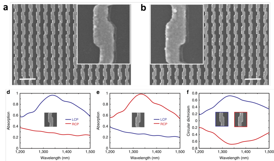
Figure 1.14 – a-b) Image MEB des structures métalliques chirales proposées par [Li et al., 2015] pour absorber sélectivement selon l'hélicité de la polarisation circulaire dans le NIR. La barre blanche indique 500 nm. Des métasurfaces énantiomères sont fabriquées et caractérisées en absorption en d) et e) respectivement. Le dichroïsme circulaire simulé et mesuré expérimentalement sont présentés en f) .
