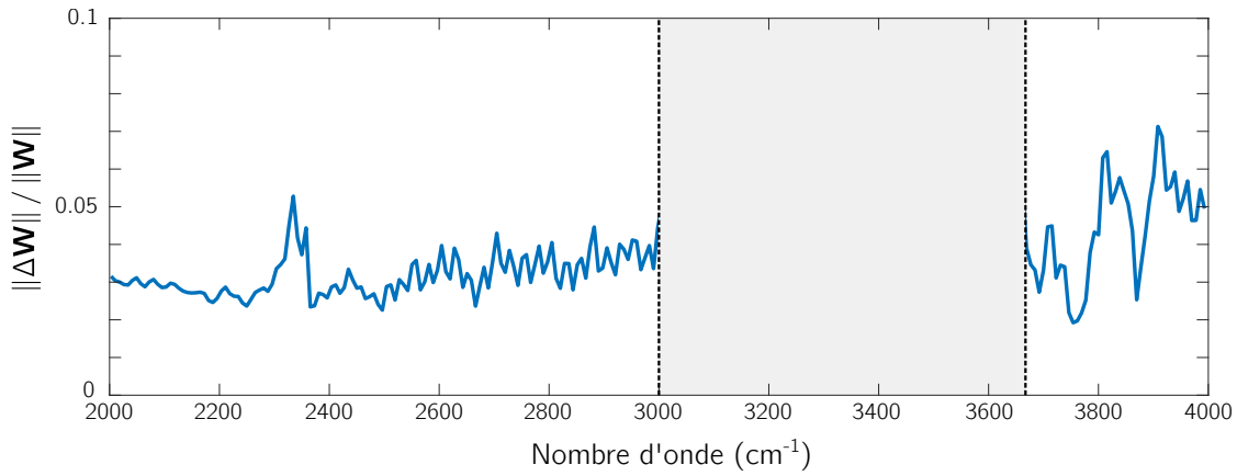
Figure 4.17 – Estimation de \|\Delta\mathbf{W}\|/\|\mathbf{W}\| sur la plage spectrale de fonctionnement du PSA.
