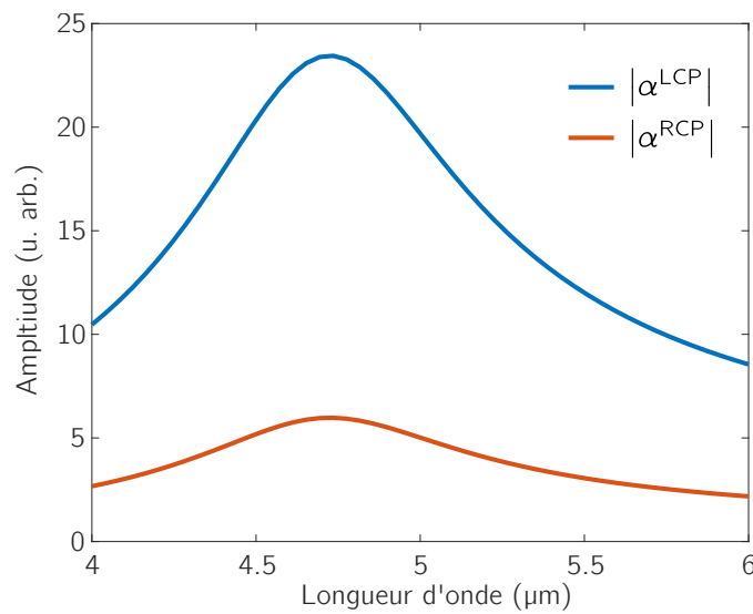
Figure 5.18 – Norme des coefficients d'excitation du QNM1 par une onde plane en incidence normale polarisée circulaire LCP (bleu) et RCP (rouge). L'amplitude du coefficient d'excitation LCP est 5 fois plus important que pour le RCP d'où l'absorption préférentielle d'une polarisation LCP par la structure (Fig.5.3 et Fig.5.17a).
