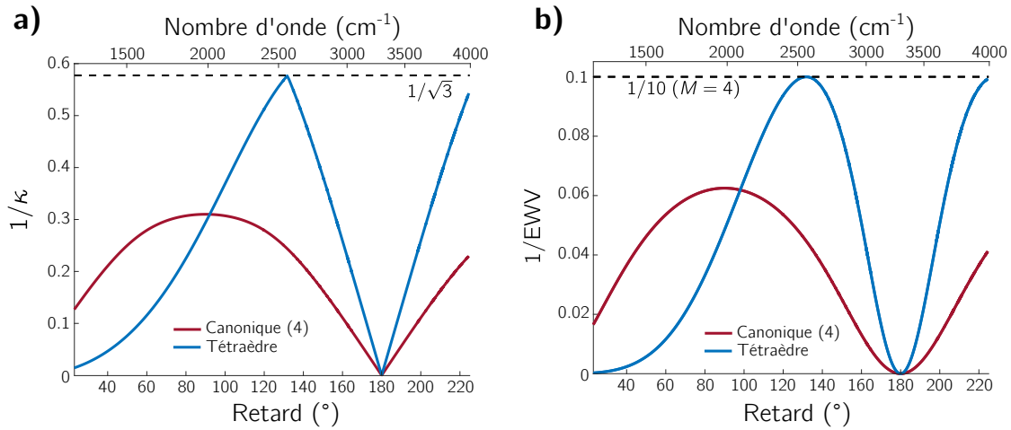
Figure 4.3 – Comparaison des figures de mérites : a) l'inverse du nombre de condition sur \mathbf{W} et b) l'inverse de l'EWV pour un PSA constitué d'une lame en \text{MgF}_2 , quart d'onde à 2000 \text{ cm}^{-1} , suivi d'un polariseur linéaire. Dans les deux figures, nous représentons la configuration d'un ensemble canonique à 4 états (rouge) et du tétraèdre (4 états, bleu). Dans a) , la ligne en pointillés à 1/\sqrt{3} représente le nombre de condition optimal qui peut être atteint ([Tyo, 2000]). En b) , la ligne en pointillés à 1/10 représente l'inverse du EWV minimal atteignable pour un PSA à M = 4 états ([Foreman and Goudail, 2019]).
