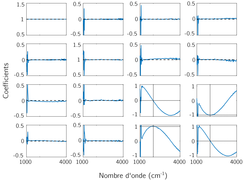
Figure 4.10 – Évolution spectrale des coefficients de la matrice de Mueller du retardateur utilisé dans le PSA construit. Cette lame à retard est quart d'onde à 2000 \text{ cm}^{-1} . Les mesures sont faites en utilisant un polarimètre de Mueller. L'ensemble des courbes sont tracées entre 1000 et 4000 \text{ cm}^{-1} . Les tirets noirs dans l'ensemble des panneaux, exceptés les quatre en bas à droite, représentent les courbes attendues pour un retardateur parfait. Les quatre panneaux restants représentent les \cos[\delta(\lambda)] et \pm \sin[\delta(\lambda)] . On trace en pointillés la longueur d'onde à laquelle le retard vaut \delta = 90^\circ , i.e. où la lame à retard devient quart d'onde.
