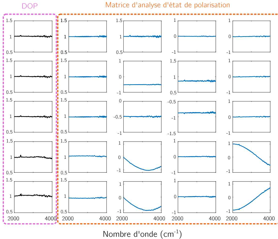
Figure 4.11 – (Encadré orange) Évolution spectrale des composantes de la matrice d'analyse d'état de polarisation \mathbf{W} pour un PSA en configuration bipyramide triangulaire. Les valeurs sont obtenues en utilisant l'Eq.(4.28) où les matrices de Mueller du polariseur et de la lame à retard ont été mesurées avec un polarimètre de Mueller. (Encadré rose) Degré de polarisation (DOP) de chaque état correspondant du PSA figurant sur la même ligne, calculé avec l'Eq.(4.28). L'ensemble des courbes sont tracées en fonction du nombre d'onde allant de 2000 à 4000 \text{cm}^{-1} .
