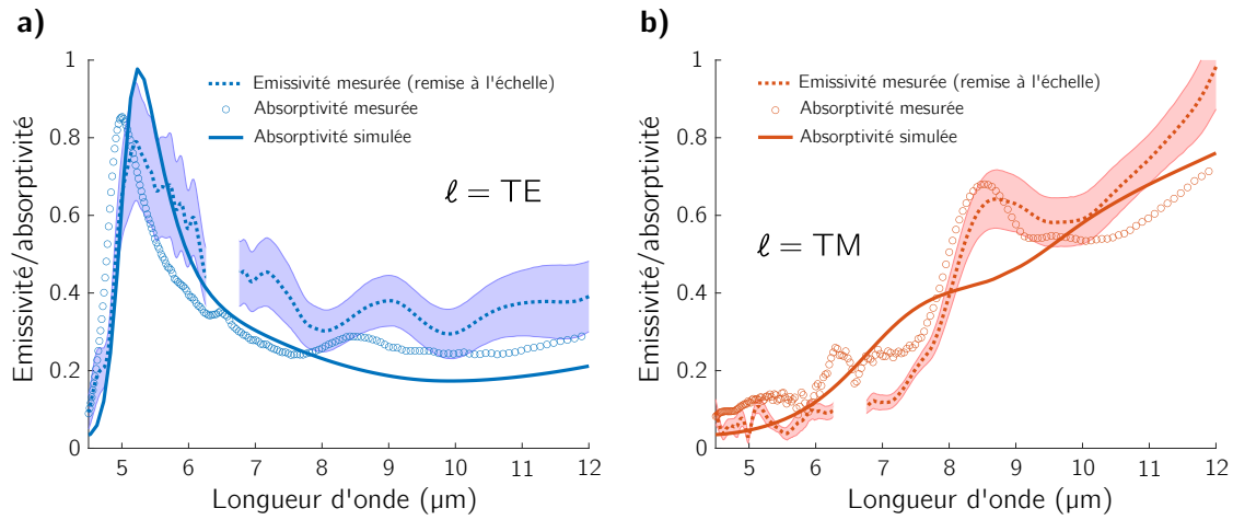
Figure 2.16 – Spectre d'émissivité/d'absorptivité de notre source en polarisation a) TE et b) TM. En traits pointillés : spectre d'émissivité remis à l'échelle de façon à avoir un maximum d'amplitude comparable au spectre d'absorption. Les barres d'erreur tracées sont à 1\sigma . La bande spectrale 6-7 \mu m affectée par le CO_2 de l'air n'est pas représentée. En rond : spectres d'absorption mesurés en réflectivité. En traits pleins : spectres d'absorption simulés numériquement.
