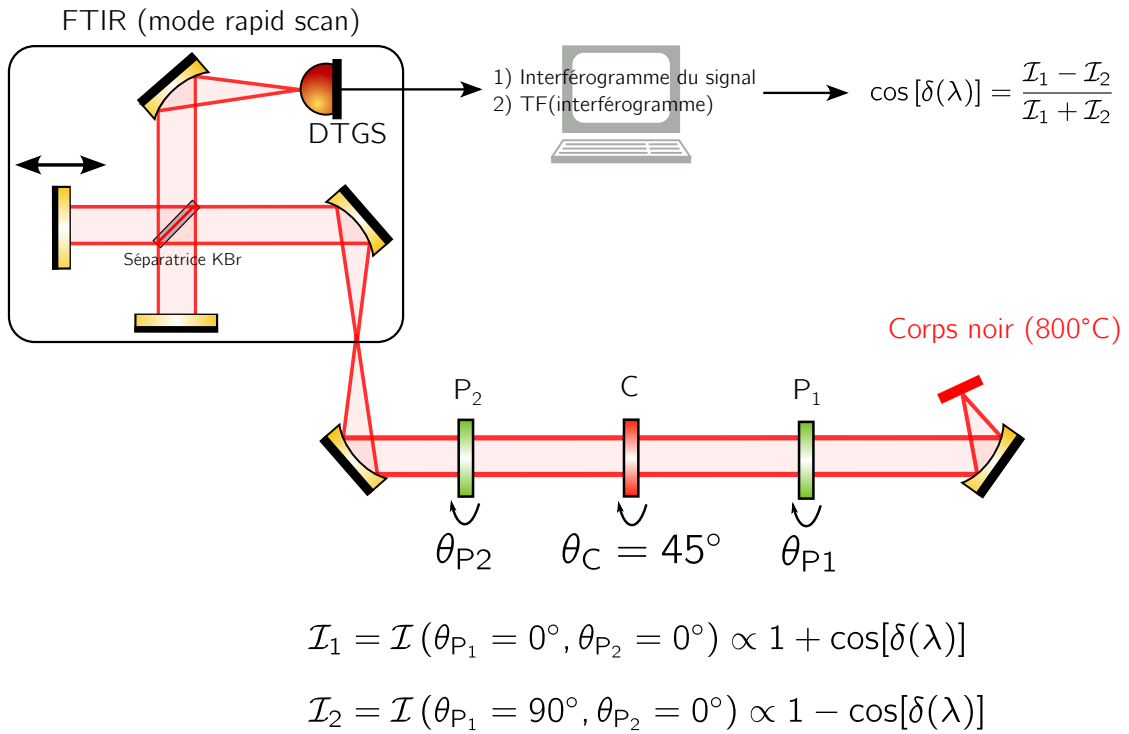
Figure 4.13 – Dispositif de mesure du retard de la lame de \text{MgF}_2 . La lame est positionnée à 45^\circ des axes des polariseurs. On mesure les intensités transmises lorsque les polariseurs sont parallèles et croisés. Celles-ci sont proportionnelles, à un facteur numérique près, au produit de la transmission à travers chacun des éléments optiques par la réponse du détecteur. Il n'est pas utile de connaître leur valeur numérique pour mesurer le retard de la lame au vu de l'Eq.(4.31)
