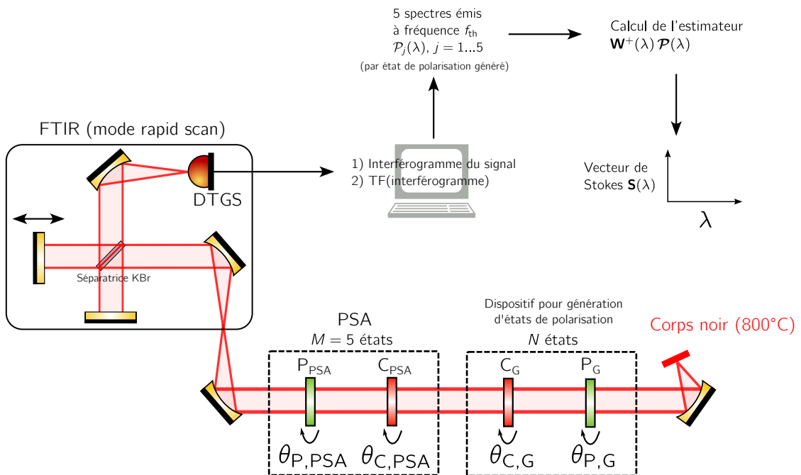
Figure 4.15 – Dispositif expérimental permettant la mesure directe des coefficients de la matrice d'analyse d'état de polarisation décrivant le PSA et permettant le test de calibration du PSA.
