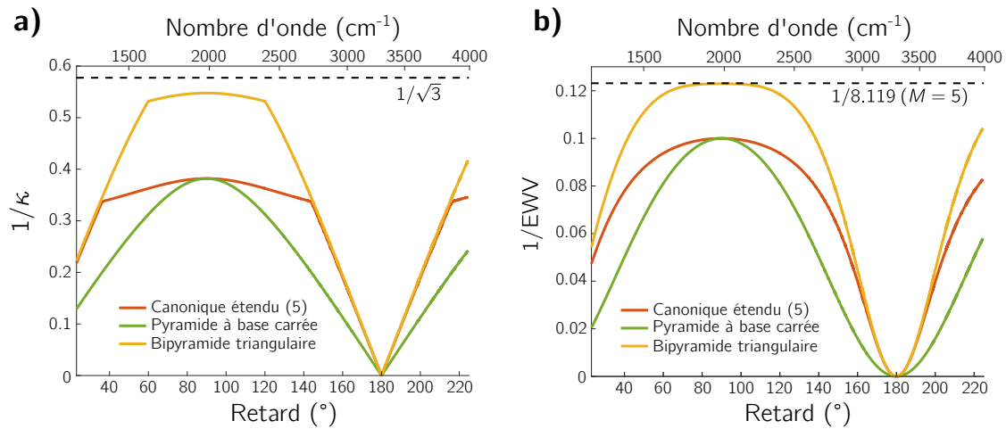
Figure 4.6 – Comparaison des figures de mérite présentées en Sec.4.1.4 et 4.1.5. a) Inverse du nombre de condition sur \mathbf{W} et b) inverse de l'EWV pour un PSA constitué d'une lame en \text{MgF}_2 , quart d'onde à 2000 \text{ cm}^{-1} , suivi d'un polariseur linéaire. Dans les deux figures, nous représentons les configurations d'un ensemble canonique étendu à 5 états (orange), d'une pyramide à base carrée fixe (5 états, vert) et d'une bipyramide triangulaire (5 états, jaune). Dans a) , la ligne en pointillés à 1/\sqrt{3} représente le nombre de condition optimal qui peut être atteint ([Tyo, 2000]). En b) , la ligne en pointillés à 1/8.119 représente l'inverse du EWV minimal atteignable pour un PSA à M = 5 états ([Foreman and Goudail, 2019]).
