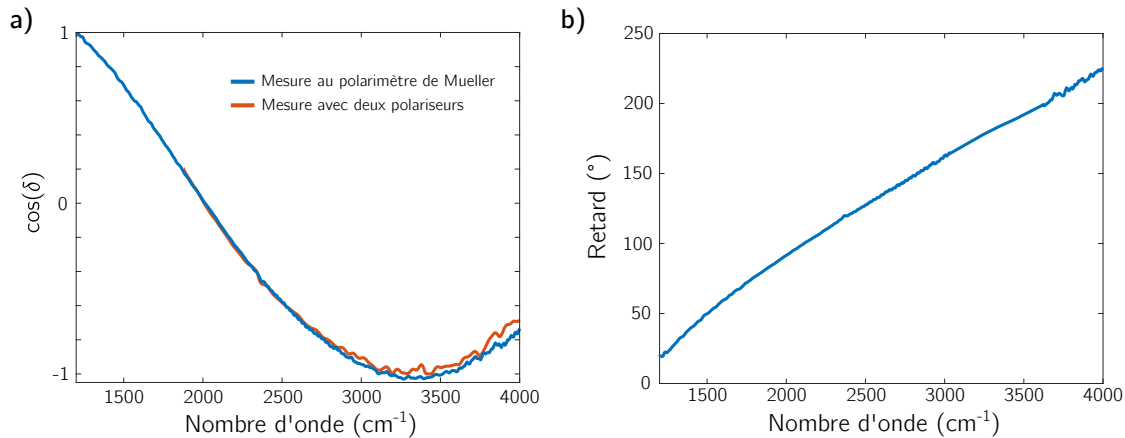
Figure 4.14 – Dispersion du retard de la lame de \text{MgF}_2 utilisée dans le PSA présenté. a) Mesure expérimentale de \cos[\delta(\lambda)] avec un polarimètre de Mueller (en bleu, reprise de la composante (4,4) de la matrice de Mueller en Fig.4.10) et par le dispositif construit en Fig.4.13 (en orange). b) Retard de la lame de \text{MgF}_2 utilisée dans le PSA, déduit de la mesure de la figure de gauche.
