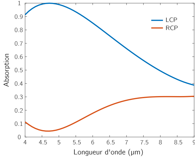
Figure 5.20 – Simulation du spectre d'absorption dans une structure en écran de Salisbury où le film métallique uniforme est remplacé par une couche homogène anisotrope.
