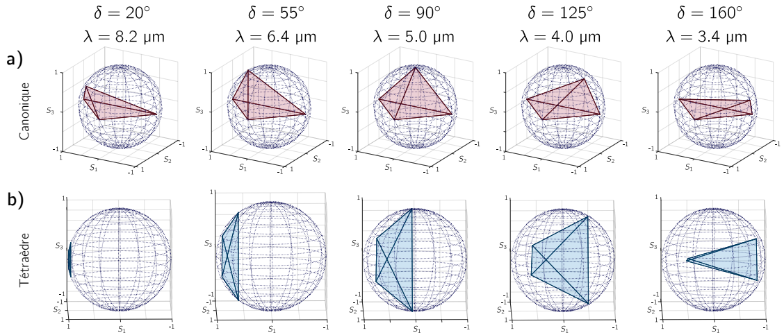
Figure 4.4 – Évolution des états du PSA sur la sphère de Poincaré en fonction du retard \delta de la lame pour les configurations a) ensemble canonique à 4 états et b) tétraèdre.
