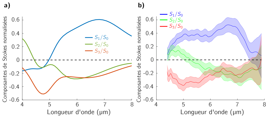
Figure 5.12 – Paramètres de Stokes normalisés par rapport à l'intensité totale a) simulé b) mesuré expérimentalement avec le PSA décrit au Chapitre 4, Sec.4.3.2. Les barres d'erreur sont à 1\sigma . La gamme spectrale entre 4 et 4.4 \mu\text{m} n'est pas représentée à cause de l'absorption du \text{CO}_2 .
