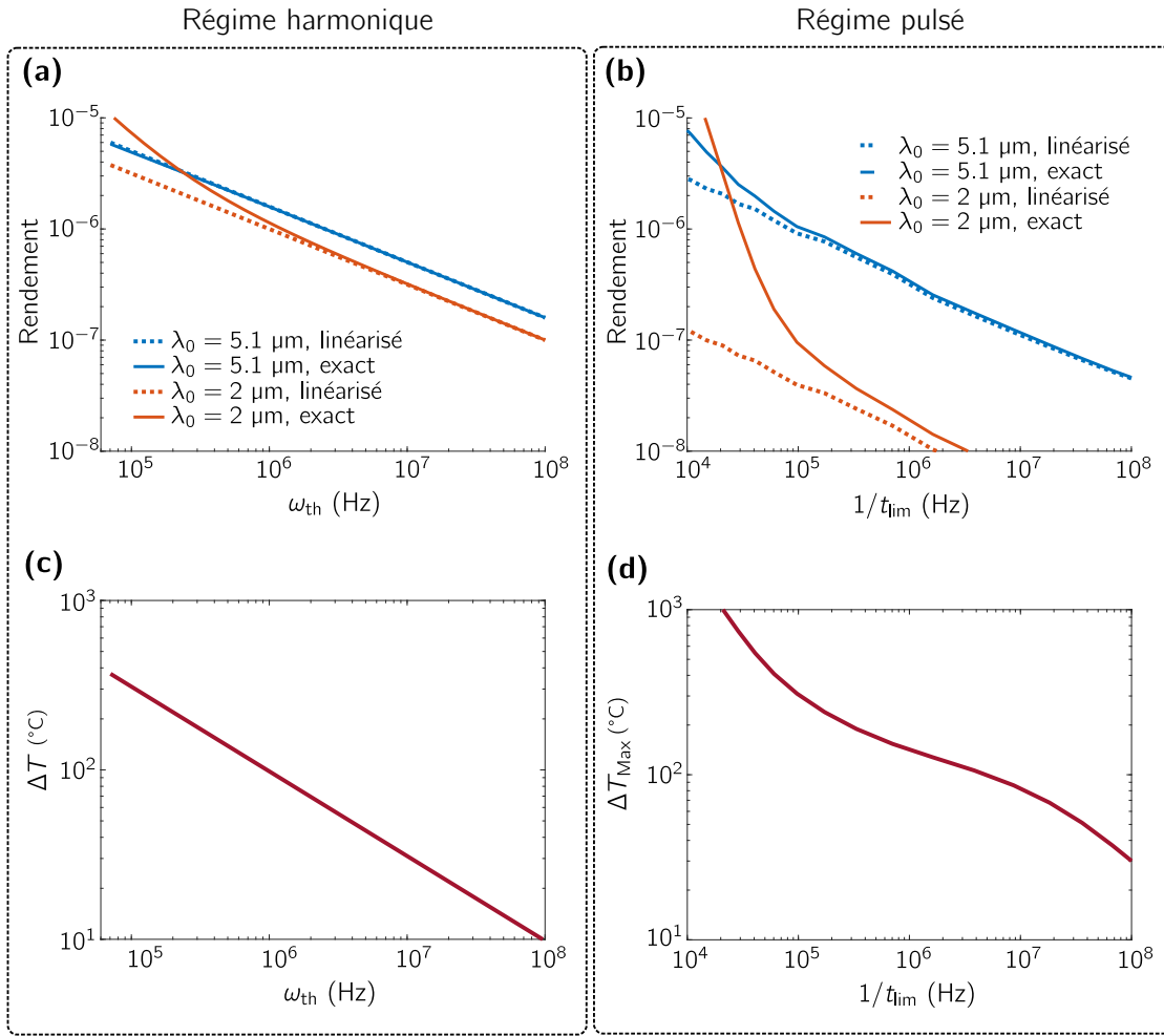
Figure 3.4 – a) : Rendement de la source en fonction de la fréquence de modulation selon les définitions données en Eq.(3.7) (exacte) et Eq.(3.22) (linéarisée) dans le cas d'une modulation harmonique à U_0 = 20 V conduisant à un échauffement tel que T_0 + T_{DC} = 724 K. b) : Rendement de la source en fonction de 1/t_{lim} selon les définitions données en Eq.(3.8) (exacte) et Eq.(3.21) (linéarisée) pour une modulation par trains d'impulsions à U_0 = 50 V et pour T_0 + T_{DC} = 500 K. c) et d) : Échauffement induits pour chacun de ces cas, pour une modulation harmonique et impulsionnelle respectivement.
