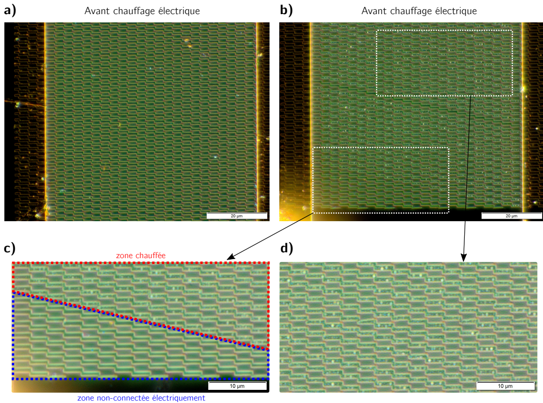
Figure 5.6 – a) Image au microscope optique en champ sombre d'un échantillon avant mise sous tension et chauffage. b) Image de la même source après utilisation. c) et d) Grossissements sur l'image b) . En c) , on distingue nettement les parties chauffées (en rouge) et non-chauffées (en bleu). Les images en champ sombre des parties chauffées en d) montrent l'apparition de bulles au niveau du platine.
