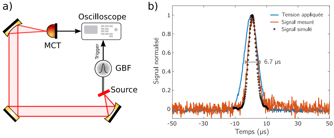
Figure 2.8 – a) Dispositif expérimental pour la mesure de la réponse de la source à un pulse de tension. b) Montage et caractérisation expérimentale de la réponse de la source présentée en Fig.2.3 à un pulse de tension gaussien. Le pulse de tension a une amplitude maximale de 5 V et une cadence de répétition de 10 kHz. Les données expérimentales ont été moyennées sur plusieurs millions de périodes.
