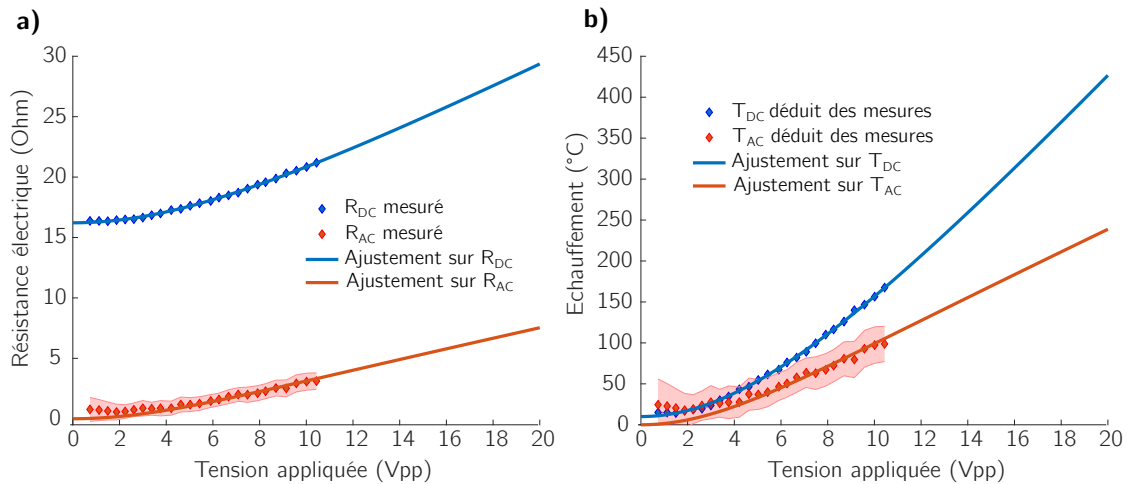
Figure 5.8 – a ) Mesure expérimentale et ajustement de l'évolution de la résistance électrique de la source en fonction de la tension du GBF. b ) Échauffement du platine déduit des mesures de résistance électrique.
