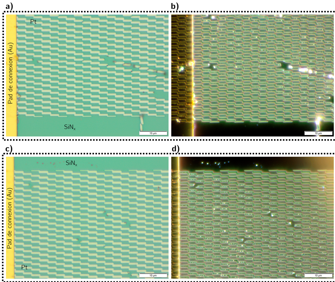
Figure 5.7 – Images au microscope optique en bright field ( a ) et c ) et dark field ( b ) et d ) de sources ayant été poussées à leur limite de fonctionnement et devenues non-fonctionnelles. a ) et b ) sont deux images d'un même échantillon ainsi que c ) et d ).
