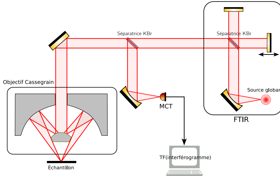
Figure 2.17 – Dispositif de mesure de réflectivité donnant accès au spectre d'absorption de la source étudiée (données expérimentales représentées en ronds transparents en Fig. 2.16).
