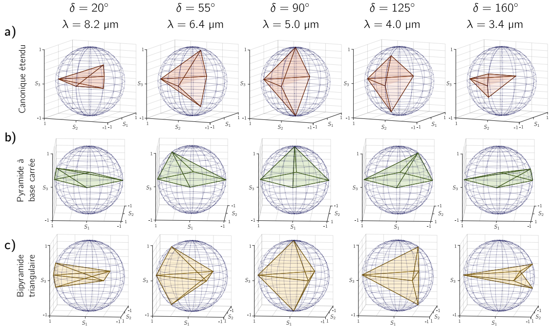
Figure 4.7 – Évolution des états de PSA à 5 états sur la sphère de Poincaré en fonction du retard de la lame pour les configurations a) ensemble canonique étendu à 5 états, b) pyramide à base carrée, c) bipyramide triangulaire.
