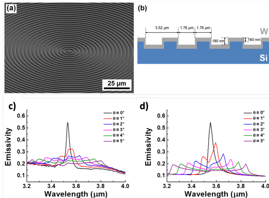
Figure 1.7 – a) Image MEB à 60^\circ de la métasurface proposée par [Park et al., 2016] en forme d'œil de boeuf constituée de 300 cercles concentriques. b) Schéma en coupe de la structure. c) Émissivité de la structure chauffée à 900^\circ\text{C} . Mesure expérimentale sous différentes incidences \theta à la normale. d) Émissivité simulée numériquement.
