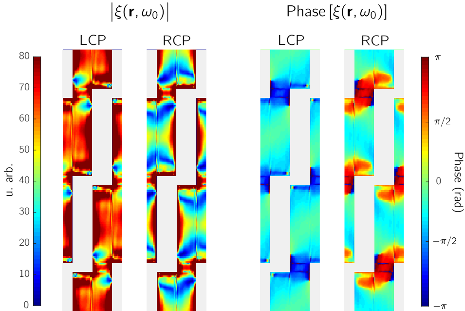
Figure C.4 – Carte de \xi (intégrande de l'Eq.(5.21)) pour le QNM1 à \omega_0 = 2\pi c/\lambda_0 , \lambda_0 = 4.7 \mu\text{m} pour les polarisations LCP et RCP. À gauche, on donne une carte de la norme de \xi , à droite, une carte de sa phase. Les zones en gris clair délimitent la structure en platine où \Delta\epsilon = 0 , conséquence du choix de la situation de référence (voir Fig.5.15).
