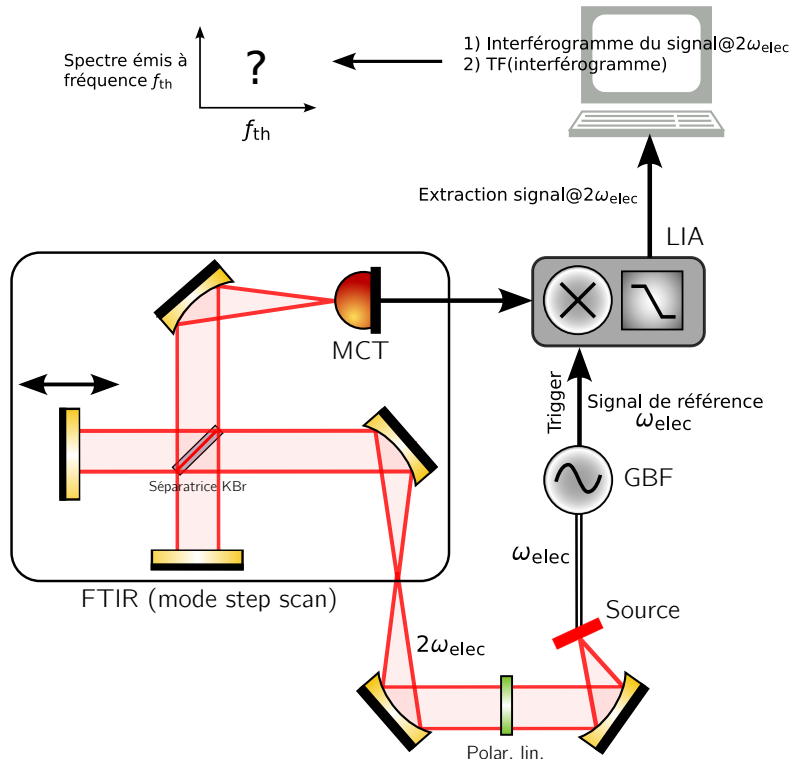
Figure 2.12 – Dispositif de mesure de la réponse en fréquence de la source.
