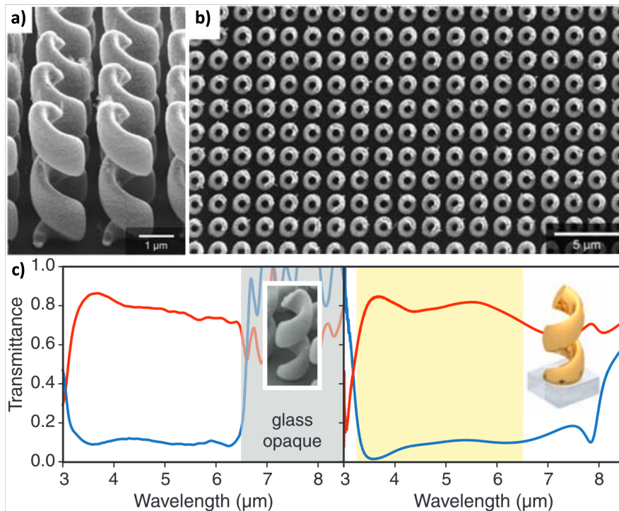
Figure 1.12 – a) Image MEB latérale des spirales d'or proposées par [Gansel et al., 2009]. b) Image MEB vue du dessus des spirales. c) Spectre de transmittance mesuré (à gauche) et simulé (à droite).
