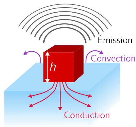
Figure 2.1 – Canaux de refroidissement d'un corps chaud posé sur un substrat froid.
