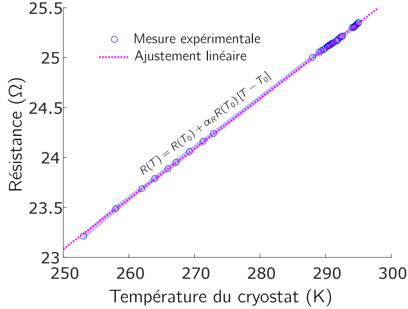
Figure 2.13 – Mesure du coefficient de température du platine \alpha_R à partir de mesure de dépendance de la résistance de notre échantillon à la température.
