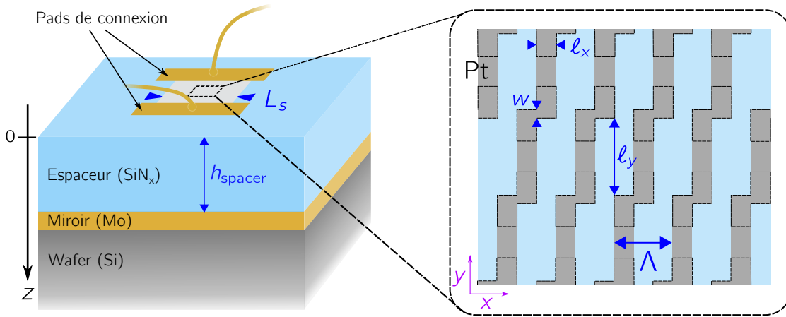
Figure 5.2 – Schéma de la source conçue pour émettre avec un fort dichroïsme circulaire. À l'issue de l'optimisation numérique sur les paramètres géométriques de la structure, nous obtenons l_x = 688 \text{ nm} , l_y = 2.737 \text{ }\mu\text{m} , w = 300 \text{ nm} , \Lambda = 2.063 \text{ }\mu\text{m} , h_{\text{spacer}} = 651 \text{ nm} , h_{\text{Pt}} = 25 \text{ nm} . Les lignes pointillées indiquées sur la structure en platine servent de support visuel pour délimiter les résonateurs en forme de Z, ils n'ont pas d'existence physique. La métasurface fait une taille de L_s \times L_s = 100 \times 100 \text{ }\mu\text{m}^2 .
