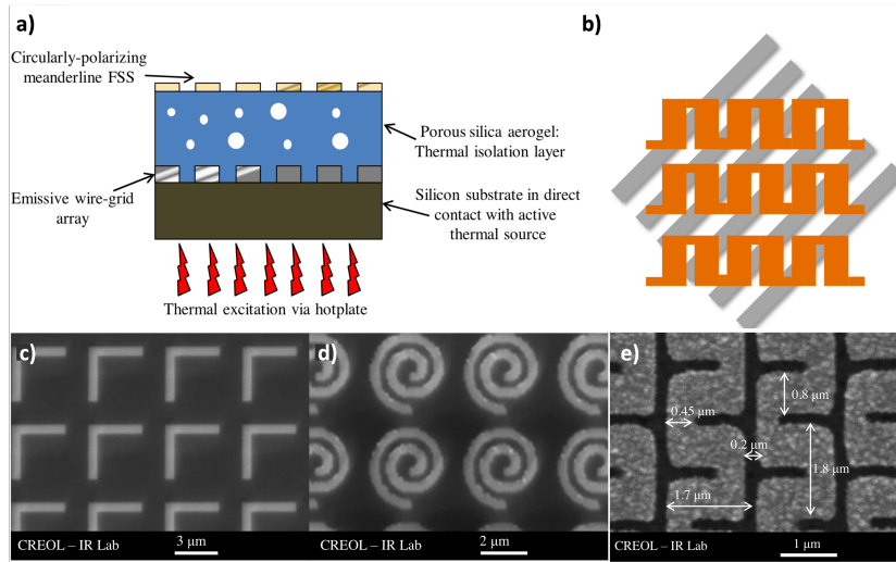
Figure 1.17 – a) Schéma en coupe de la source incandescente composite proposée par [Wadsworth et al., 2011] pour émettre du rayonnement thermique dans le MIR polarisé circulairement. b) Schéma de la source vue du dessus. La couche supérieure est une méta-surface permettant de convertir une polarisation linéaire incidente à 45^\circ en une circulaire (une quart d'onde 2D en somme). Le substrat en silicium est chauffé. Des fils métalliques sont posés en contact direct avec le chauffage et émettent un rayonnement polarisé linéairement. c-d) Structures testées alternativement aux meanderlines en forme de L ( c) ) ou de spirale ( d) ). Ces dernières ne donnent aucun dichroïsme circulaire lorsqu'elles sont chauffées seules (sans fils métalliques en-dessous). e) Image MEB des meanderlines .
