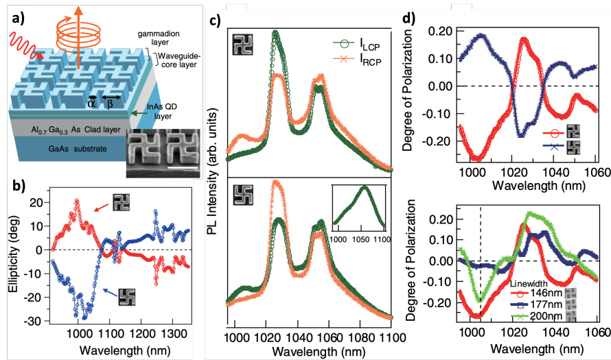
Figure 1.15 – a) Schéma de la source proposée par [Konishi et al., 2011] à base d'un cristal photonique chirale. En inset, image MEB d'un gammadion "gauche". La barre d'échelle indique 1 µm. b) Mesure du spectre d'ellipticité du rayonnement transmis selon la normale à la surface. En gris/rouge (resp. noir/bleu) les résultats obtenus pour des gammadions gauches (resp. droits). c) Spectre de photoluminescence pour des gammadions gauches (haut) et droits (bas). En vert l'émission polarisée circulaire gauche, en orange l'émission polarisée circulaire droite. En inset : spectre de photoluminescence lorsque le miroir du haut n'est pas texturé. d) (haut) Degré de polarisation pour des gammadions gauche (rouge) et droit (bleu) ayant une largeur de bras de \alpha = 146 nm. (bas) Degré de polarisation pour des gammadions gauche avec différentes largeurs de bras.
