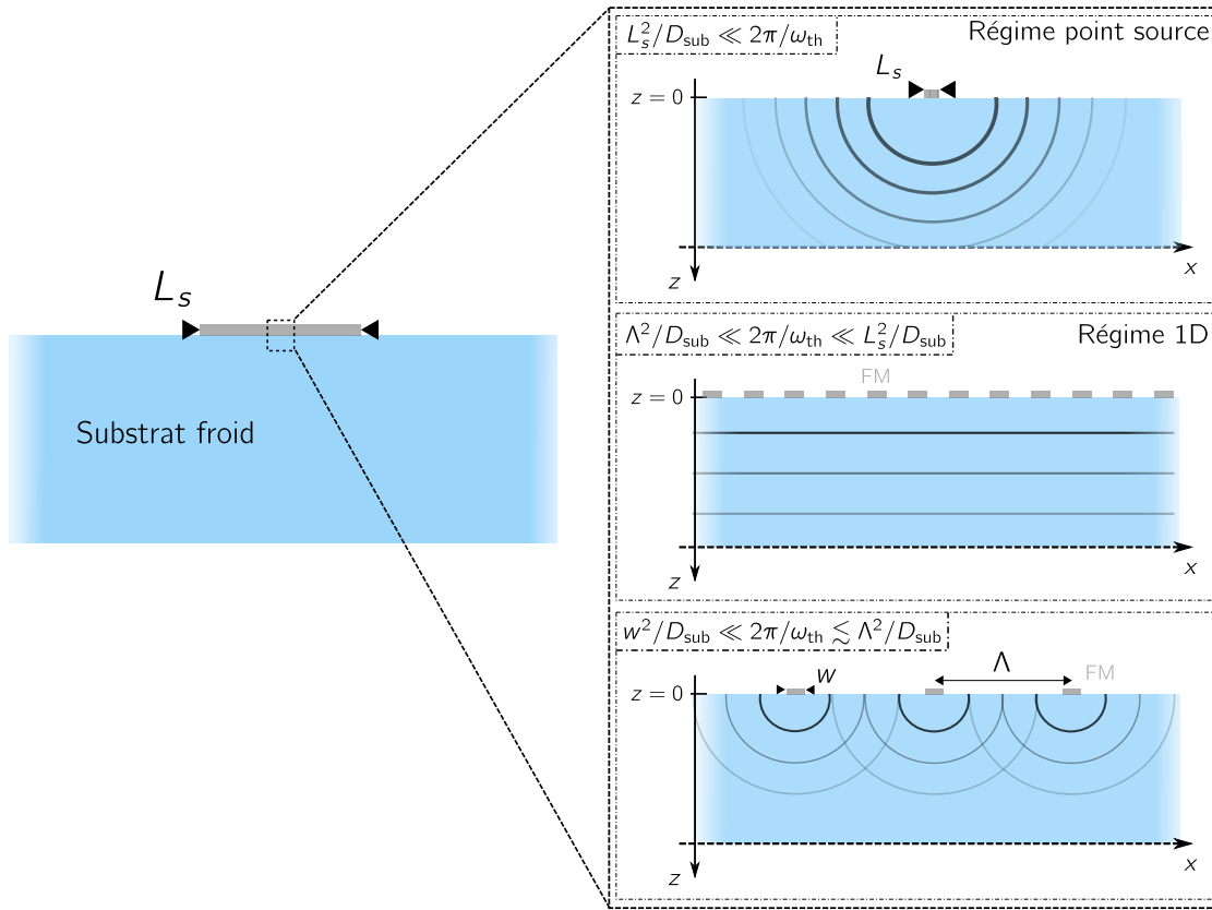
Figure 3.2 – Régimes de diffusion thermique en fonction de la fréquence de modulation de la source. Les arcs de cercles et lignes représentent les fronts d'onde thermiques.
