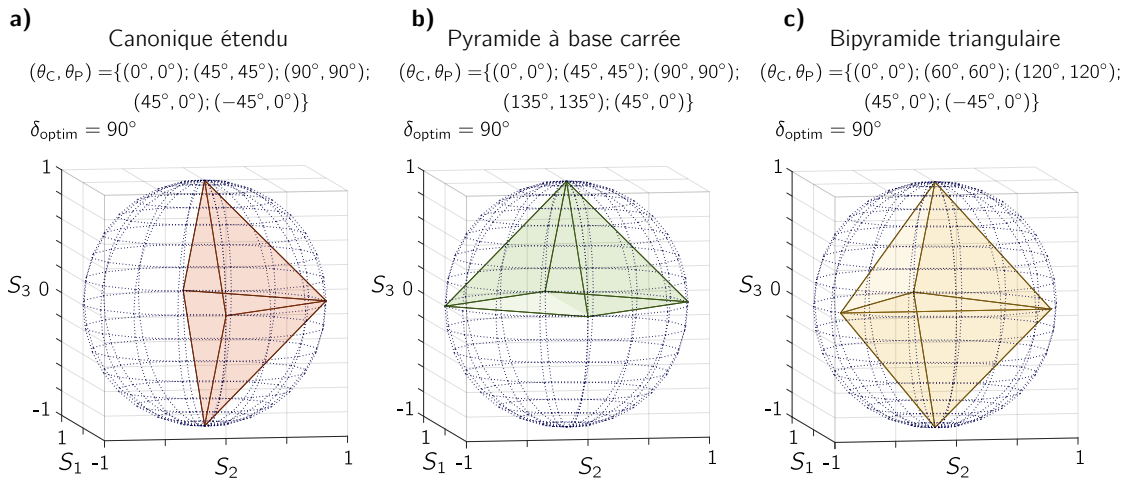
Figure 4.5 – Polyèdres inscrits dans la sphère de Poincaré représentant les différentes configurations du PSA présenté en Sec.4.2.3 pour leur retard optimal respectif : a) ensemble canonique étendu à 5 états, b) pyramide à base carrée fixe à 5 états, c) bipyramide triangulaire à 5 états.
