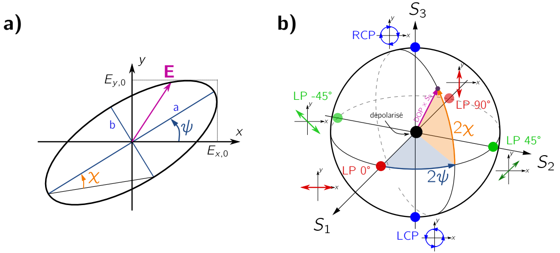
Figure 4.1 – a) Ellipse de polarisation, utilisée pour décrire l'état de polarisation d'un rayonnement complètement polarisé. b) États de polarisation canonique sur la sphère de Poincaré.
