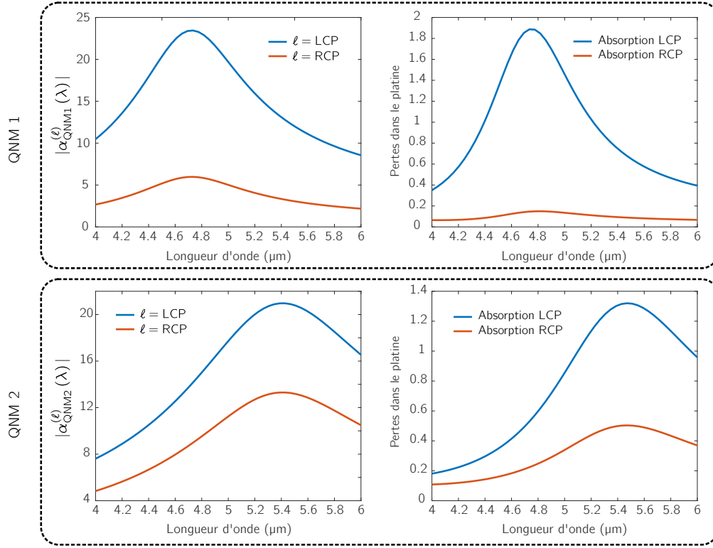
Figure C.1 – Colonne de gauche : Norme des coefficients d'excitation \alpha_X^{(\ell)}(\lambda) , X=1,2 étant le numéro du QNM identifié en Fig.5.16 et (\ell) la polarisation correspondante. Colonne de droite : Simulation du spectre d'absorption pour un unique QNM considéré. Il s'agit des QNMs contrôlant principalement la physique autour de 5 \mu\text{m} .
