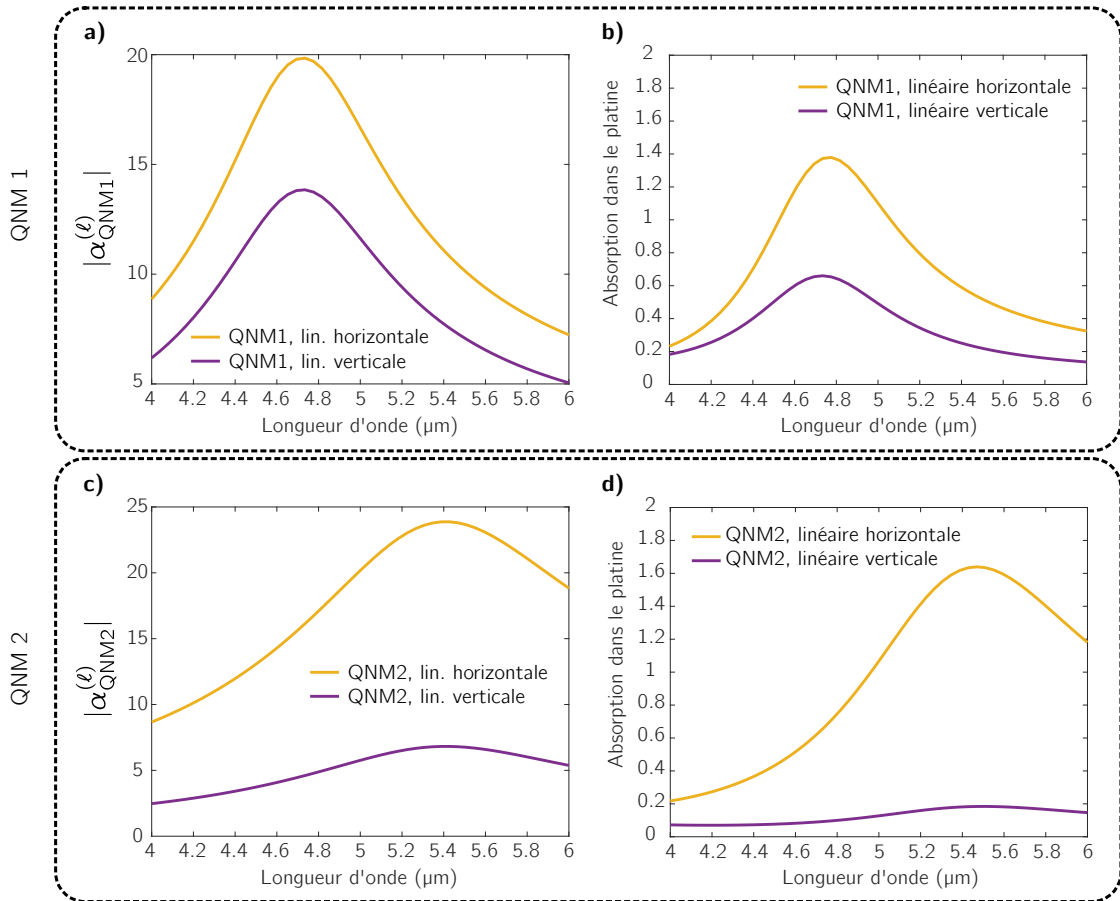
Figure 5.19 – Simulation du spectre d'absorption dans le platine lorsque l'échantillon est éclairé sous incidence normale avec une onde plane polarisée linéairement selon la direction horizontale x (convention d'orientation en Fig.5.2) et selon la direction verticale y en tronquant le champ à un seul QNM. On garde en a) uniquement le QNM1 et en b) uniquement le QNM2. L'absorption peut dépasser 1 lorsqu'on ne considère pas l'interférence de suffisamment de QNMs.
