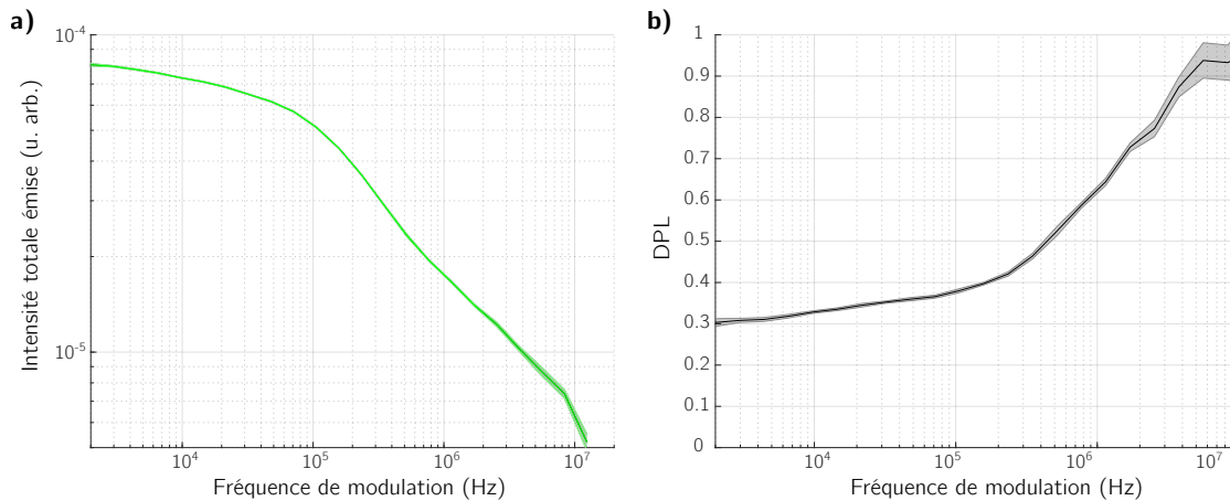
Figure 2.11 – a) Réponse de la source en fonction de la fréquence de modulation thermique f_{th} = \omega_{th}/(2\pi) = 2f_{elec} . Il s'agit de la somme des réponses de polarisations orthogonales présentées en Fig.2.10. b) Degré de polarisation linéaire (DPL) entre polarisations croisées verticale (TE) et horizontale (TM) normalisé par rapport à l'intensité totale.
