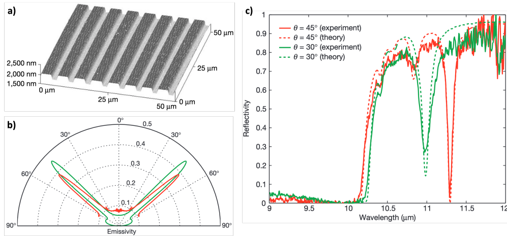
Figure 1.3 – a) Profil de la source incandescente en réseau 1D de SiC proposée par [Greffet et al., 2002] mesuré à l'AFM. b) Simulation (en vert) et mesure expérimentale (en rouge) de la directivité de l'émissivité de la source à 11.36 \mu\text{m} . c) Spectre de réflectivité simulée (pointillés) et mesurée (traits pleins) sous différentes incidences. La transmission à travers l'échantillon étant nulle dans ce domaine spectral, ces courbes donnent le spectre d'émissivité via 1 - R ce qui montre un pic très fin vers 11 \mu\text{m} avec une valeur maximale proche de 0.85 à 11.36 \mu\text{m} sous 45^\circ .
