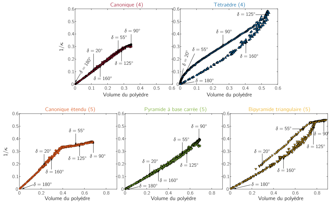
Figure 4.8 – Tracé de l'évolution de l'inverse du nombre de condition de la matrice d'analyse d'état de polarisation pour 5 configurations (4 états : canonique, tétraèdre. 5 états : canonique étendu, pyramide à base carrée, bipyramide triangulaire) en fonction du volume du polyèdre représentant cette même configuration. On observe une corrélation entre volume occupé par le polyèdre et le nombre de condition sans qu'une loi évidente puisse être trouvée. On peut noter que plus le volume est faible, plus le conditionnement est mauvais, ce qui suffit pour l'étude présentée.
