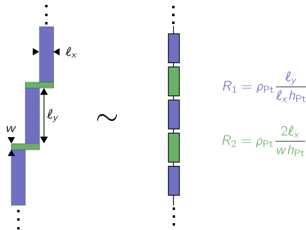
Figure 5.4 – Estimation grossière de la résistance électrique de la source.
