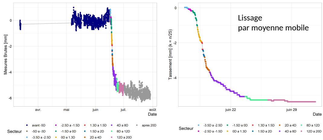
Figure 5.10. Exemples de résultats du lissage des mesures par moyenne mobile, avec largeur de la fenêtre k = n/25 où n est le nombre de mesures
