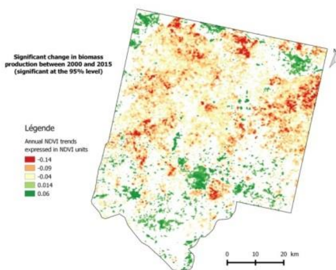
Figure 64: Tendances de NDVI entre 2000 et 2015 dans la zone d'étude (Leroux et al., 2016).
