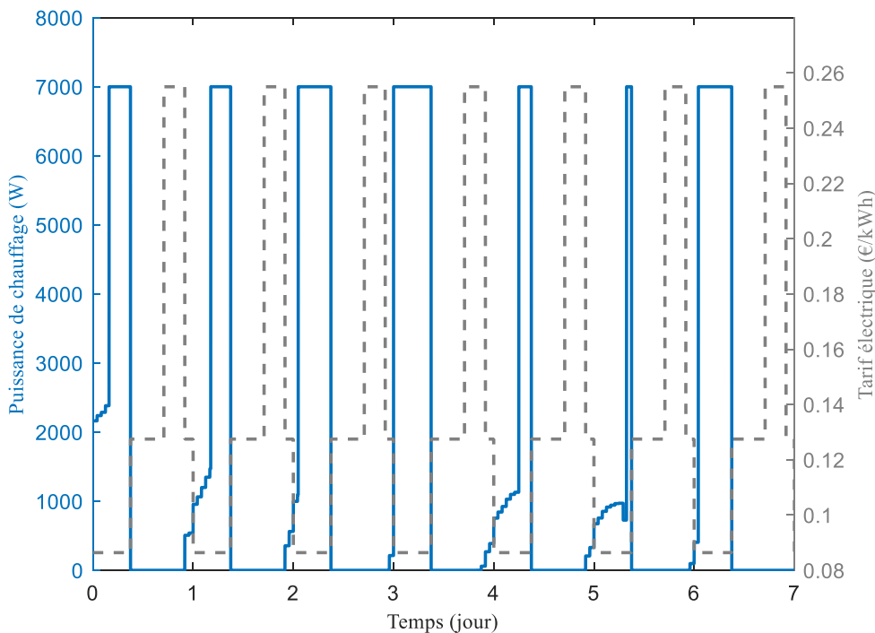
Figure 3.10 : Commande optimale de chauffage pendant la 1 ère semaine de chauffe
