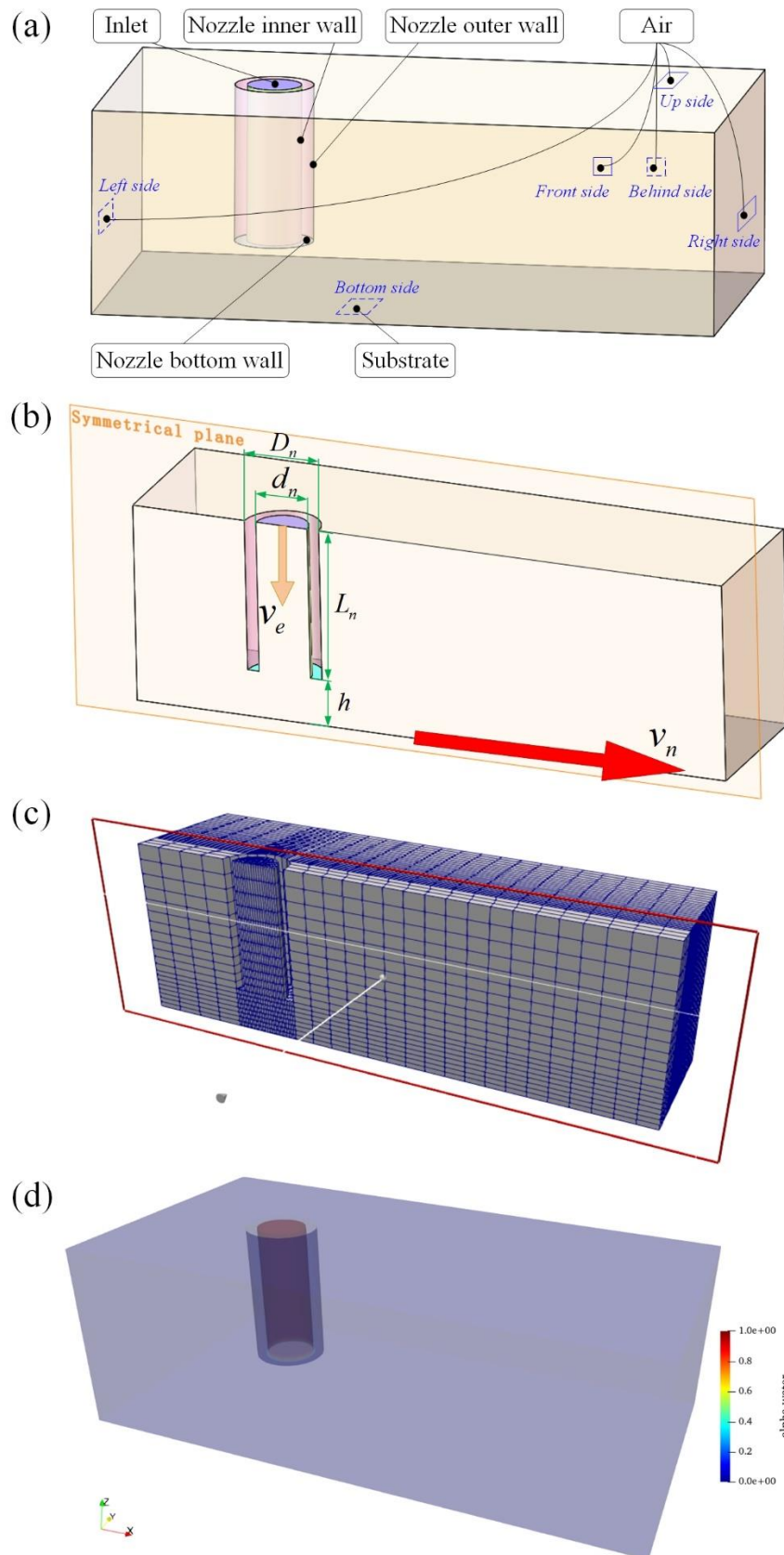
Figure 4.7 Mod éisation num érique du profil 3D du DF : (a) mod èle g éom étrique 3D ; (b) les param ètres critiques du mod èle ; (c) maillages g én ér és ; (d) condition initiale de la fraction de phase
