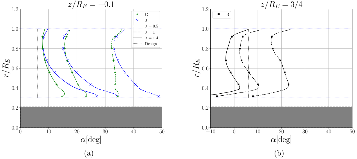
FIGURE 3.17 – Profils radiaux moyens d’angle d’attaque. Les angles ont été calculés pour les rotors de Glauert et Joukowsky en z/R_E = -0.1 (a), tandis que pour le rotor de Betz, les angles ont été calculés à partir du profil radial d’induction axiale en z/R_E = 0.8 et en considérant a' = 0 (b).
