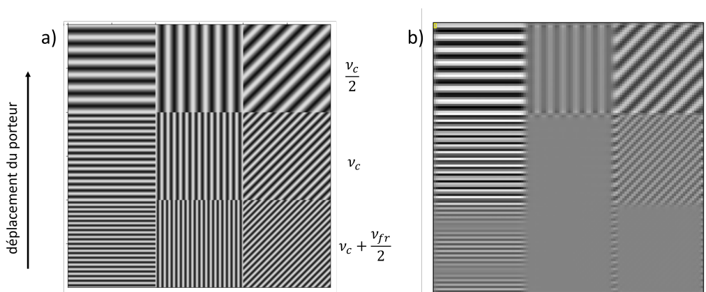
FIGURE 3.7 – a) Mire sinusoïdale en entrée b) Image monochromatique à \sigma_e , qui montre la transmission privilégiée des fréquences spatiales orientées dans la direction du déplacement.
