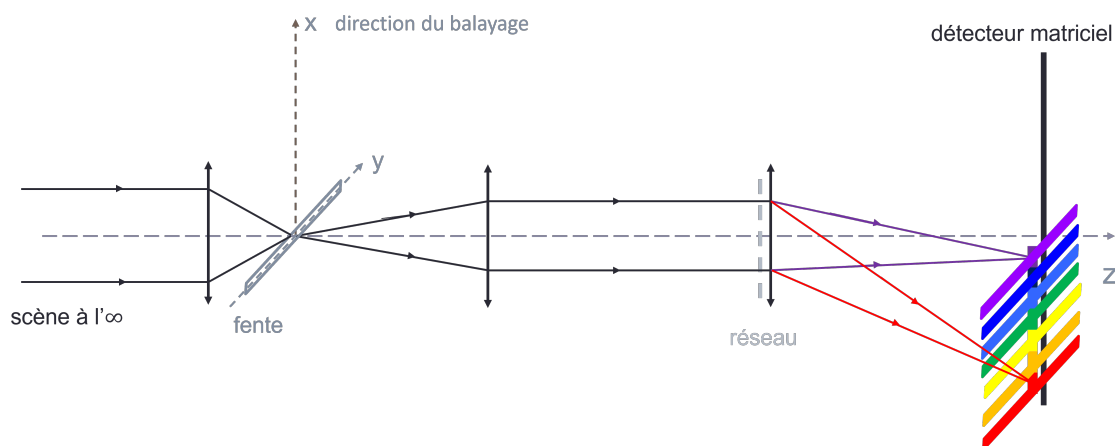
FIGURE 1.3 – Fonctionnement d'un spectro-imageur à réseau en mode pushbroom . La lumière provenant de la scène est focalisée sur la fente d'entrée avant d'être collimatée puis dispersée par le réseau et conjuguée sur le détecteur.
