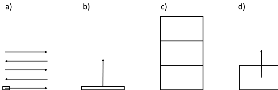
FIGURE 1.2 – Différents modes d’acquisition selon la classification de Sellar et Boreman : a) whiskbroom : l’instrument ne voit qu’un pixel à la fois b) pushbroom : l’instrument voit une ligne et le balayage se fait dans la direction perpendiculaire à cette ligne c) framing : l’instrument fait l’image d’un champ rectangulaire, puis se déplace à la position suivante d) windowing : l’instrument voit un champ rectangulaire qui se déplace continûment.
