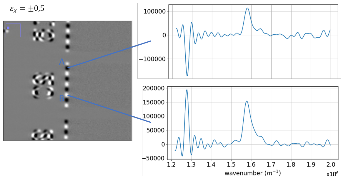
FIGURE 4.11 – Spectres aux positions A(133, 218) et B(133, 248) avec une perturbation \varepsilon_x = 0,5 pixel, K = 6 . Le pic à 1,28 \cdot 10^6 \text{ m}^{-1} est le pic parasite, tandis que le pic à 1,58 \cdot 10^6 \text{ m}^{-1} est le pic nominal.
