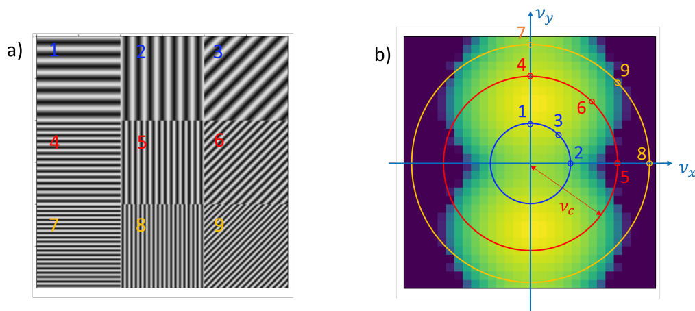
FIGURE 3.6 – a) Mire sinusoïdale monochromatique b) Fréquences présentes sur la mire représentées dans l'espace des fréquences spatiales. Le déplacement se fait dans la direction \vec{y} (direction verticale sur les images).
