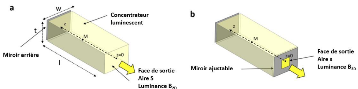
Figure II.17 –Concept d'amélioration de la luminance en sortie d'un concentrateur luminescent grâce à un confinement « 3D ». a) Concentrateur luminescent « 2D » avec un miroir haute réflexion sur la face arrière. b) Concentrateur luminescent « 3D », ajout partiel de miroir sur la face de sortie pour réduire la surface de sortie à s . [Pichon 21]
