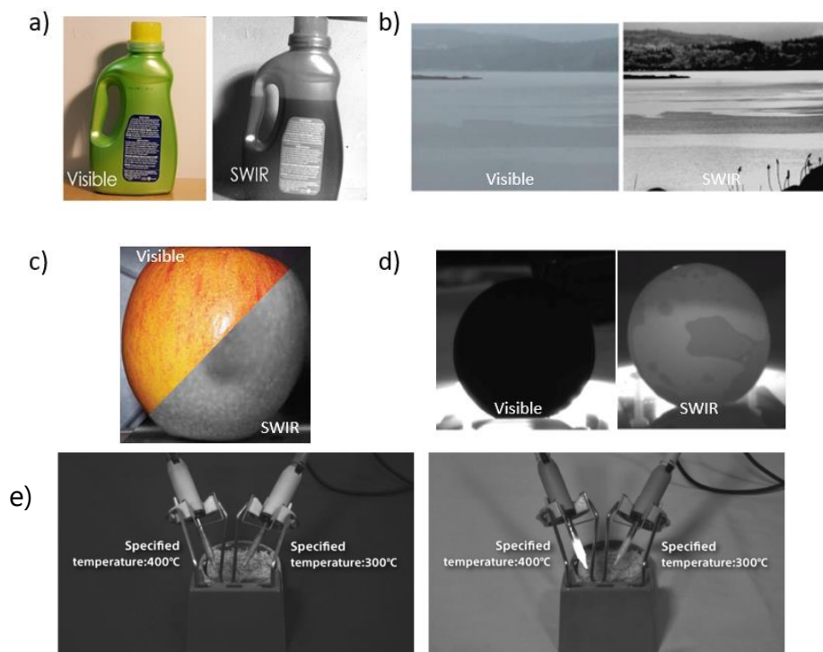
Figure In.1 – Exemple d'applications de l'imagerie dans le SWIR comparée à l'imagerie visible dans le cas : a) de contrôle qualité pour voir à travers du plastique opaque (@optics.org). b) d'imagerie par temps pluvieux (@A.Rogalski 2021). c) d'une pomme abimée(@SWIRIS). d)
