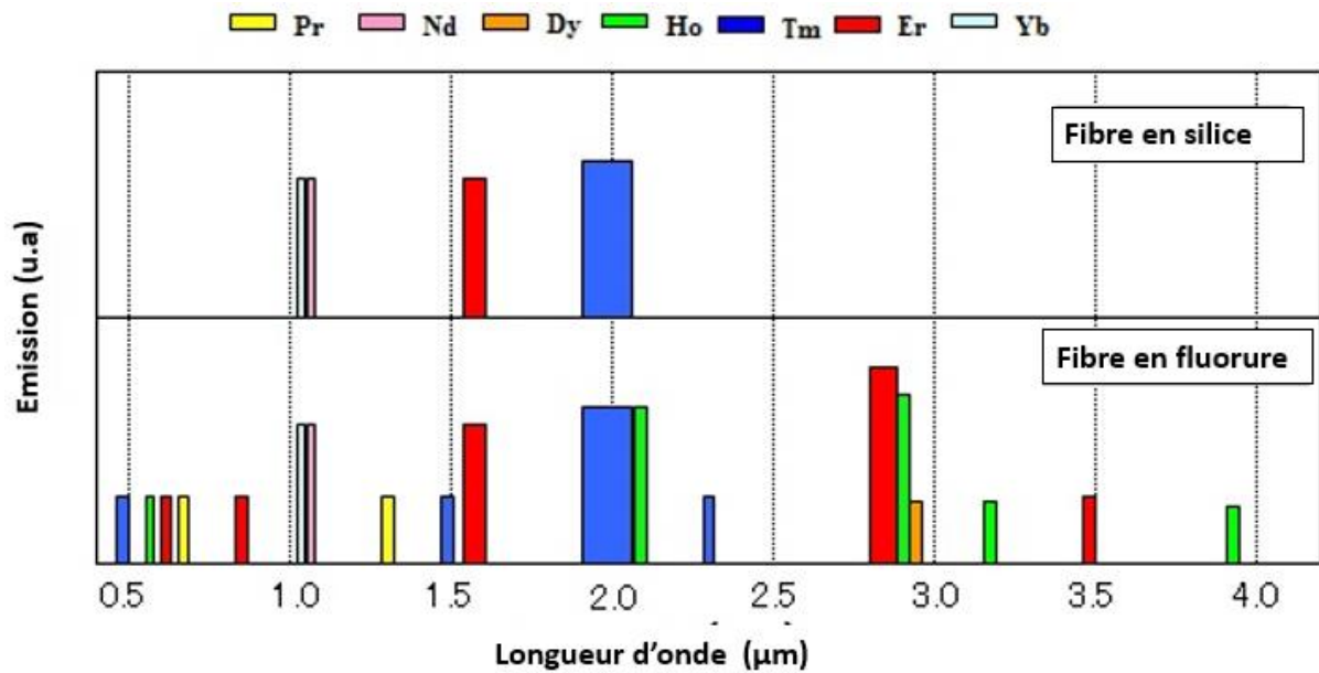
Figure 1.8 – Longueur d’onde d’émission spontanée amplifié selon le dopant et le matériau de la fibre. [FiberLabs 21].
