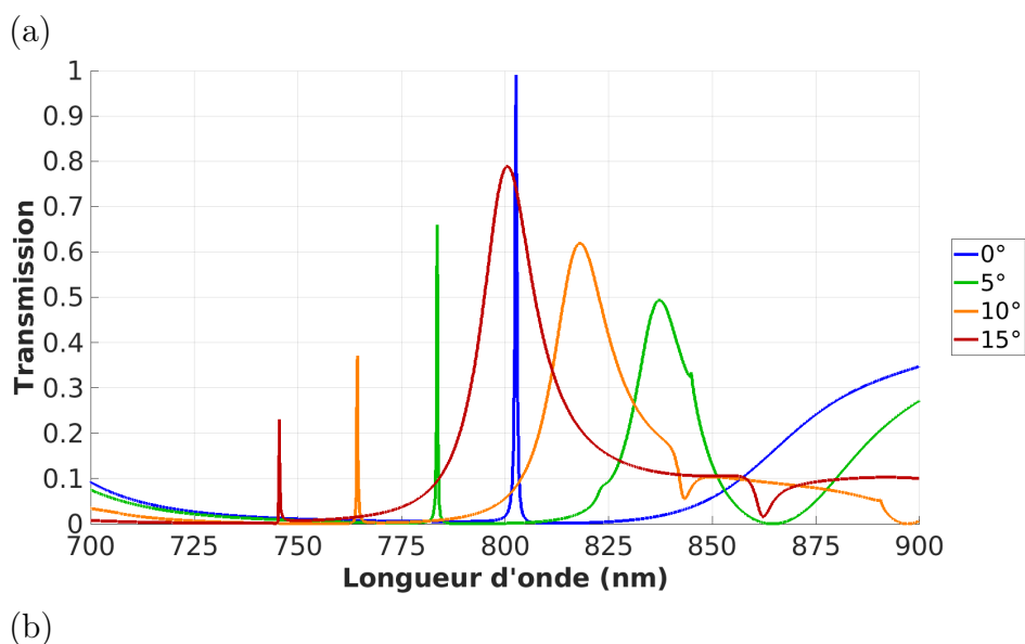
FIGURE IV.10 – Spectres en transmission d'un ZCG 1D pour voir l'impact de certaines variations de géométrie ou d'angle incident. Les courbes sont obtenues par simulation. (a) Variations de la période \Lambda (haut) et du facteur de remplissage f (bas). On voit une augmentation de \lambda_R avec \Lambda comme dans un RWG classique, mais la forme de la résonance et la transmission de fond s'en trouvent grandement modifiées, notamment lorsqu'il s'agit de faire varier f . (b) Variations de l'angle d'incidence \theta . Dès que \theta \neq 0^\circ plusieurs pics de résonance apparaissent, dont deux autour de la résonance de l'incidence normale. Mais contrairement au RWG classique, ces deux pics ne se déploient pas symétriquement, ils semblent conserver la distance qui les sépare tout en se décalant vers ses longueurs d'ondes plus faibles.
