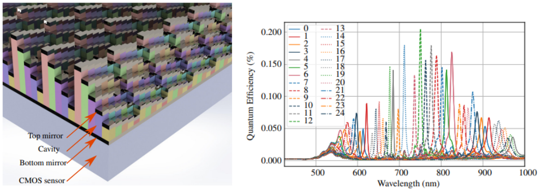
(a) Schéma de la matrice des 25 cavités Fabry-Perot du capteur hyperspectral de l'IMEC.
