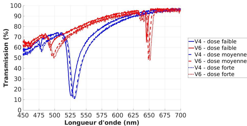
FIGURE III.24 – Spectres en transmission de deux filtres ciblant le VIS, ayant subi chacun trois conditions d'exposition différentes, dont on a mesuré les diamètres après gravure. h_R = 30 nm et h_S = 55 nm. Dimensions du filtre V4 : \Lambda = 303 nm et D_C = 152 nm, avec un diamètre réel qui prend les valeurs suivantes : D_{faible} = 160 nm, D_{moyen} = 179 nm et D_{fort} = 189 nm. Dimensions du filtre V6 : \Lambda = 418 nm et D_C = 108 nm, avec un diamètre réel qui prend les valeurs suivantes : D_{faible} = 108 nm, D_{moyen} = 126 nm et D_{fort} = 135 nm. Ils correspondent à une zone de la courbe III.12 où les CD restent assez proches de la valeur attendue.
