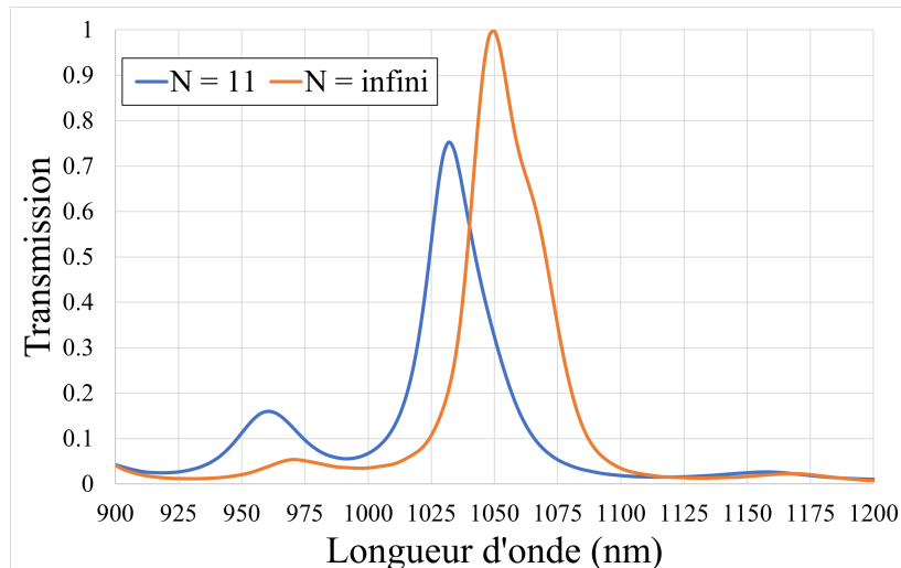
FIGURE IV.19 – Exemple de spectres de h-FPC avec un nombre fini assez faible de périodes N = 11 . Ici, \Lambda = 160 \text{ nm} , donc le réseau a une taille latérale de 1,76 \mu\text{m} .
