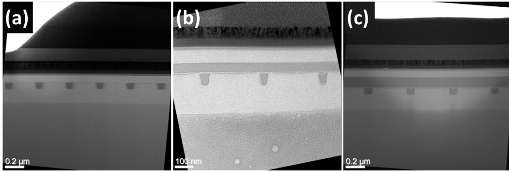
FIGURE III.8 – Coupes TEM de trois RWGs du Mask1 en SiN. (a) h_S = 0 \text{ nm} , \Lambda = 320 \text{ nm} et D_{\text{consigne}} = 220 \text{ nm} ; (b) h_S = 55 \text{ nm} , \Lambda = 320 \text{ nm} et D_{\text{consigne}} = 240 \text{ nm} ; (c) h_S = 100 \text{ nm} , \Lambda = 440 \text{ nm} et D_{\text{consigne}} = 320 \text{ nm} . On aperçoit sur la fig. (a) des résidus après gravure, probablement du SiN, formant une fine ligne sur le réseau.
