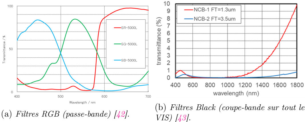
FIGURE I.13 – Transmissions de filtres en résine de chez Fujifilm (Color Mosaic) ayant des fonctions spectrales dans le VIS.
