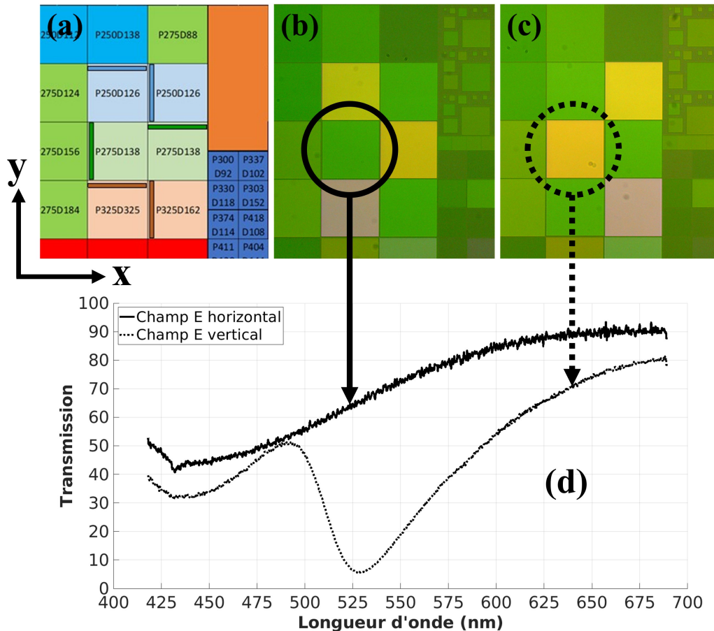
FIGURE IV.3 – Effets de la polarisation sur la résonance d'un réseau 1D. Les RWGs ont un socle en SiN d'épaisseur h_S = 55 nm et un réseau en aSi de hauteur h_R = 30 nm. (a) Schéma du design de la matrice de réseaux, avec les indications de période P et de diamètre D . Les réseaux 1D sont identifiés par un long rectangle représentant un créneau, qui donne l'orientation du réseau. (b - c) Photographies des RWGs prises en réflexion (i.e. vue du dessus, sous illumination du dessus) pour deux polarisations orthogonales de la source. (d) Spectres en transmission des filtres entourés en fonction de la polarisation de la source.
