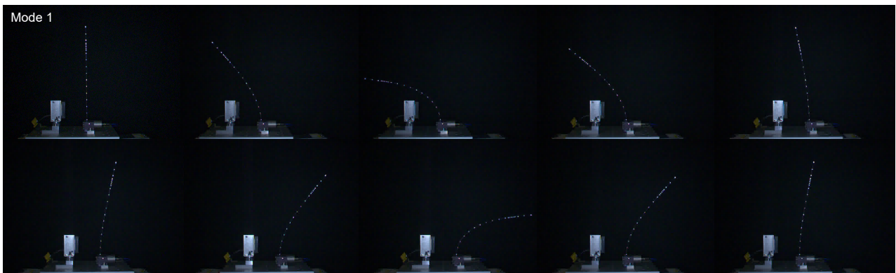
Figure E.16: Mouvement de la poutre encastrée-libre excité par accélération de la base sur son premier mode non linéaire sur \simeq 1 période.
