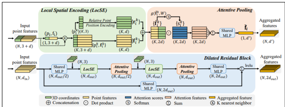
Figure 5.1 Schéma de la proposition RandLA-Net Tirée de Hu et al. (2019)
