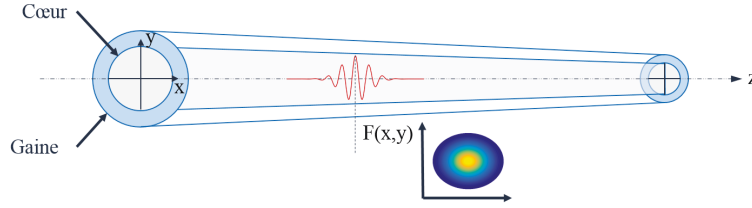
FIGURE I.2 – Propagation d'une impulsion courte dans une fibre optique monomode à saut d'indice présentant un diamètre de cœur de 2a .
