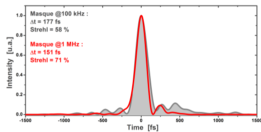
(c) Compression de l'impulsion à 500 kHz avec le masque optimisé à 100 kHz (courbe grise) et à 1 Mhz (courbe rouge).
