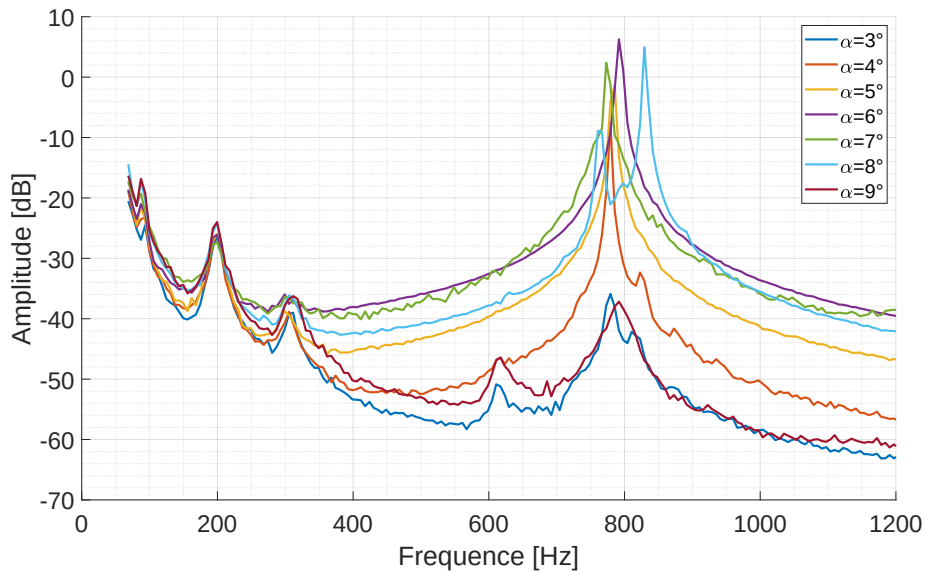
FIGURE 3.5 – Spectre vibratoire pour des incidences allant de 3 à 9^\circ , Cas I, Re = 8 \times 10^5
