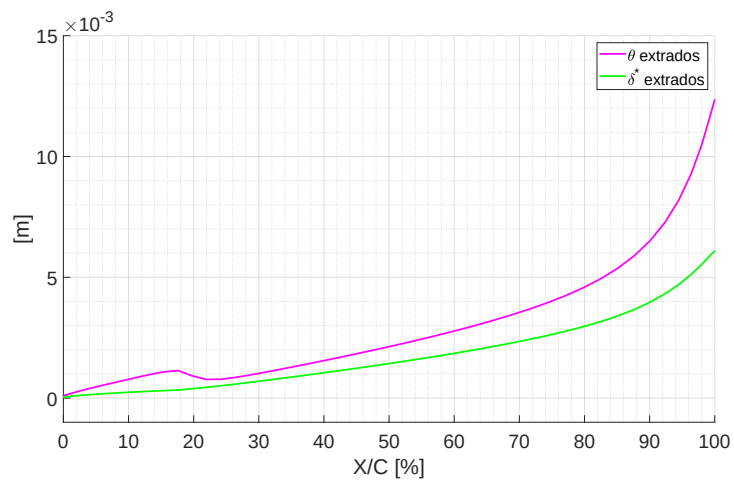
FIGURE 2.27 – Épaisseur de déplacement et de quantité de mouvement sur un NACA0015 à 6^\circ d'incidence et à Re=8 \times 10^5
