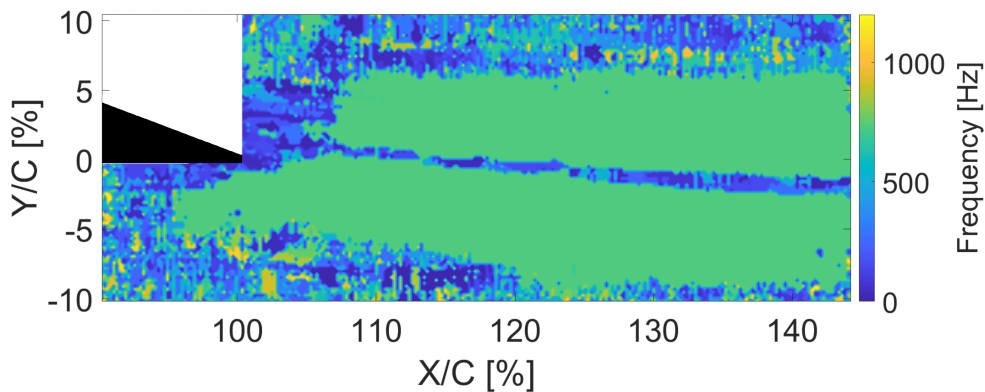
FIGURE 3.38 – Cartographie fréquentielle du sillage proche pour Re = 8 \times 10^5 et \alpha=8^\circ Cas I
