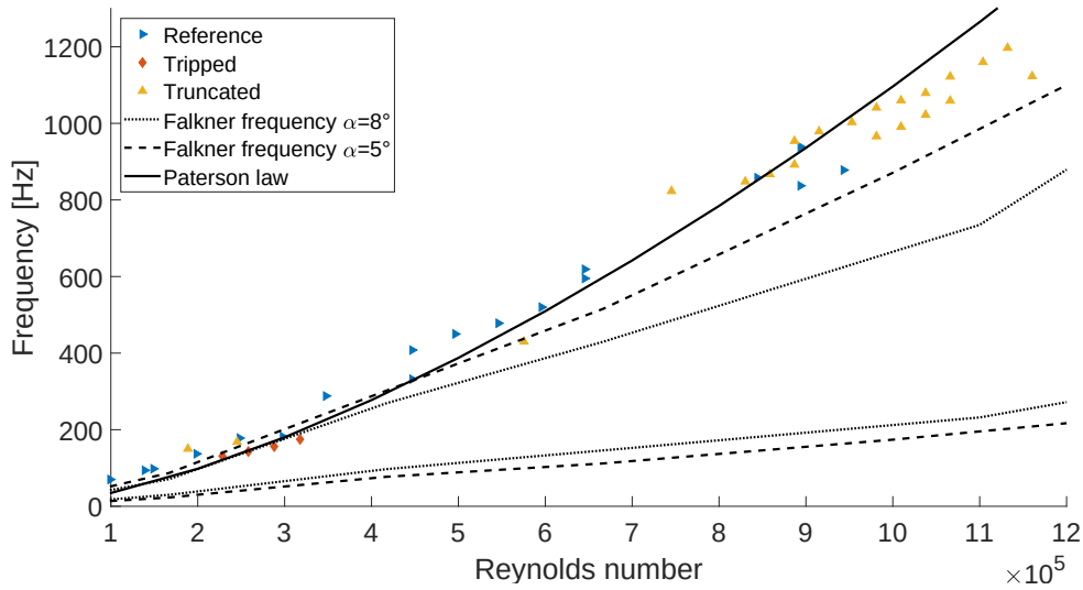
FIGURE 4.1 – Comparaison entre les fréquences expérimentales mesurées et les courbes de stabilité de OBRMSKI et al. (1969)
