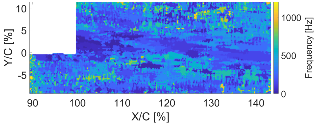
FIGURE D.7 – Variations fréquentielles d’amplitudes maximales pour Re = 8 \times 10^5 et AoA=9^\circ Cas I
