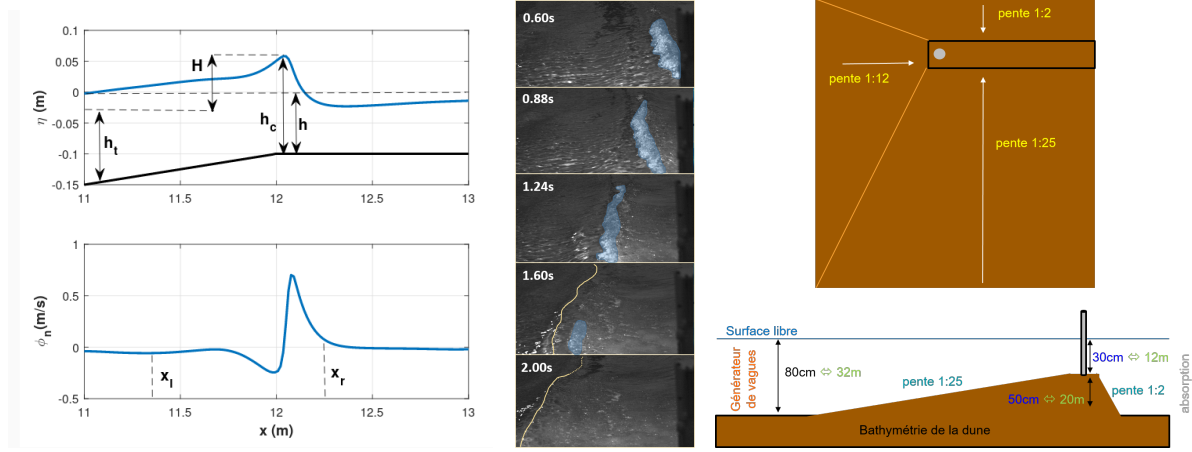
FIGURE 1 – Schéma 2D des paramètres d’une vague déferlante [3] (gauche) ; timestack des images d’une vague déferlante avec l’identification de la mousse générée (zones bleues) et d’une deuxième crête de vague (ligne jaune) avant déferlement (centre) ; et schéma 3D de la dune et de la position de la structure sur la dune (droite).
