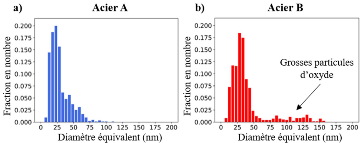
Figure II.7 : Distribution des diamètres équivalents de cercles des populations d'oxydes nanométriques présentes dans les aciers a) A et b) B (cf. Annexe I).
