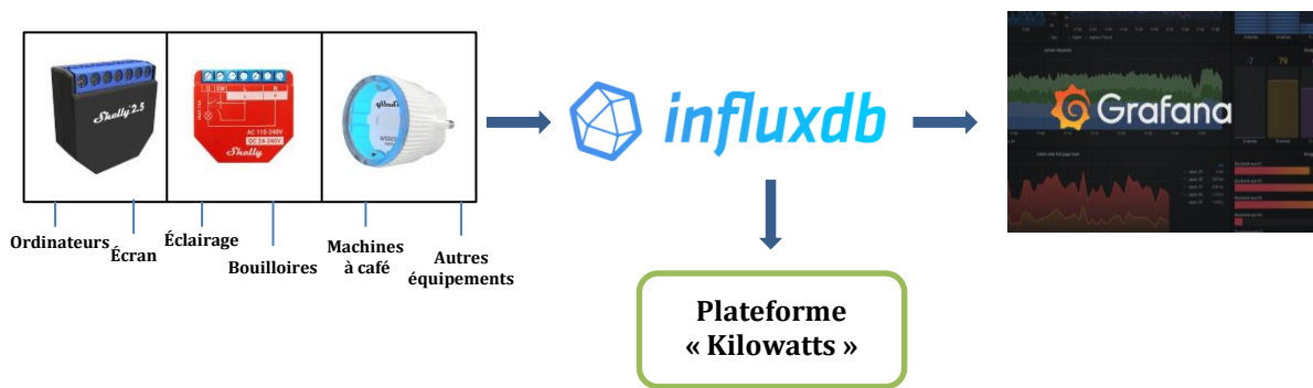
Figure 26: Processus d'acquisition des données par capteurs connectés
